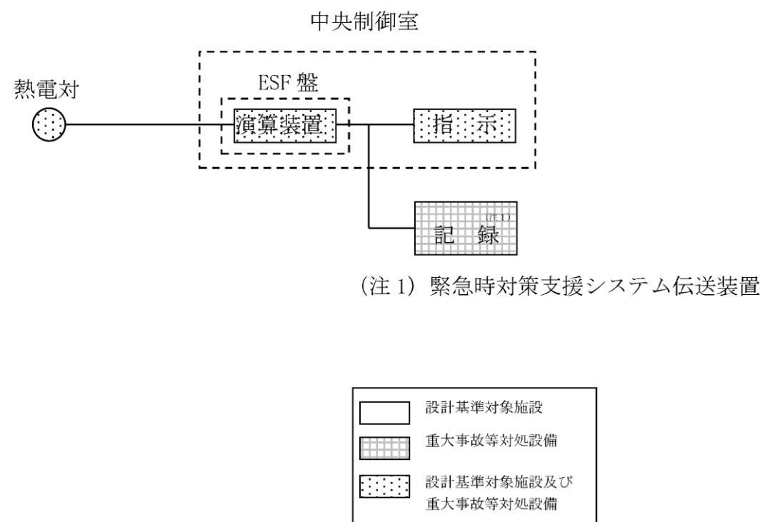
図 58-6-8 7号炉残留熱除去系熱交換器出口温度の概略構成図
