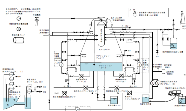
第 2.1-1 図 高圧・低圧注水機能喪失時の重大事故等対策の概略系統図 (2/3) (低圧代替注水系(常設)による原子炉注水及び代替格納容器スプレー冷却系(常設)による格納容器冷却段階)
