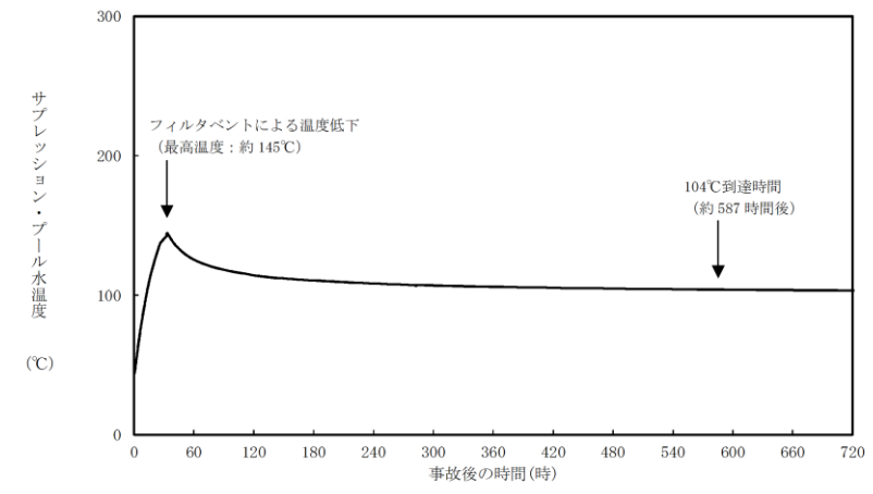
図 1.6 サプレッション・プール水温度 (格納容器過圧・過温破損) (残留熱代替除去系を使用しない場合)
