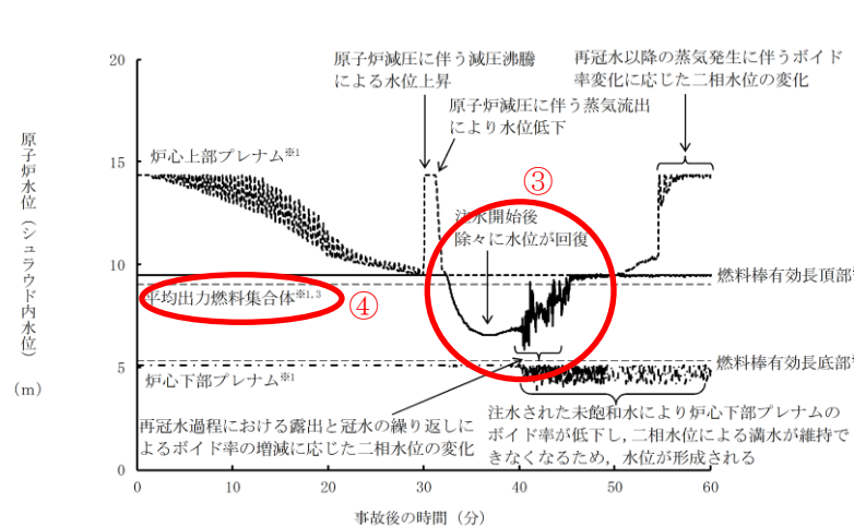
第 2.1.2-1(2) 図 原子炉水位 (シュラウド内水位) の推移※2
