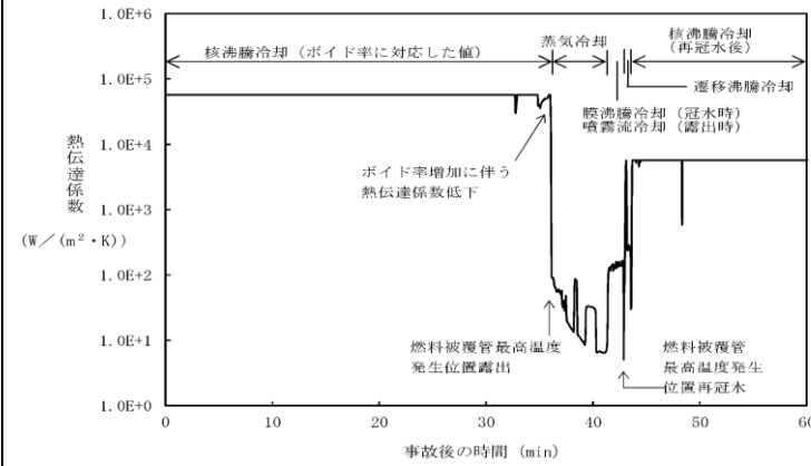
第2.2-11 図 燃料被覆管の最高温度発生位置における熱伝達係数の推移
