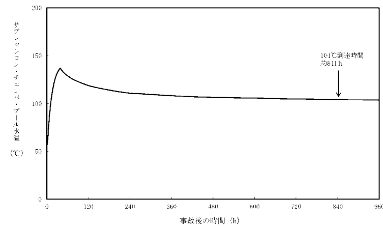
図 1.6 サプレッション・チェンバ・プール水温の推移 (格納容器過圧・過温破損) (代替循環冷却系を使用しない場合)
