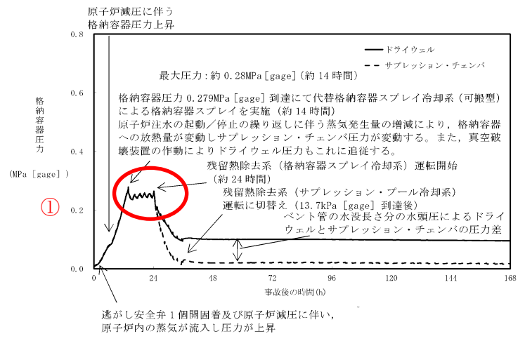
第 2.3.3-16 図 格納容器圧力の推移
