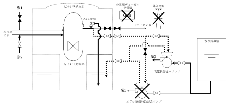
第 2.3.2.2.1 図 「全交流動力電源喪失 (外部電源喪失+DG 喪失)+RCIC 失敗」の重大事故等対策の概略系統図 (1/4) (原子炉注水)
