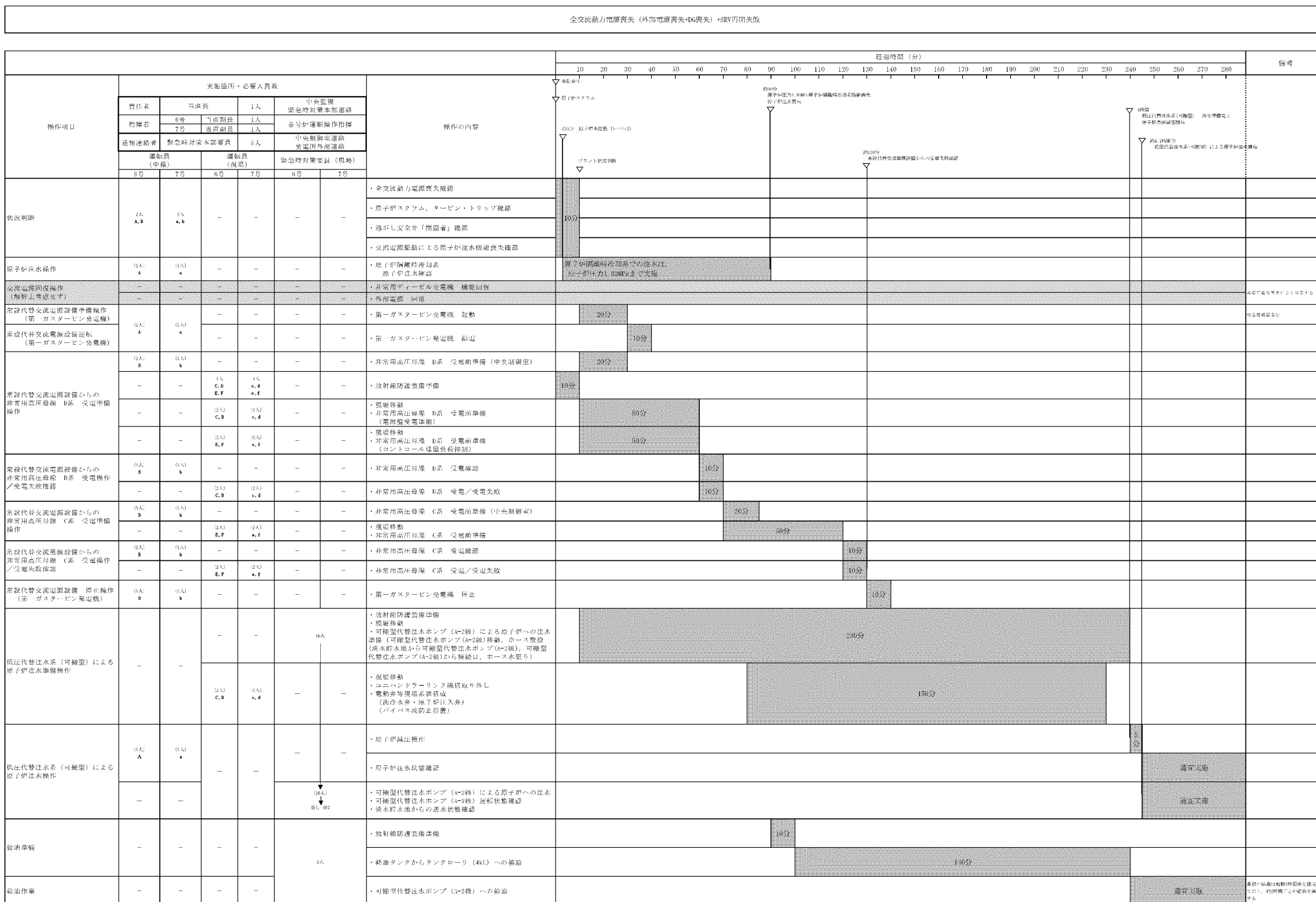
第2.3.4.6図 「全交流動力電源喪失（外部電源喪失+DG 喪失）+SRV 再開失敗」の作業と所要時間(1/2)
