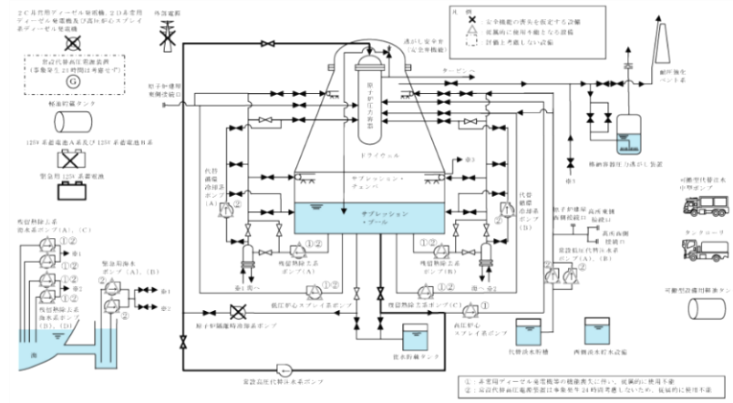
第2.3.2-1 図 全交流動力電源喪失 (TBD, TBU) 時の重大事故等対策の概略系統図 (1/3) (高圧代替注水による原子炉注水段階)
