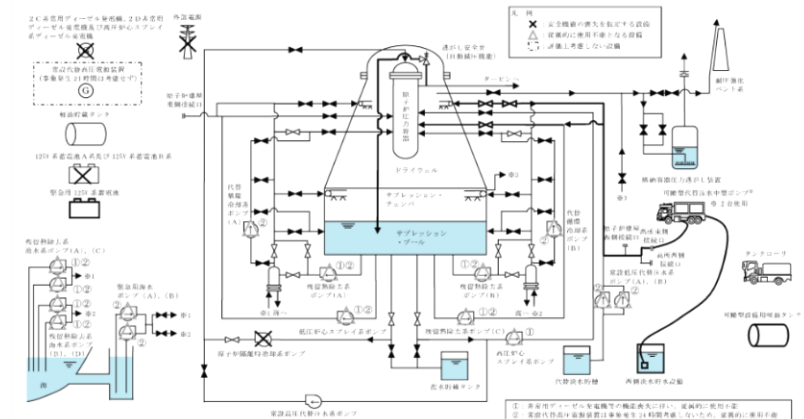
第2.3.2-1 図 全交流動力電源喪失 (TBD, TBU) 時の重大事故等対策の概略系統図 (2/3) (低圧代替注水 (可搬型) による原子炉注水及び代替格納容器スプレイ冷却系 (可搬型) による格納容器冷却段階)
