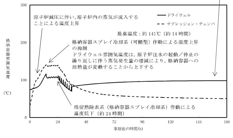
第 2.3.3-17 図 格納容器雰囲気温度の推移
