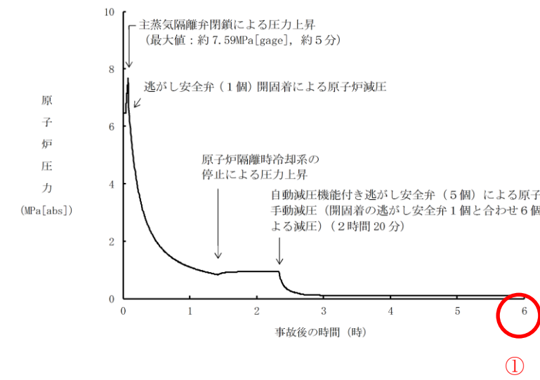
第 2.3.4.2-1(1) 図 原子炉圧力の推移
