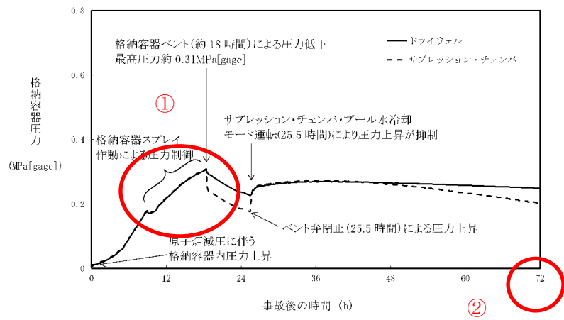
第 2.3.4.19 図 格納容器圧力の推移
