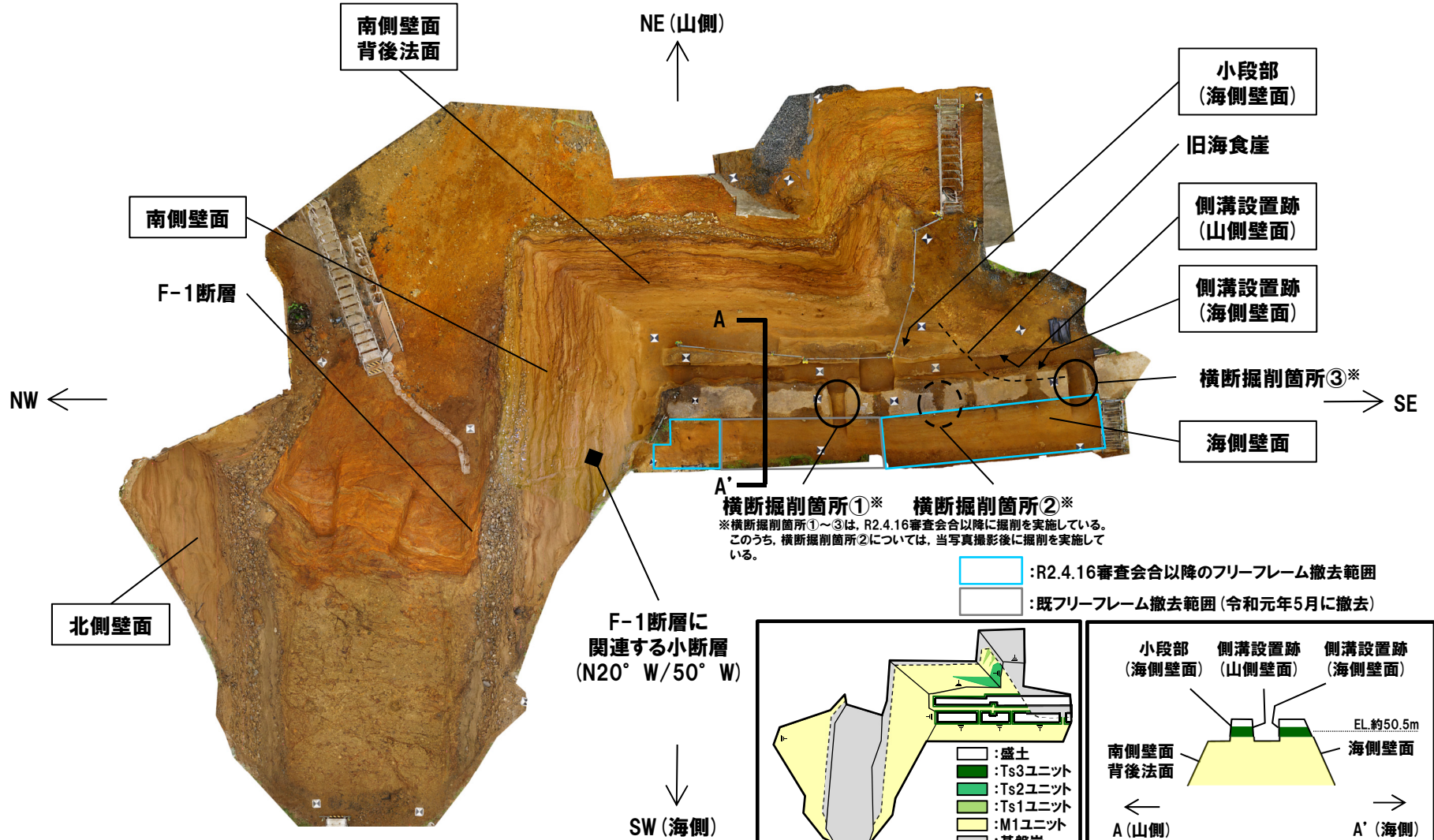
南側壁面の背後法面 天端付近 断面模式図(A-A'断面)
