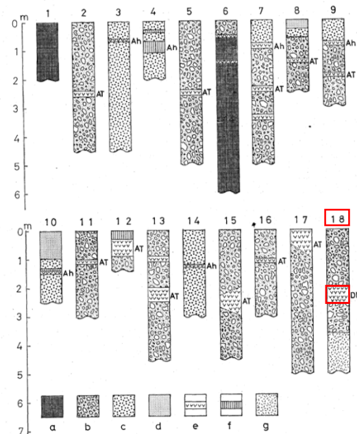
第5図 柱状図
