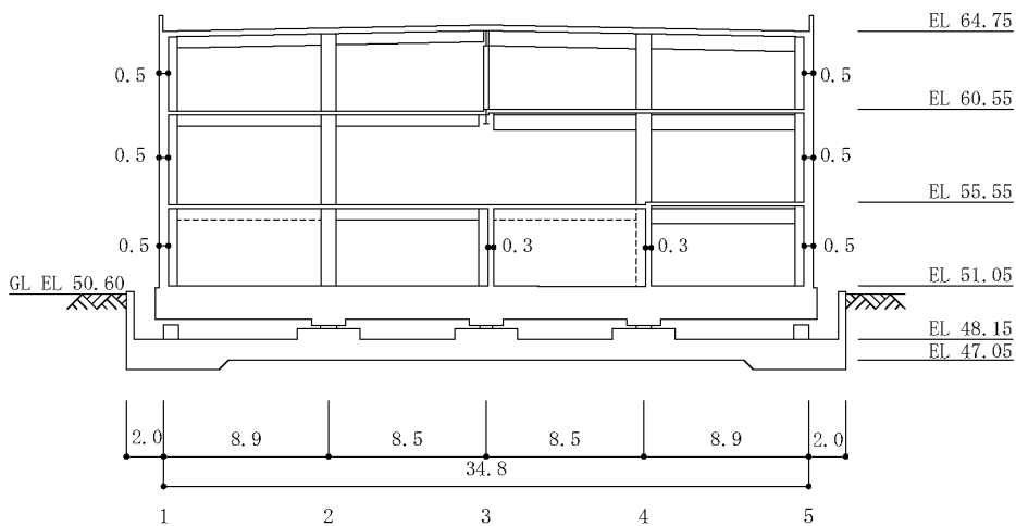
B-B断面（D通り）断面図（X方向）
