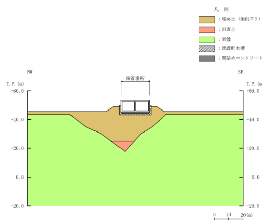
断面図
