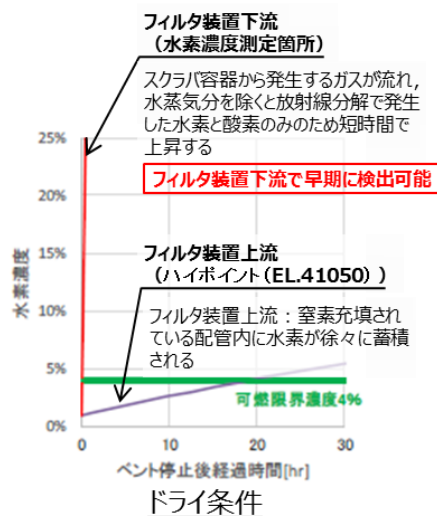
図3 D/W ベント時の格納容器フィルタベント系配管の水素濃度 (ベント停止時の窒素パーージ中断時)
