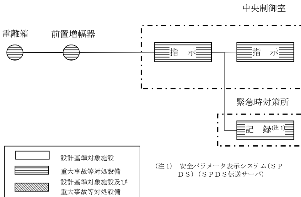
図5 第1ベントフィルタ出口放射線モニタの概略構成図
