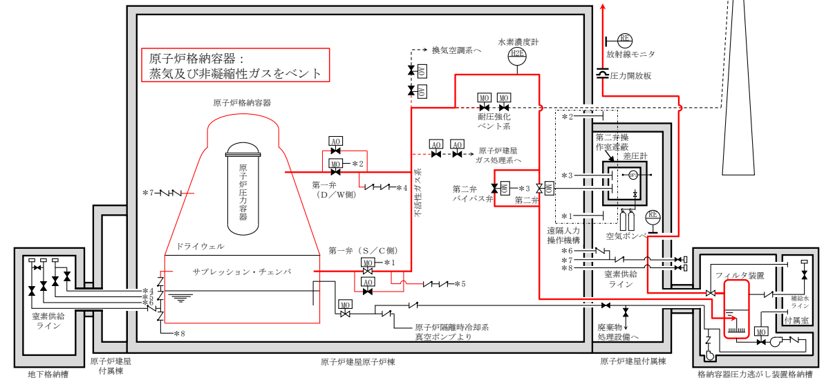
第5図 水素爆発防止対策（系統運転状態）
