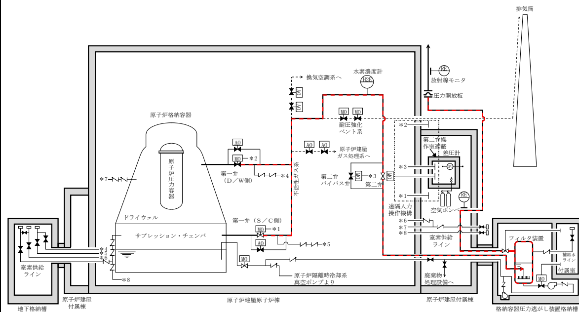
第 4.4-3 図 漏えい試験の試験概要図
