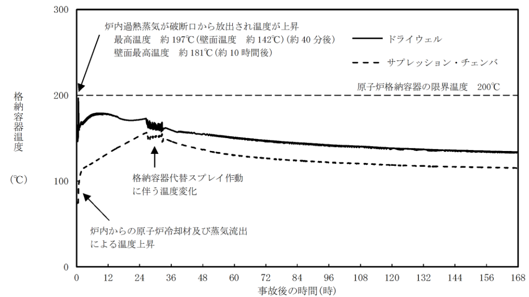
図 2 大 LOCA+SBO+ECCS 機能喪失時における格納容器温度の推移
