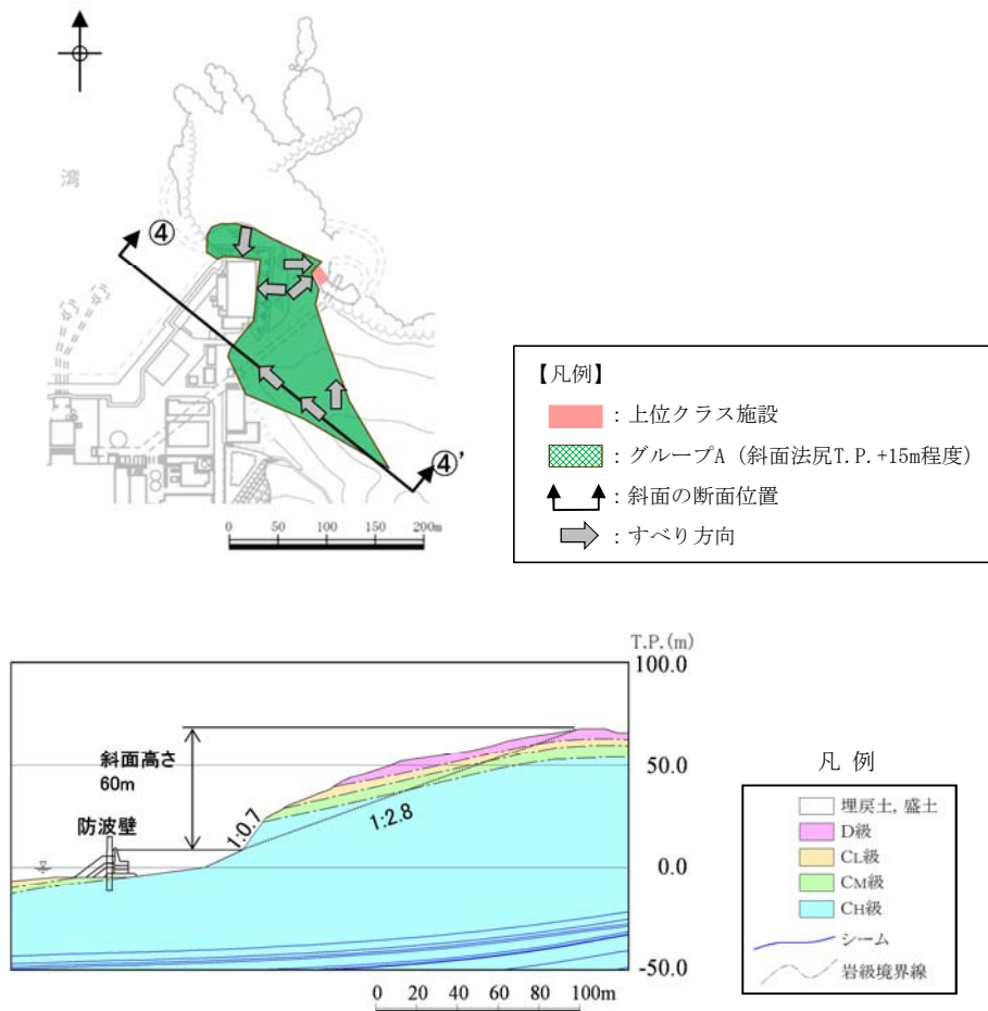
第 20 図 ④-④' 断面の比較結果
