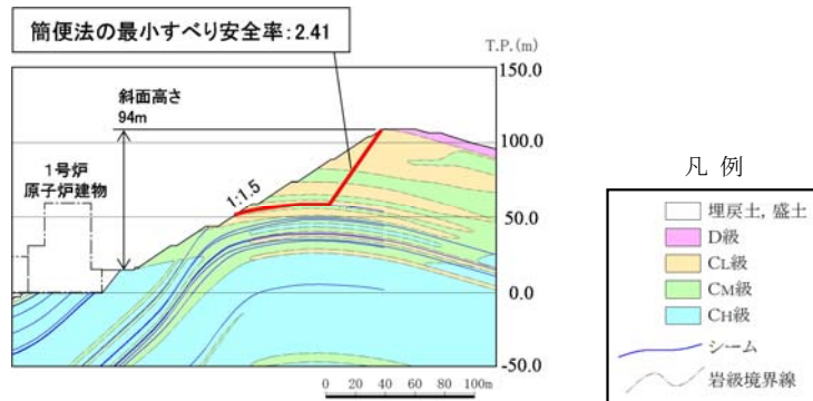
第 19 図 ③-③' 断面の比較結果
