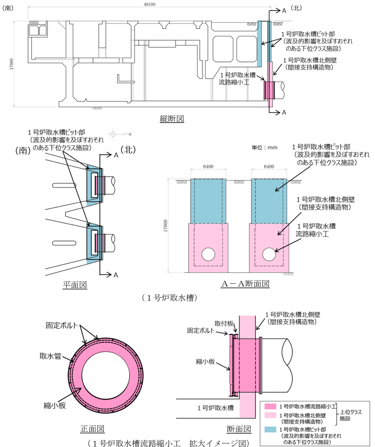
第1図 1号炉取水槽流路縮小工等の範囲
