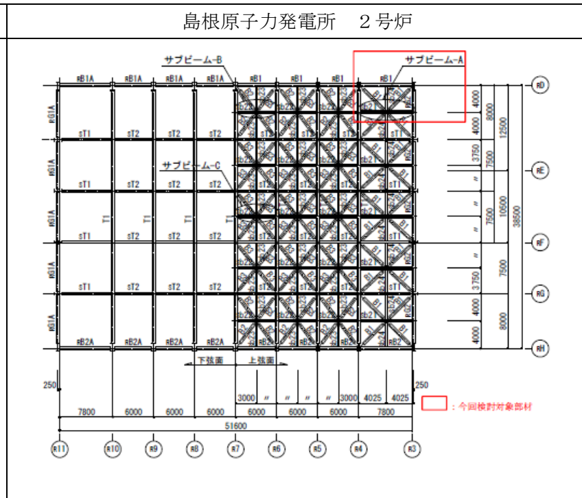
第3-4図 部材位置図 (トラス二次部材: サブビーム)
