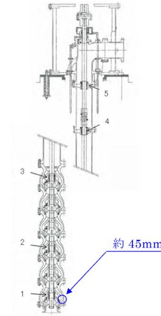
第4図 残留熱除去系海水系ポンプ
