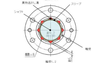
第5図 非常用ディーゼル発電機(高圧炉心スプレイ系ディーゼル発電機を含む。)用海水ポンプ軸受部
