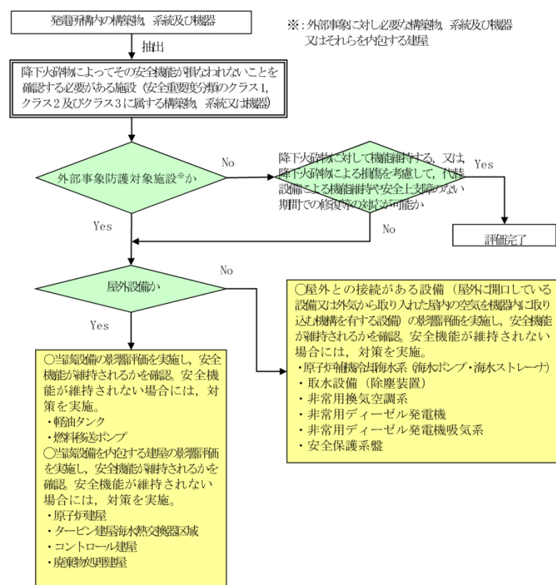
図 1.3 降下火砕物に対する安全施設の評価フロー
