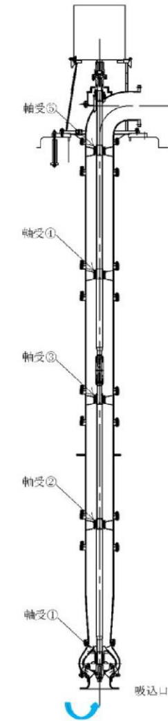
第2-2図 原子炉補機海水ポンプ軸受構造
