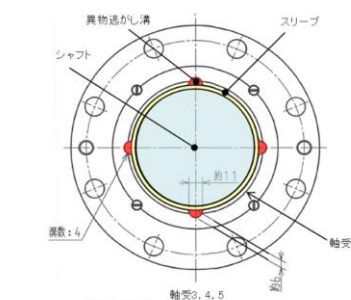
第3図 残留熱除去系海水系ポンプ
