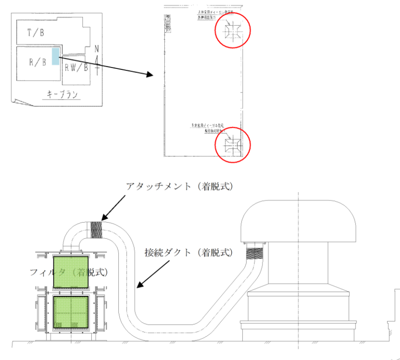
非常用ディーゼル発電機 給気フィルタ (対策案)
