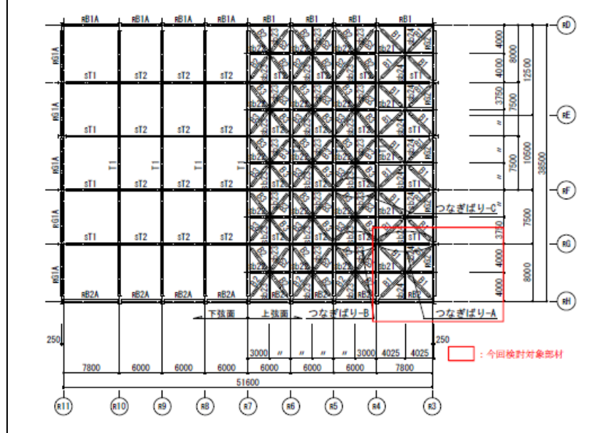
第3-5図 部材位置図 (トラス二次部材: 繋ぎ梁)
