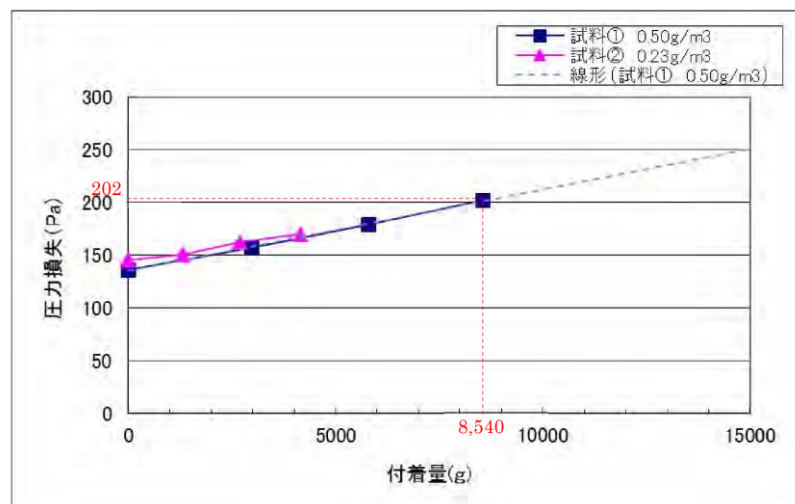
図 7-4 バグフィルタの詰まり試験結果
