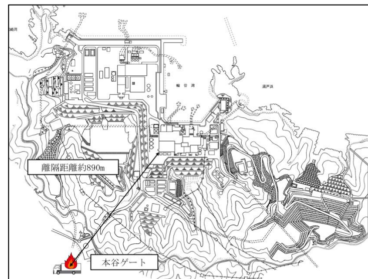
第 2-1 図 燃料輸送車両の離隔距離
