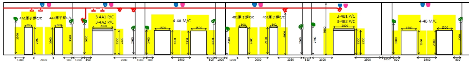
A-A' 断面 (※)
