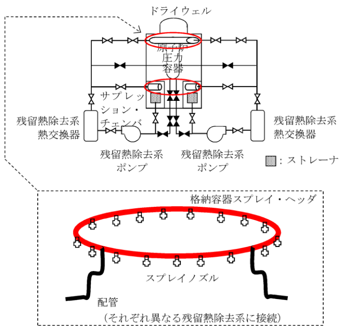
図4 格納容器スプレイ冷却系 系統概略図 (○: 単一設計の静的機器)
