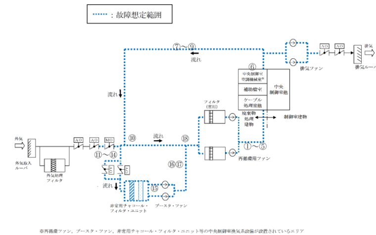
別紙図 1-9-2-1 中央制御室換気系概要図
