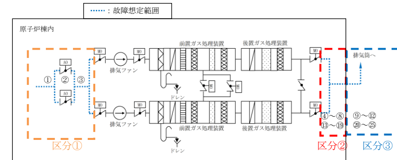
別紙図 1-9-1-1 非常用ガス処理系概略図
