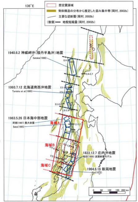
図-2.1.1 秋田県で想定した津波断層の概略の波源域 (「過去の地震の震源モデル・想定震源域、および活断層の分布」(地震調査研究推進本部、日本海東縁部の地震活動の長期評価について、平成15年6月20日、p.42)に加筆)
