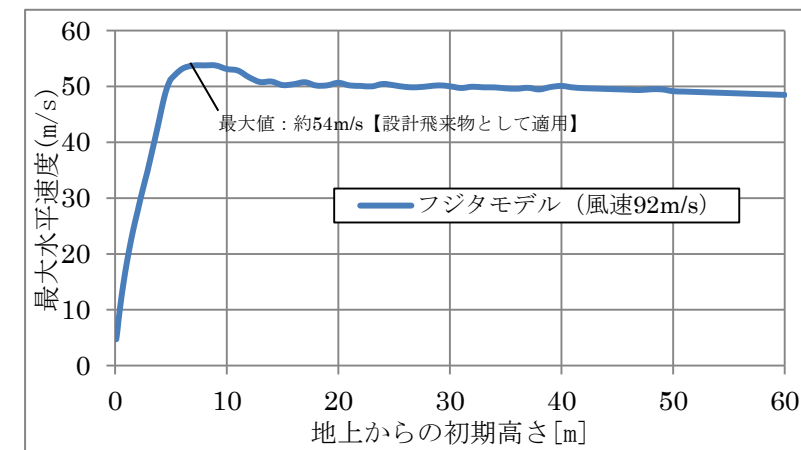
図2 砂利の飛散解析結果 (砂利 : 40mm×40mm×40mm, 0.2kg)
