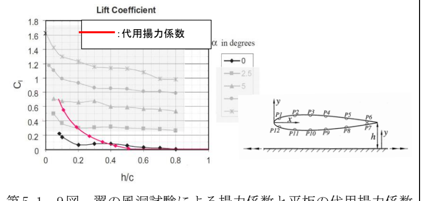
第5.1-9 図 翼の風洞試験による揚力係数と平板の代用揚力係数 (文献 (19) に代用揚力係数を加筆)
