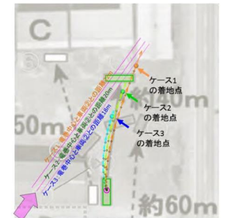
図 30 フジタモデルによるトラック飛散の再現解析結果
