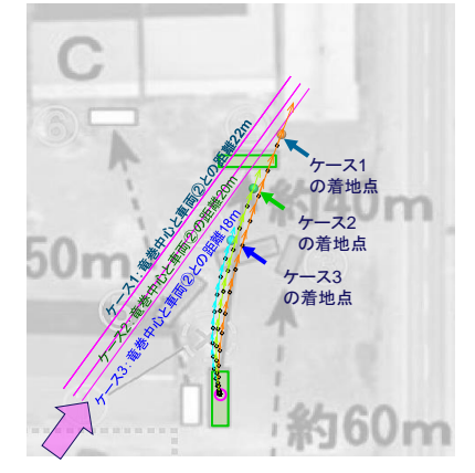
第 6.3-2 図 フジタモデルによる 4t トラックの飛散解析結果 (文献 (27) の写真に軌跡を加筆)
