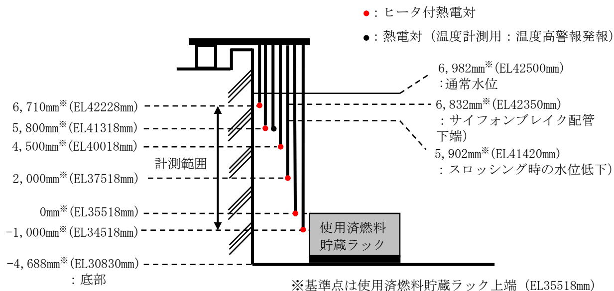
第 1.2 - 11 図 燃料プール水位・温度（S A）の設置図
