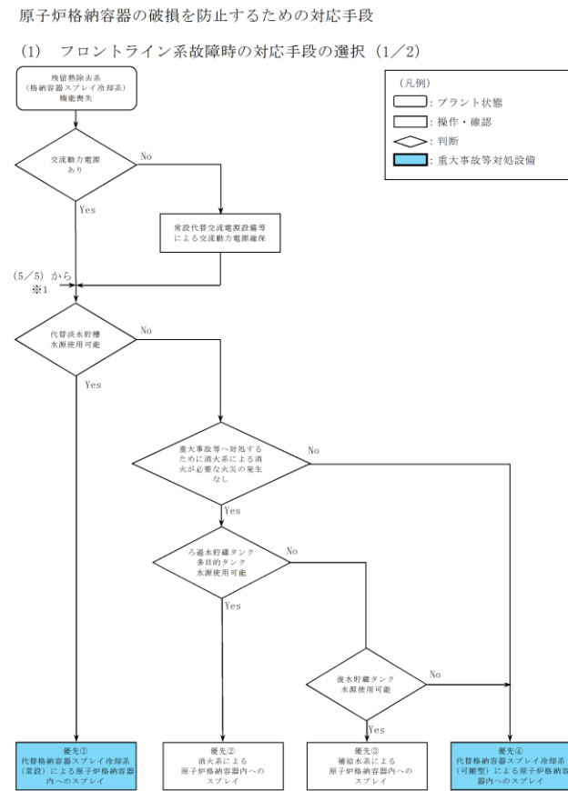
第 1.6-29 図 重大事故等時の対応手段選択フローチャート
