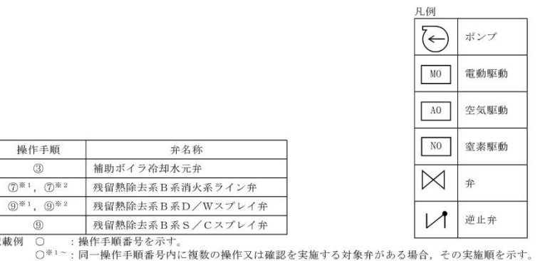
第 1.6-11 図 消火系による原子炉格納容器内へのスプレイ 概要図
