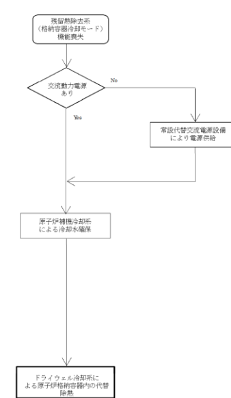
原子炉格納容器破損を防止するための対応手段 (1) フロントライン故障時の対応手段の選択 (2/2)
