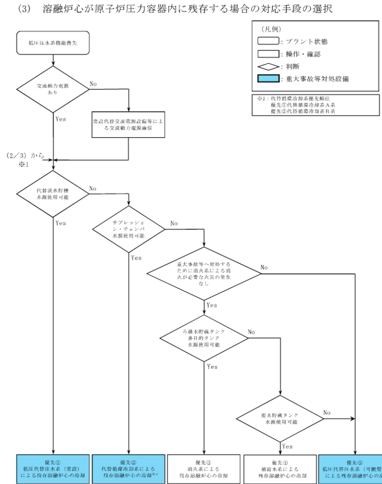
第1. 4-35図 重大事故等時の対応手段選択フローチャート (3 / 3)
