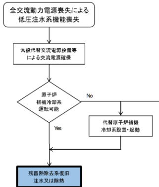
第 1.4.32 図 重大事故等発生時の対応手段選択フローチャート
