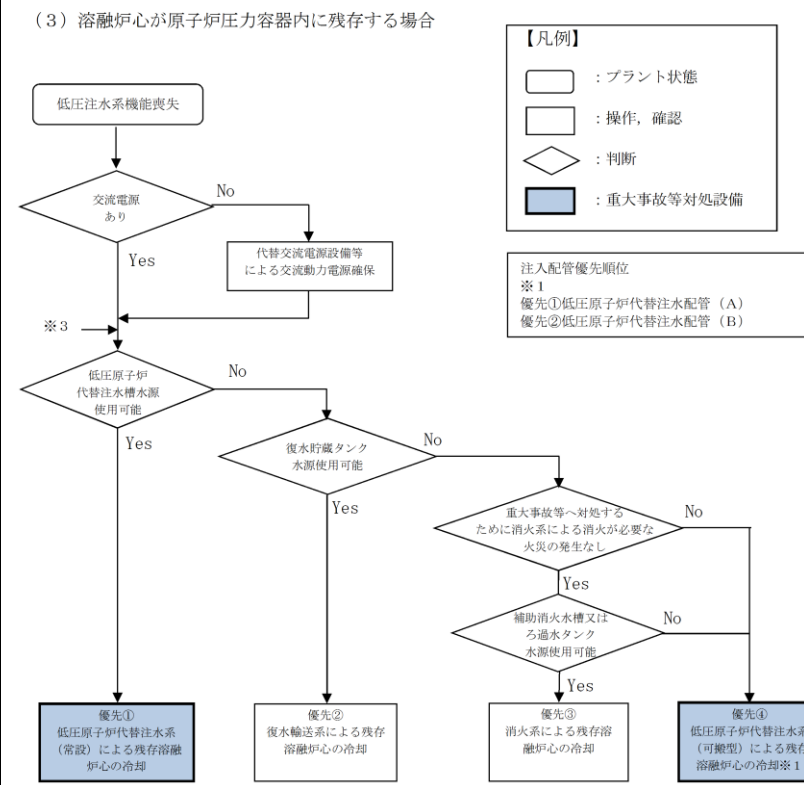
第 1. 4-33 図 重大事故等発生時の対応手段選択フローチャート (3 / 3)
