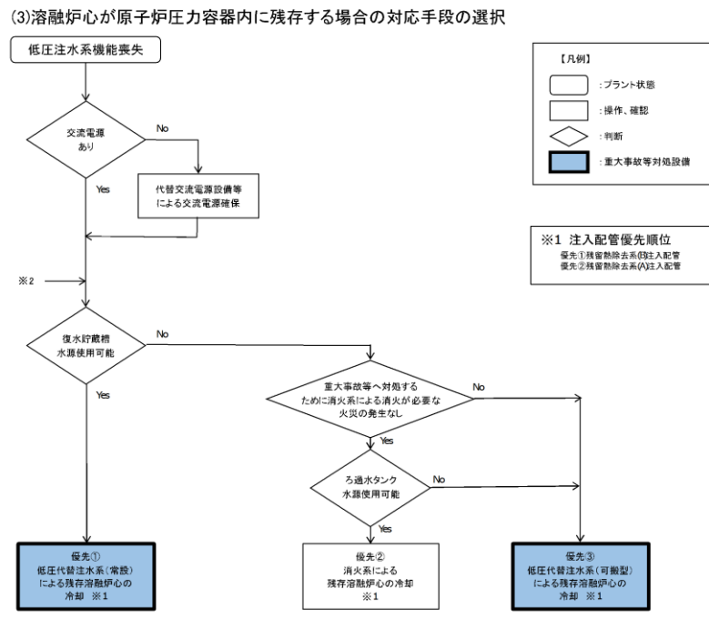
第 1. 4. 32 図 重大事故等発生時の対応手段選択フローチャート (2 / 2)
