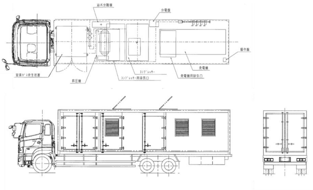
图 2.8.4-2 可搬式氮素供給装置 構造図
