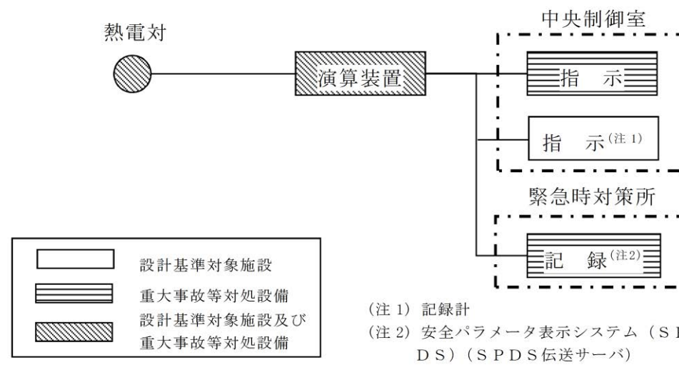
第 58-6-60 図 燃料プール水位・温度 (SA) の概略構成図(2)
