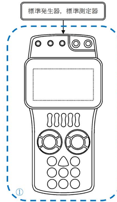
① 搬型計測器に模擬入力を実施し計器の校正を実施 (点検・検査)
