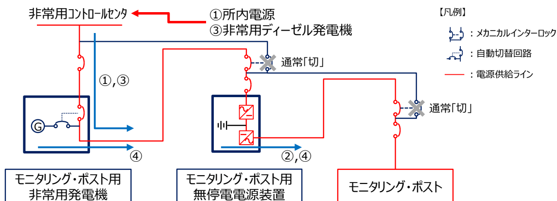
第 1 図 モニタリング・ポストの電源構成概要図
