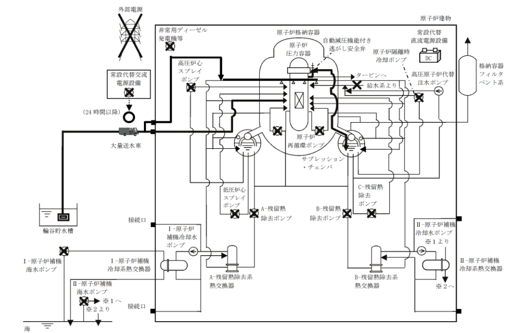
図2 「全交流動力電源喪失(外部電源喪失+DG失敗)+高圧炉心冷却失敗」の重大事故等対策の概略系統図(原子炉減圧, 原子炉注水及び原子炉格納容器冷却)
