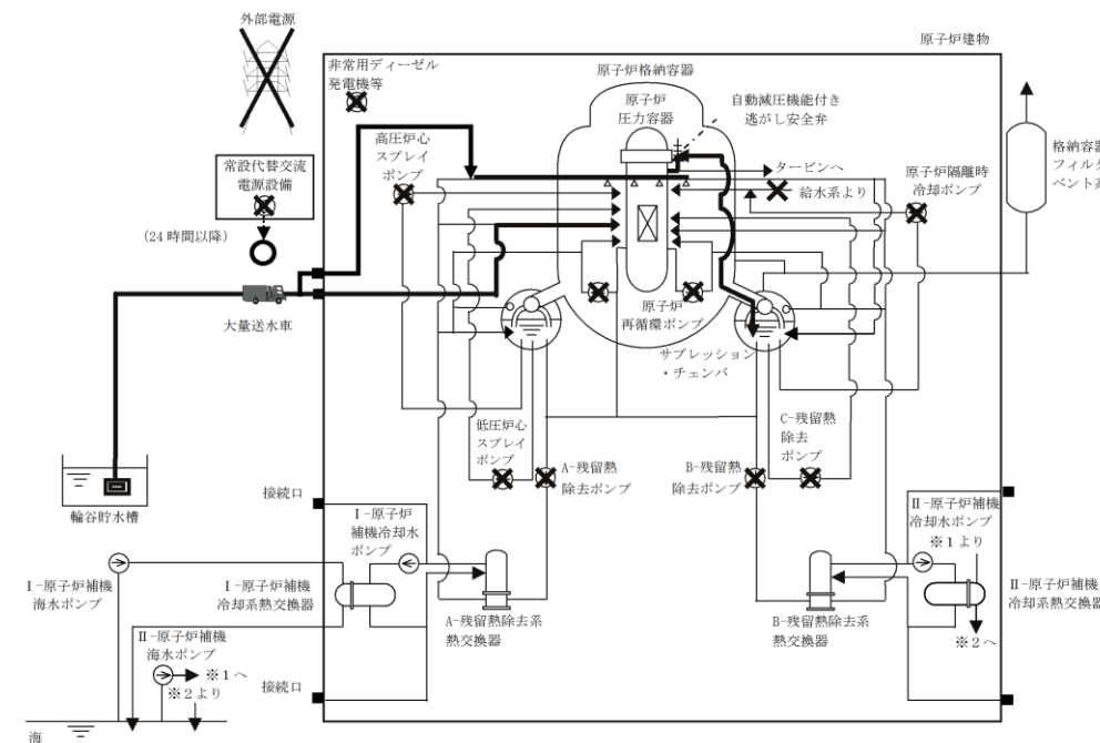
図4 「全交流動力電源喪失（外部電源喪失+DG失敗）+SRV再開失敗 +HPCS失敗」の重大事故等対策の概略系統図 (原子炉減圧，原子炉注水及び原子炉格納容器冷却)
