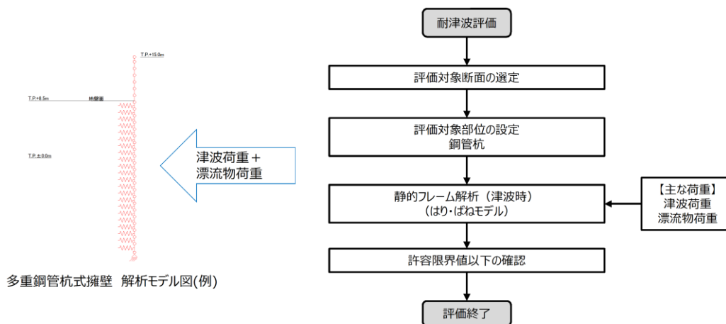
第 1-106 図 設計フロー
