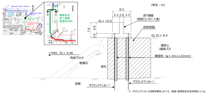
第 1-19(5) 図 防波壁 (鋼管杭式逆 T 擁壁) 防波扉北側部 (⑤-⑤断面) 断面 図
