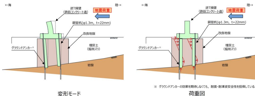
第1-75図 防波壁（鋼管杭式逆T擁壁）の変形モード及び荷重図（地震時）
