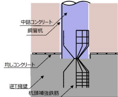
杭頭部 拡大図
