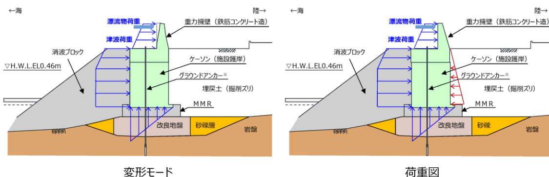
第 1-76 図 防波壁（波返重力擁壁）の変形モード及び荷重図（地震時）
