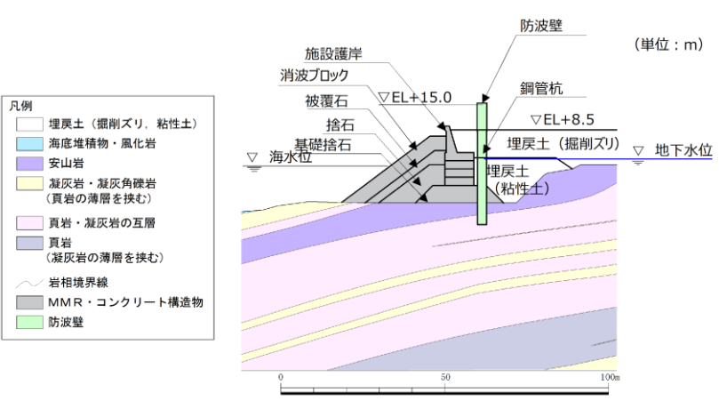
第 1-56 図 防波壁（多重鋼管杭式擁壁）の地質断面図（①-①）
