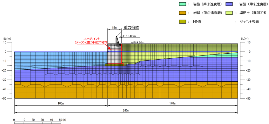
第7図 波返重力擁壁の解析モデル図 (例)
