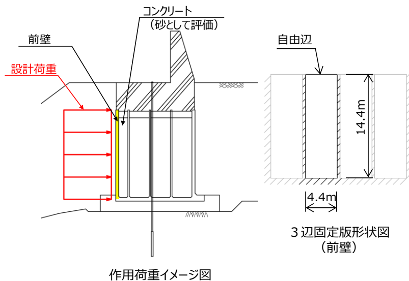
第 1-108 図 防波壁（波返重力擁壁）ケーソンの作用荷重イメージ図
