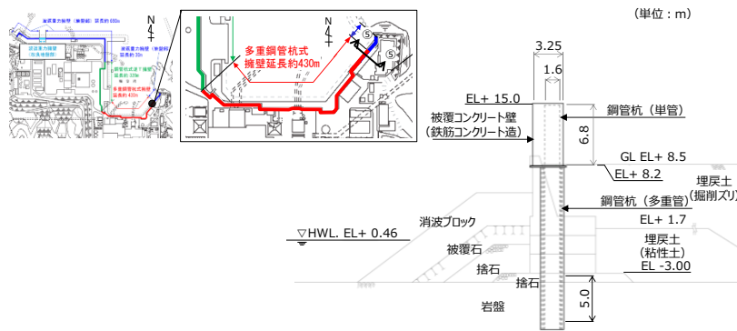
第 1-14(5) 図 防波壁 (多重鋼管杭式擁壁) 北東端部 (⑤-⑤断面) 断面図
