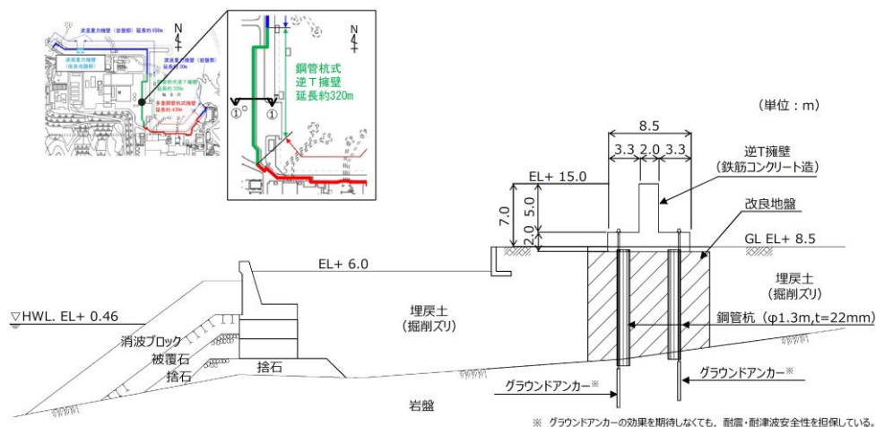
第 1-19(1) 図 防波壁（鋼管杭式逆 T 擁壁）荷揚護岸北側部（①－①断面）断面図
