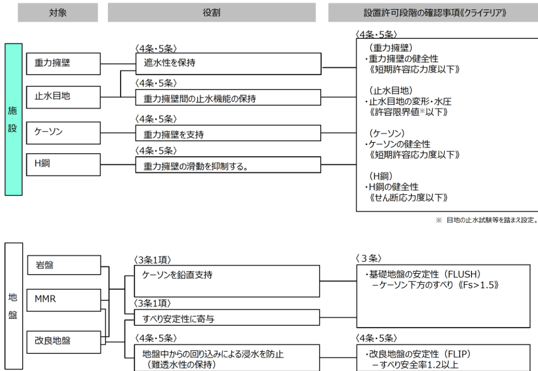
第 1-103 図 設置許可段階における確認項目 [防波壁 (波返重力擁壁)]
