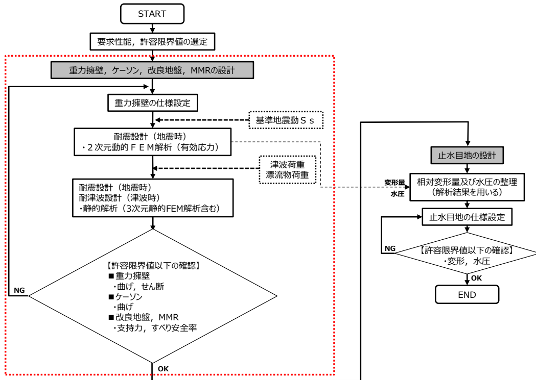
第 1-100 図 防波壁（波返重力擁壁）の設計フロー
