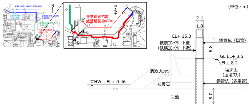
第 1-14(6) 図 防波壁 (多重鋼管杭式擁壁) 西端部 (⑥-⑥断面) 断面図
