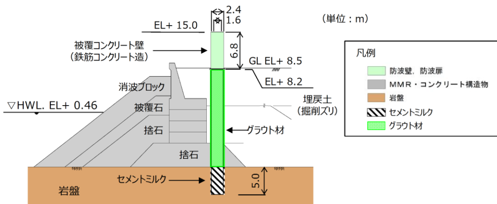
第 1-86 図 防波壁（多重鋼管杭式擁壁）弱部③概要図（杭間部（A-A 断面）断面図）
