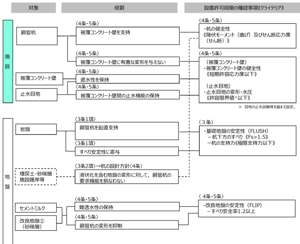
第 1-95 図 設置許可段階における確認項目 [防波壁（多重鋼管杭式擁壁）]
