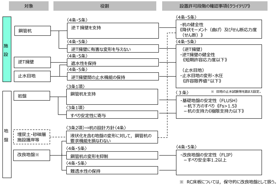
第 1-99 図 設置許可段階における確認項目 [防波壁 (鋼管杭式逆T擁壁)]
