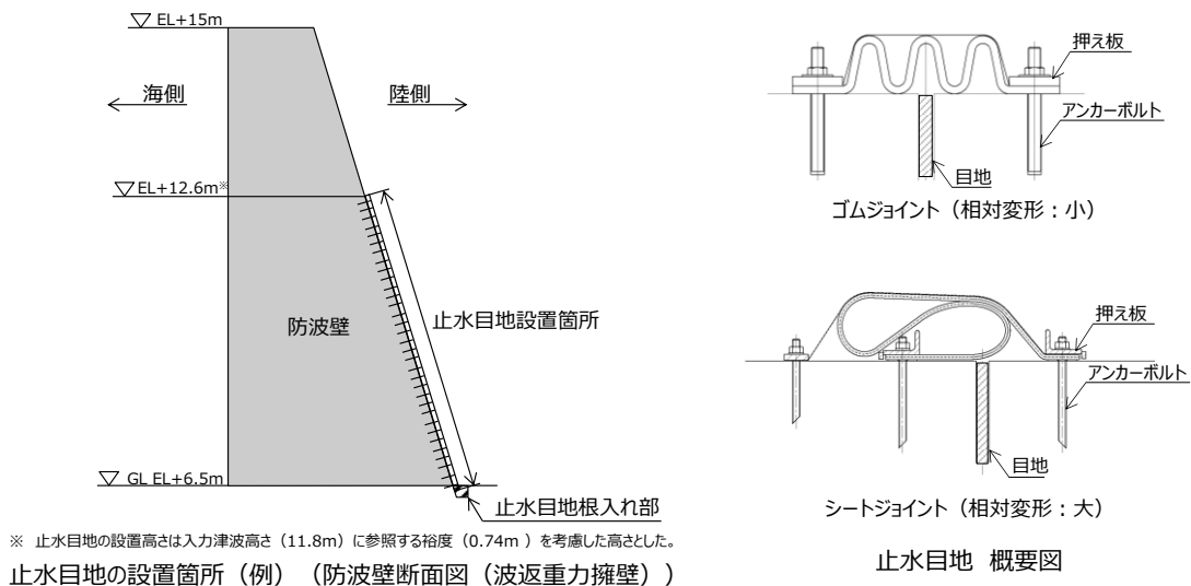
第 1-50 図 防波壁の止水目地の設置箇所及び概要図
