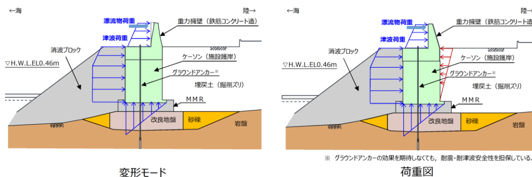
第1-79図 防波壁（波返重力擁壁）の変形モード及び荷重図（津波時）
