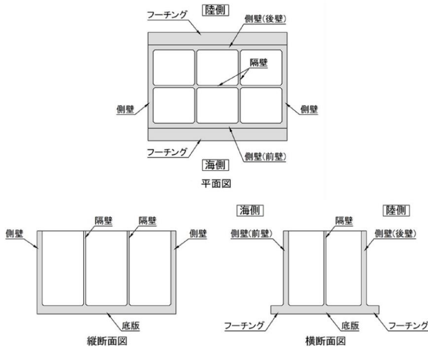
第5図 ケーソン各部の名称（港湾基準 図-参 1.2.1 を加筆・修正）
