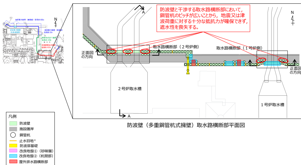
第 1-82 図 防波壁（多重鋼管杭式擁壁）弱部②概要図（取水路横断部）
