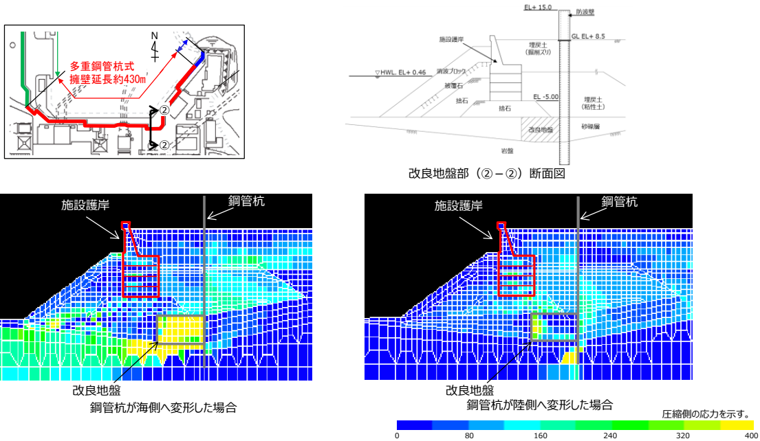
第 1 図 鋼管杭の曲げモーメント最大時刻における水平有効応力分布図 (改良地盤部 (2-2))
