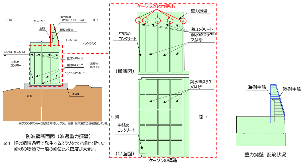
第4図 防波壁（波返重力擁壁）ケーソンの構造
