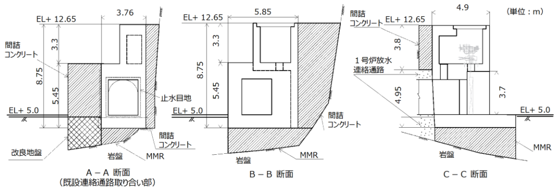
第 1-30 図 1 号放水連絡通路防波扉の断面図 (1)
