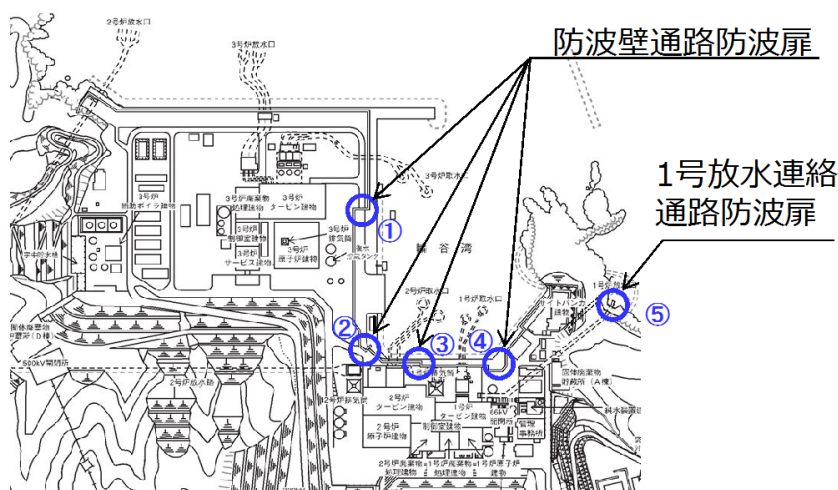
第1-34図 防波壁通路防波扉の位置図
