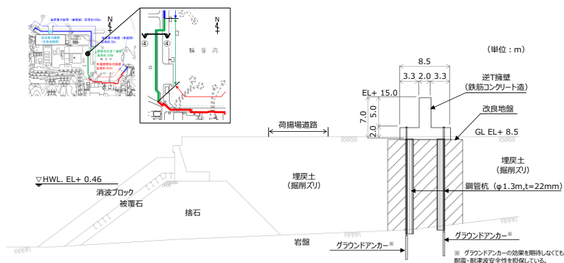
第 1-19(4) 図 防波壁（鋼管杭式逆 T 擁壁）防波扉南側部（④-④断面） 断面図
