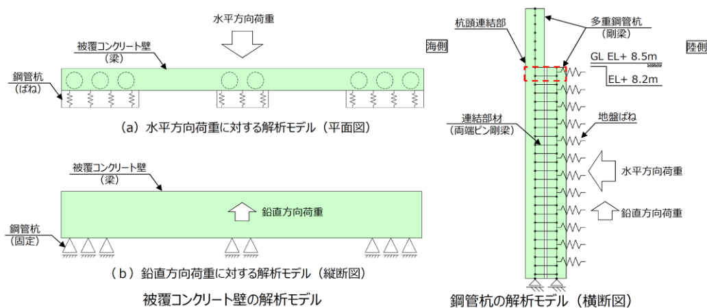
第 1-107 図 解析モデル
