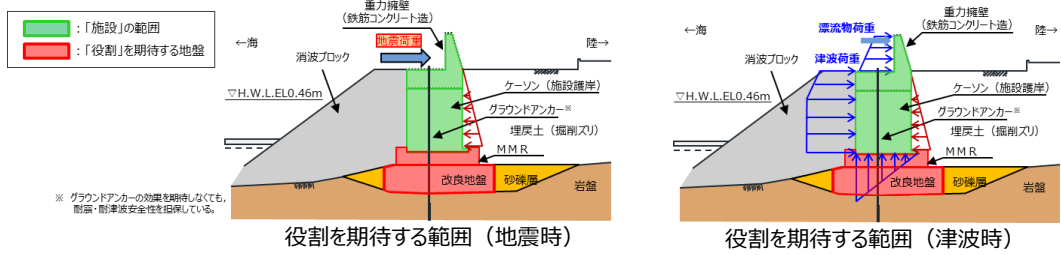
第 1-8 図 防波壁（波返重力擁壁）の役割を期待する範囲
