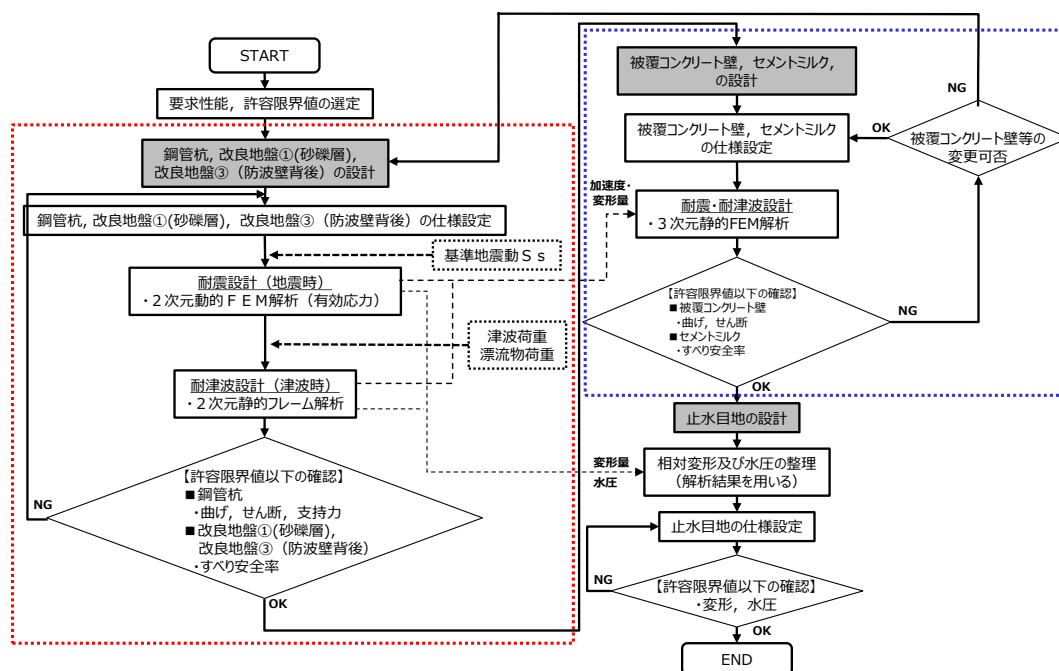
第 1-92 図 防波壁（多重鋼管杭式擁壁）の設計フロー
