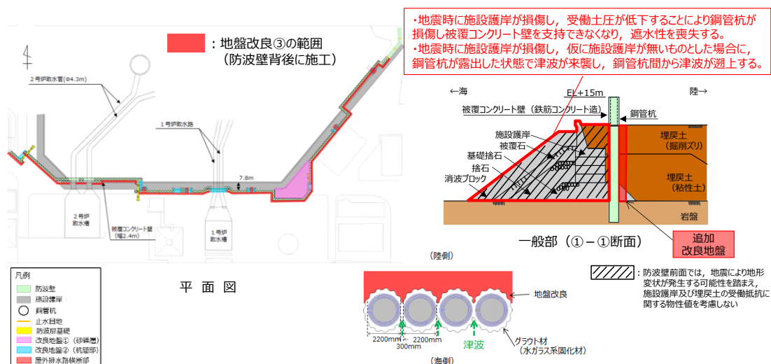
第 1-87 図 防波壁（多重鋼管杭式擁壁）弱部③概要図
