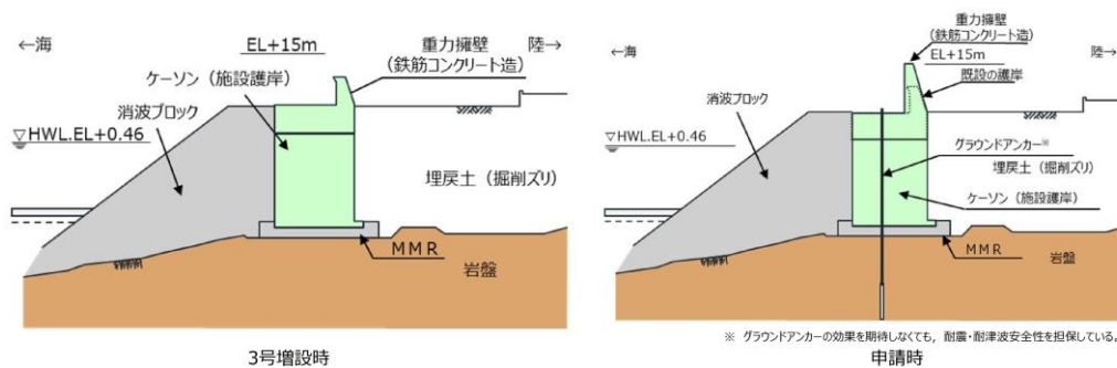
第1図 防波壁（波返重力擁壁）断面図
