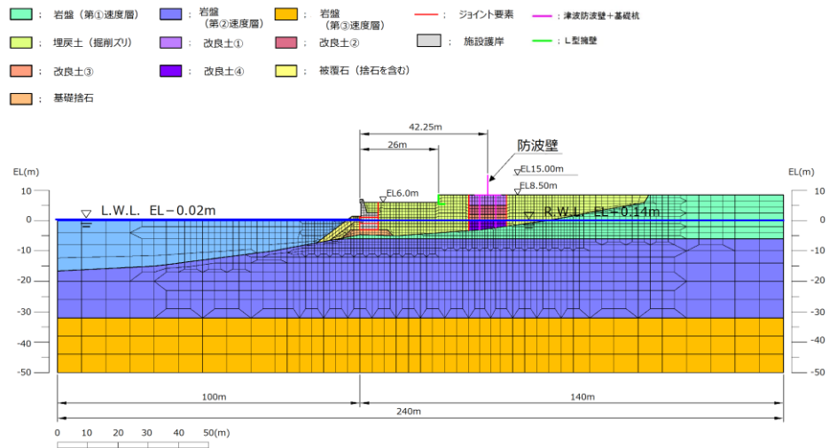
第 2-26 図 地下水位概要図（地震時）
