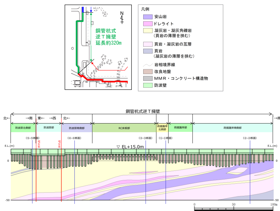
第 1-61 図 防波壁（鋼管杭式逆T擁壁）の岩相縦断図
