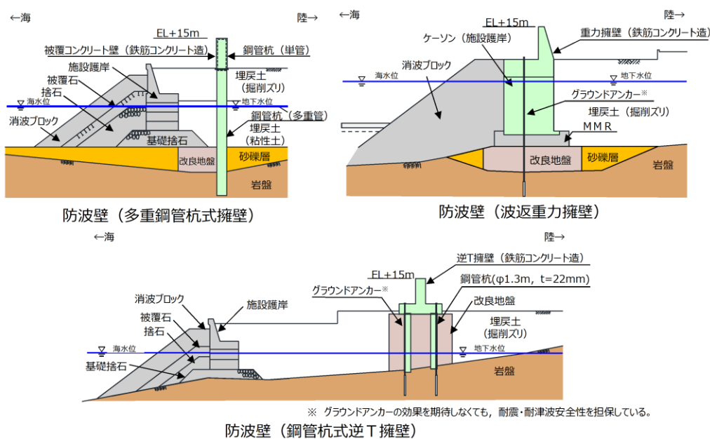
第 1-111 図 地下水位設定の概要
