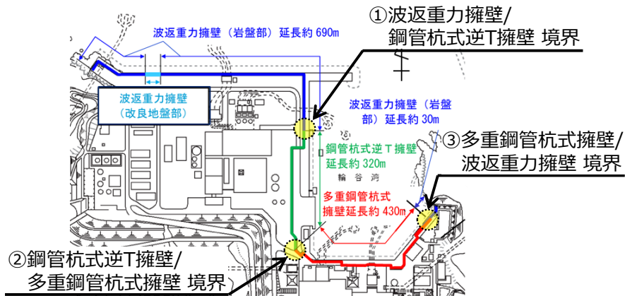
第 1-51 図 防波壁の構造形式の境界位置図
