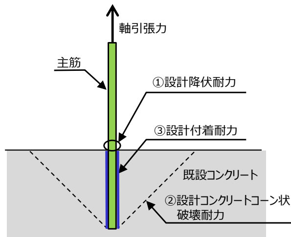
第3図 あと施工アンカーとして考えた時の主筋定着部の確認項目
