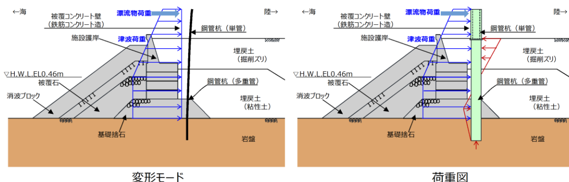
第 1-77 図 防波壁（多重鋼管杭式擁壁）の変形モード及び荷重図（津波時）
