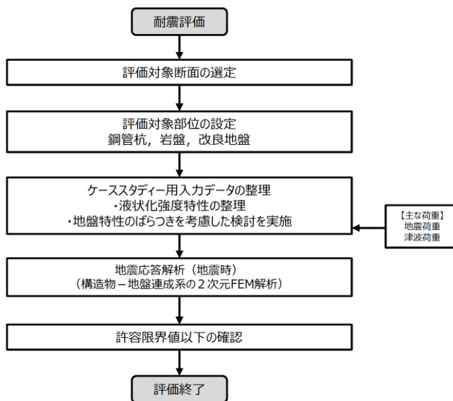
第 1-105 図 設計フロー
