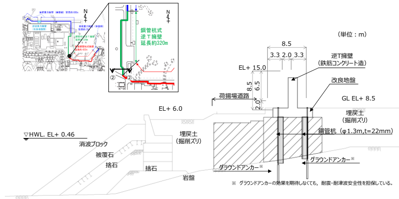
第 1-19(2) 図 防波壁（鋼管杭式逆 T 擁壁）荷揚護岸南側部（②-②断面） 断面図
