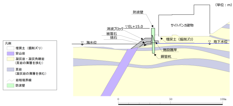
第 1-60 図 防波壁 (多重鋼管杭式擁壁) の地質断面図 (⑤-⑤)
