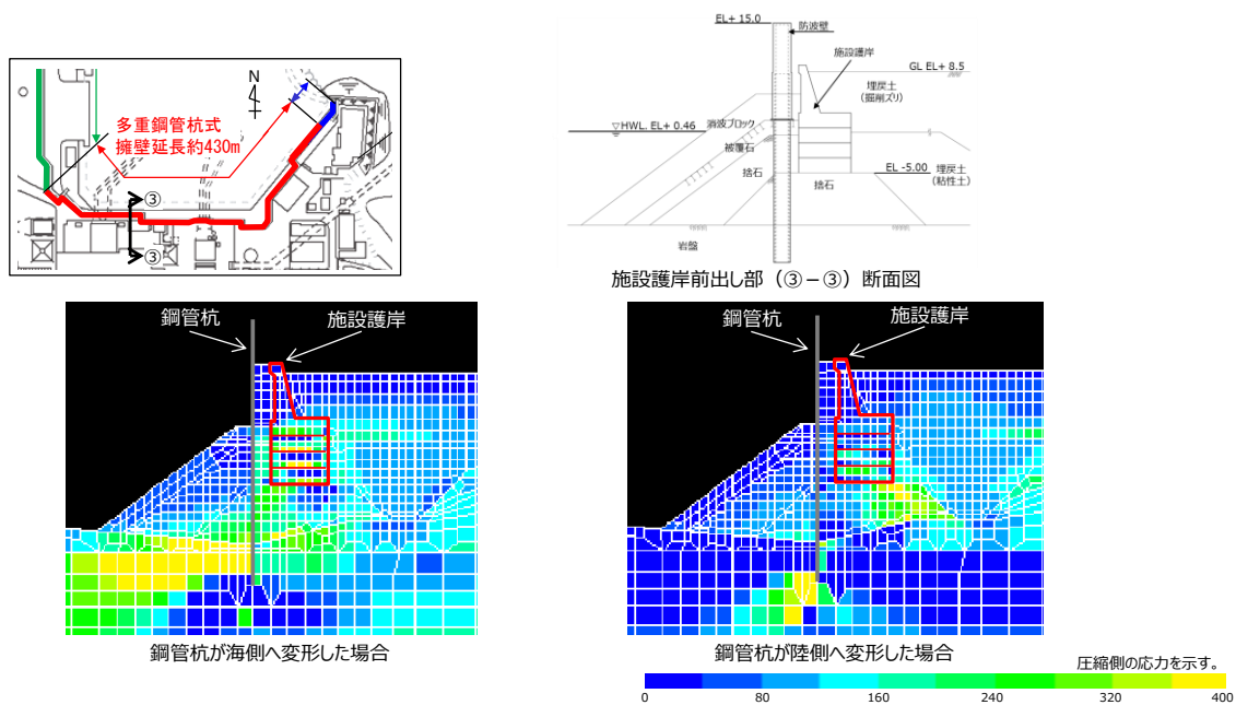
第 2 図 鋼管杭の曲げモーメント最大時刻における水平有効応力分布図 (施設護岸前出し部 (3-3))
