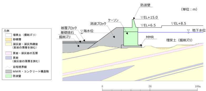
第 1-68 図 防波壁（波返重力擁壁）の地質断面図 (①-①)
