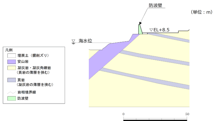
第 1-72 図 防波壁 (波返重力擁壁) の地質断面図 (⑤-⑤)
