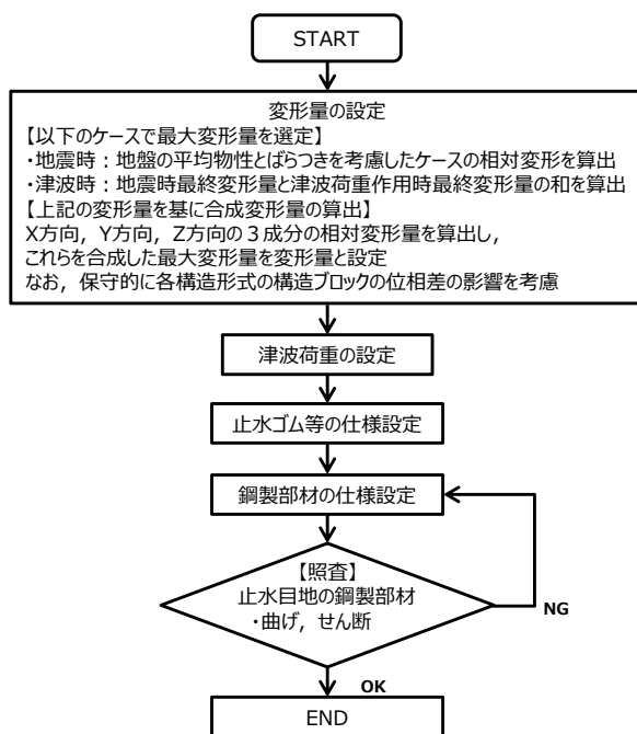
第 1-104 図 設計フロー
