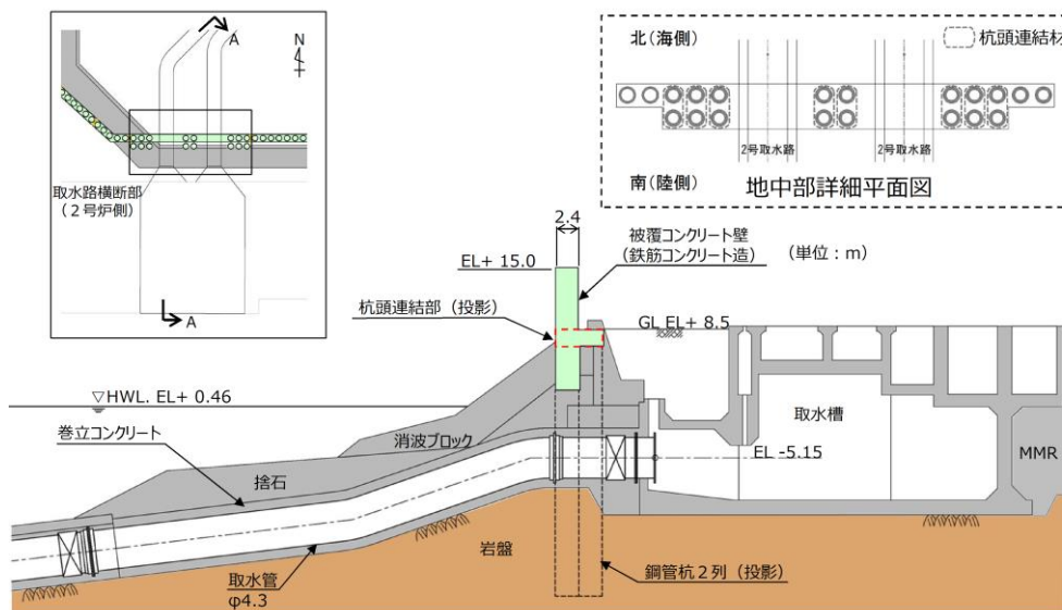
第 1-84 図 防波壁（多重鋼管杭式擁壁）弱部②概要図（取水路横断部（2号炉側，A-A断面）断面図）
