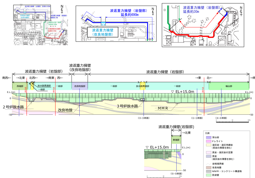
第 1-66 図 防波壁（波返重力擁壁）の岩相縦断図
