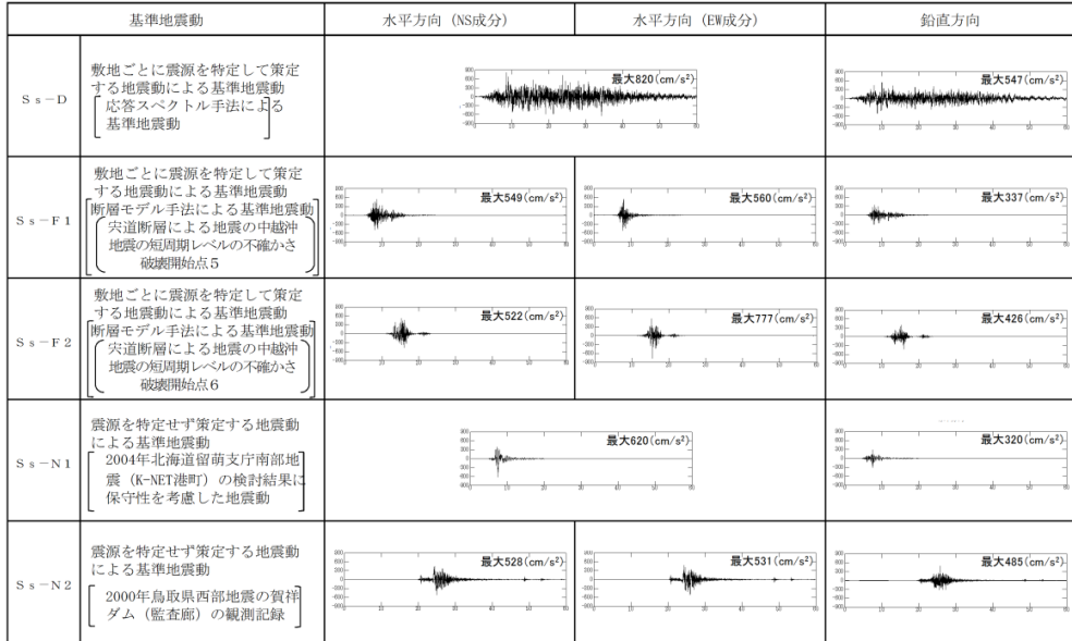
第 1-112 図 基準地震動 S s の時刻歴波形
