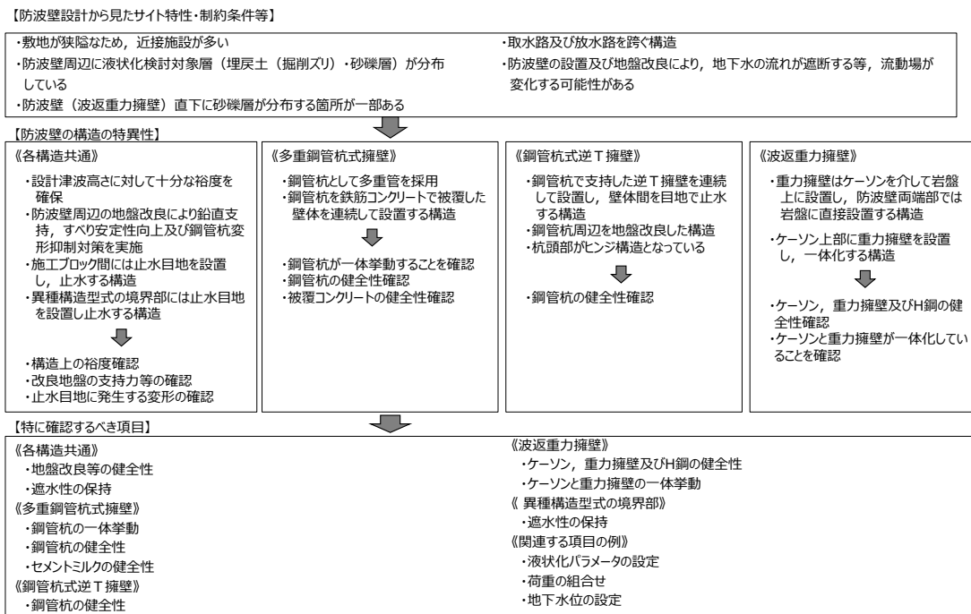
第1-80図 防波壁の各構造の特異性と特に確認すべき項目の整理
