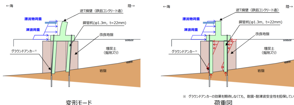
第1-78図 防波壁（鋼管杭式逆T擁壁）の変形モード及び荷重図（津波時）
