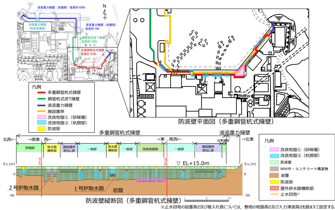
第 1-12 図 防波壁（多重鋼管杭式擁壁）の縦断図
