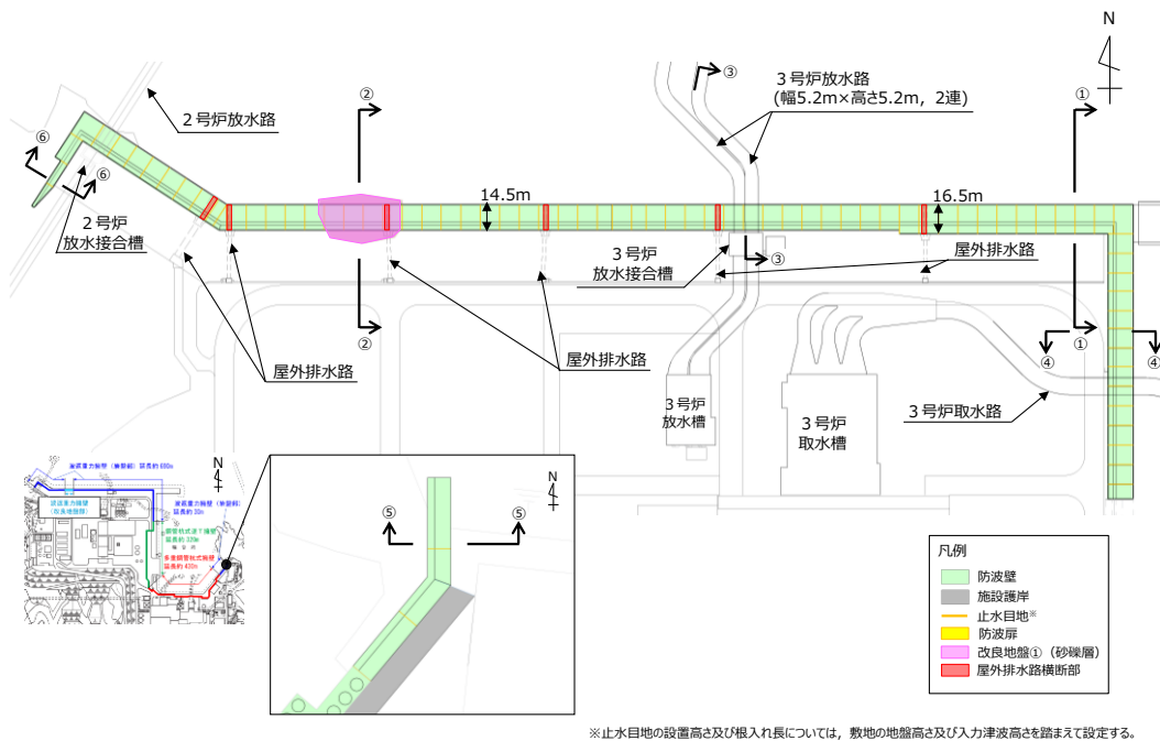
第 1-23 図 防波壁 (波返重力擁壁) の平面図
