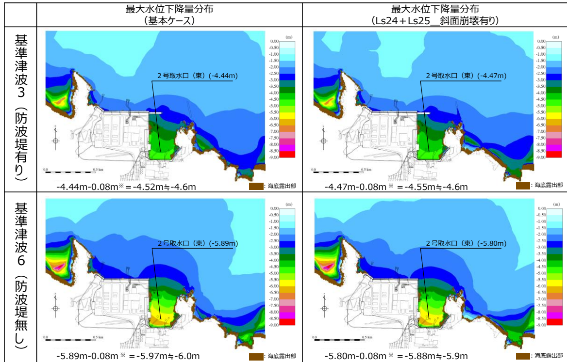
図2-54(4) 斜面崩壊(Ls24+Ls25)の有無による最大水位下降量分布の比較 (基準津波3(防波堤有り)及び基準津波6(防波堤無し))
