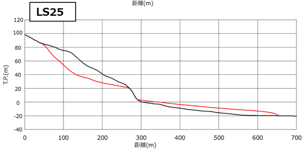
図 2 - 53 Ls24・Ls25の断面図
