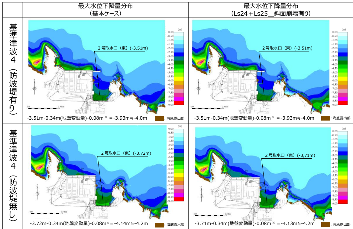
図2-54(5) 斜面崩壊(Ls24+Ls25)の有無による最大水位下降量分布の比較 (基準津波4(防波堤有り)及び基準津波4(防波堤無し))
