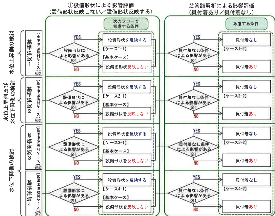
図-1-4-3 影響評価検討フロー
