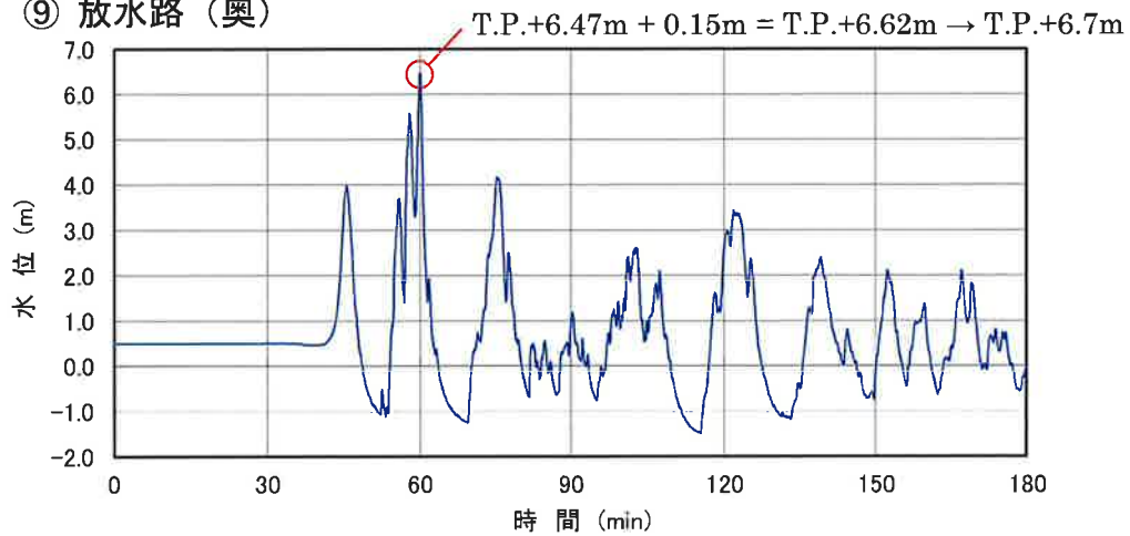
図-1-6-2 入力津波の時刻歴波形 (3/5)
