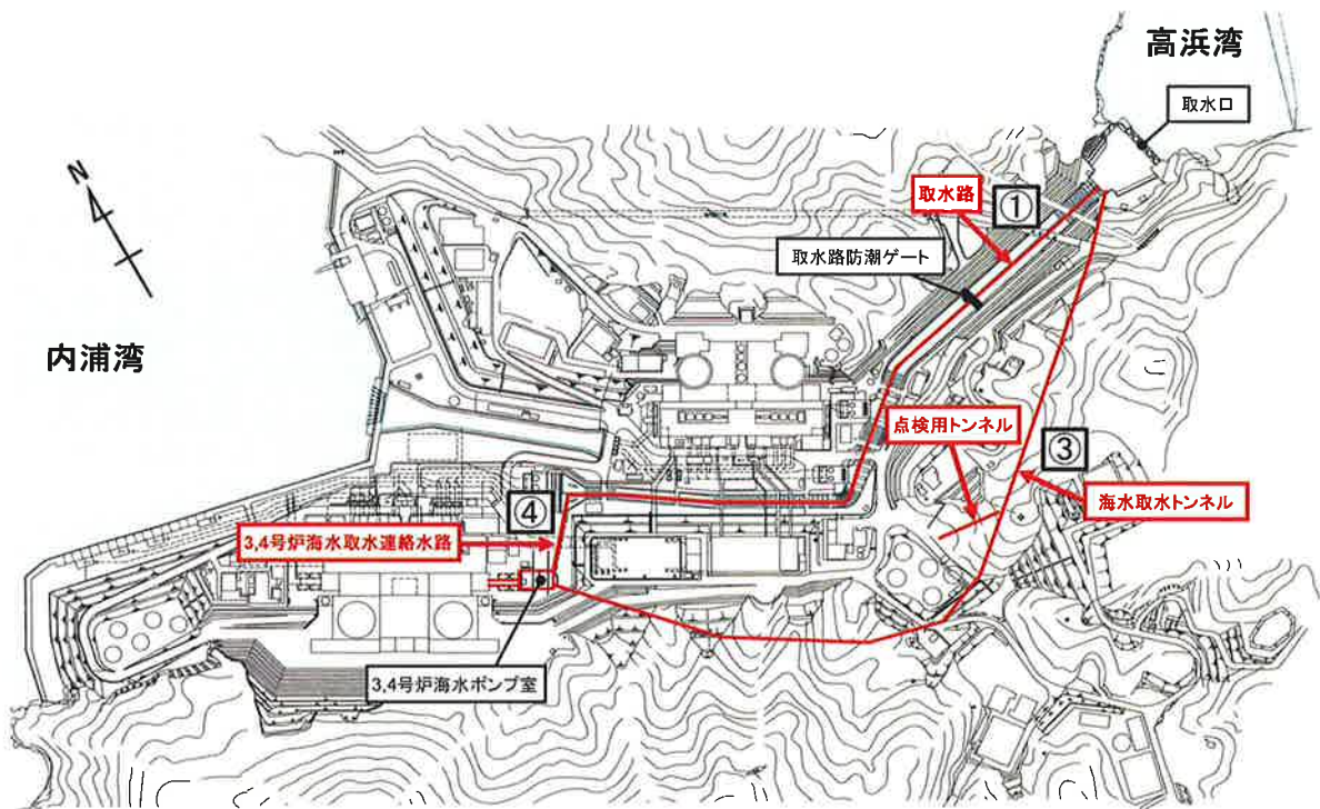
図-2-2-22 3, 4号炉海水取水系配置図
