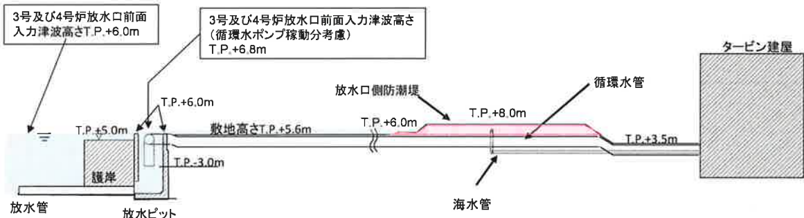
図-2-2-51 3号及び4号炉 放水路系配置図
