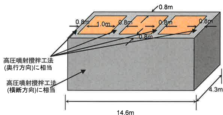
図-3-1-10 地盤改良工法（高压喷射搅拌工法）概念図
