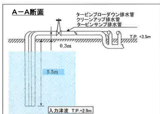
図-2-2-41 3, 4号炉循環水ポンプ室付近排水管路経路図
