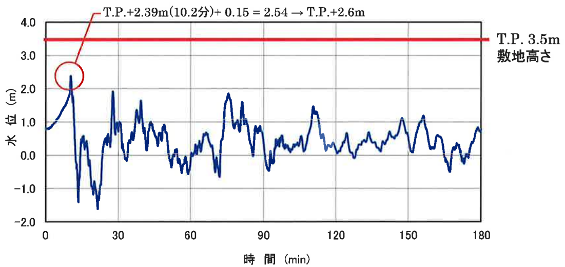
図-2-2-21 2号炉海水ポンプ室 津波波形
