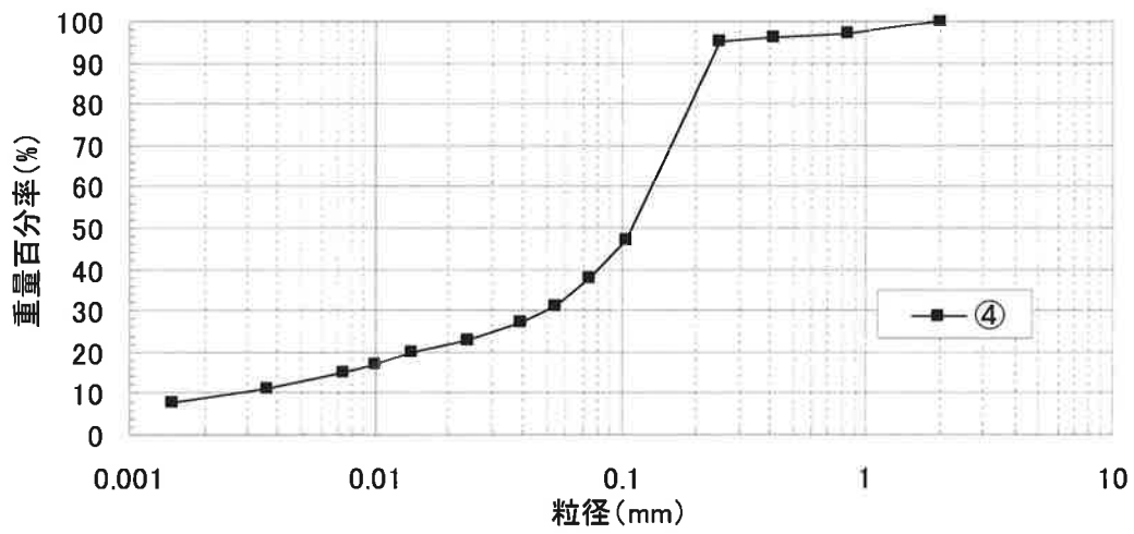
図-2-5-8 粒径加積曲線 (調査地点④)
