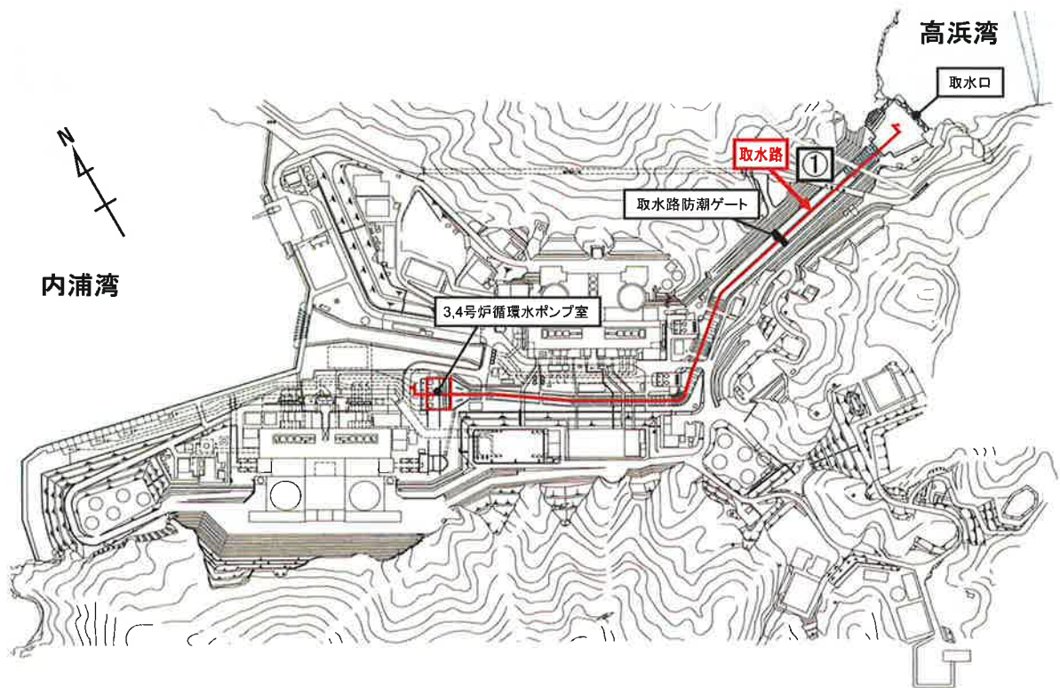
図-2-2-29 3,4号炉海水取水系配置図
