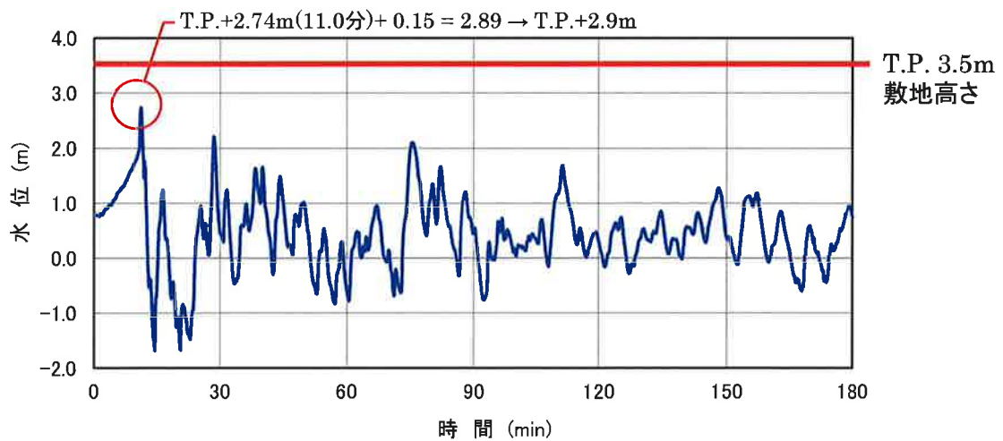
図-2-2-26 3,4号炉循環水ポンプ室 津波波形
