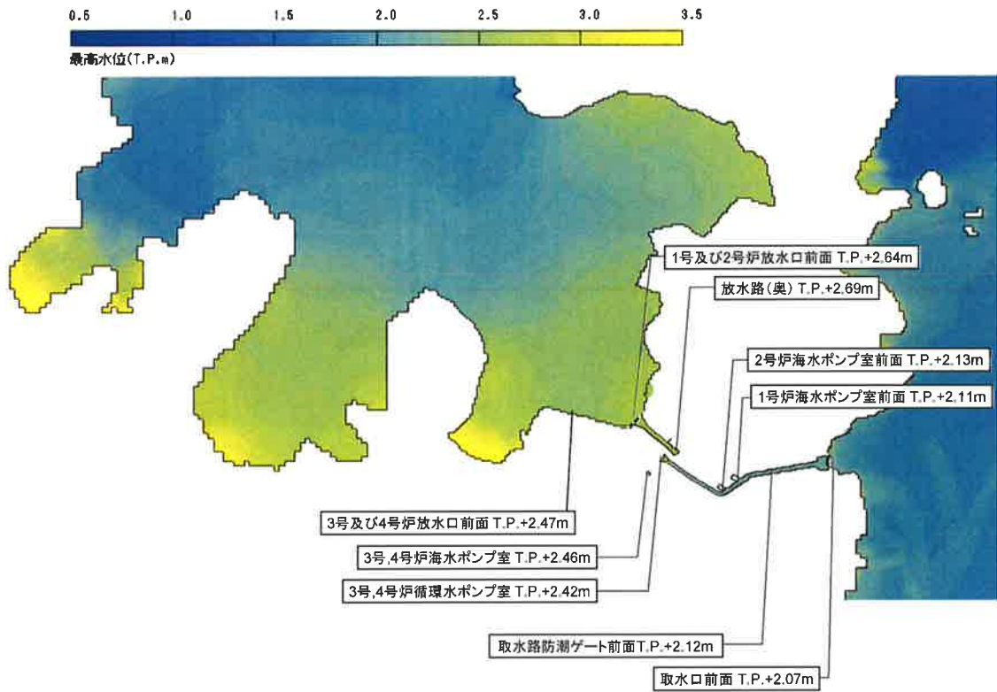
図-2-2-2 津波対策を踏まえた津波最高水位分布 (2)
