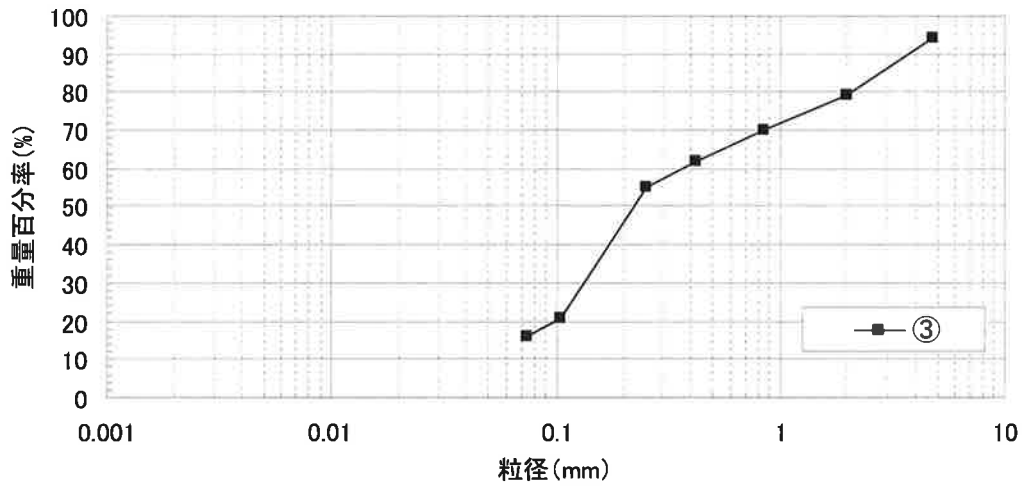
図-2-5-7 粒径加積曲線 (調査地点③)
