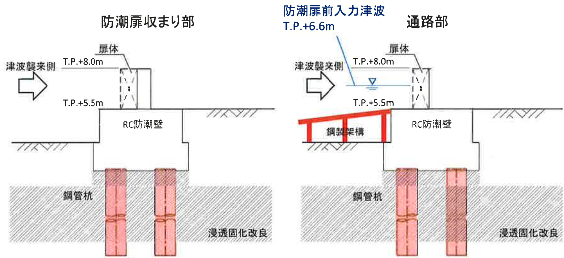
図-2-2-46 防潮扉断面図
