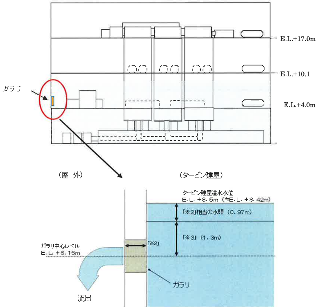
図-2-4-10 タービン建屋溢水水位イメージ
