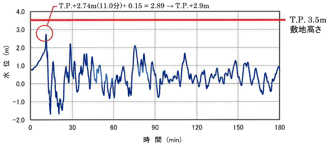
図-2-2-40 3,4号炉循環水ポンプ室 津波波形
