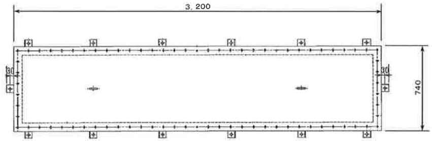
浸水防止蓋 2
