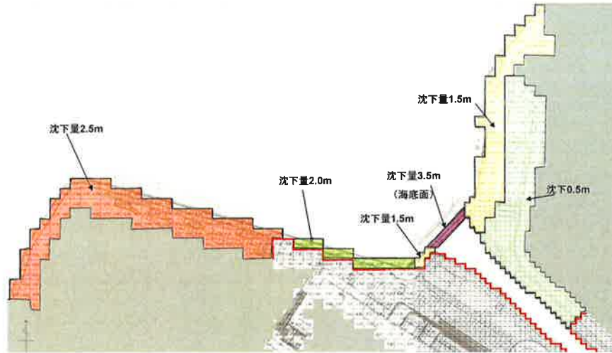
図-1-3-1 現地盤からの沈下量想定
