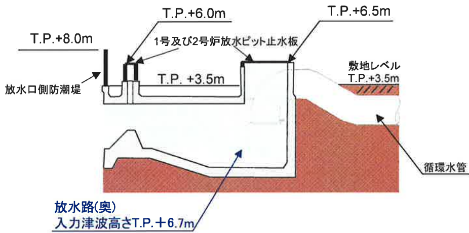
図-2-2-48 1号及び2号炉 放水ピット断面図
