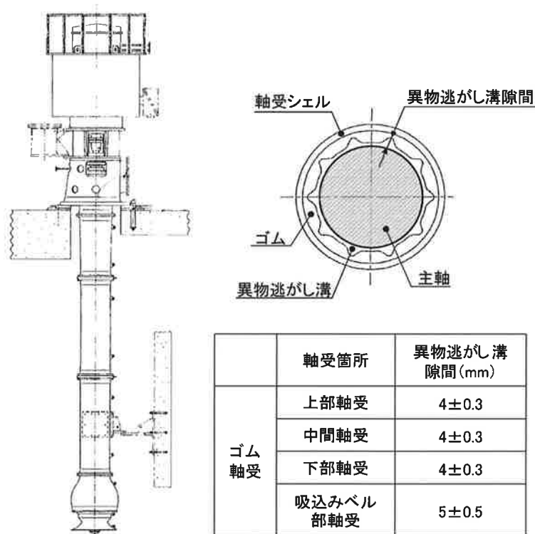
図-2-5-3(1/2) 海水ポンプ軸受構造図 (1号炉及び2号炉)
