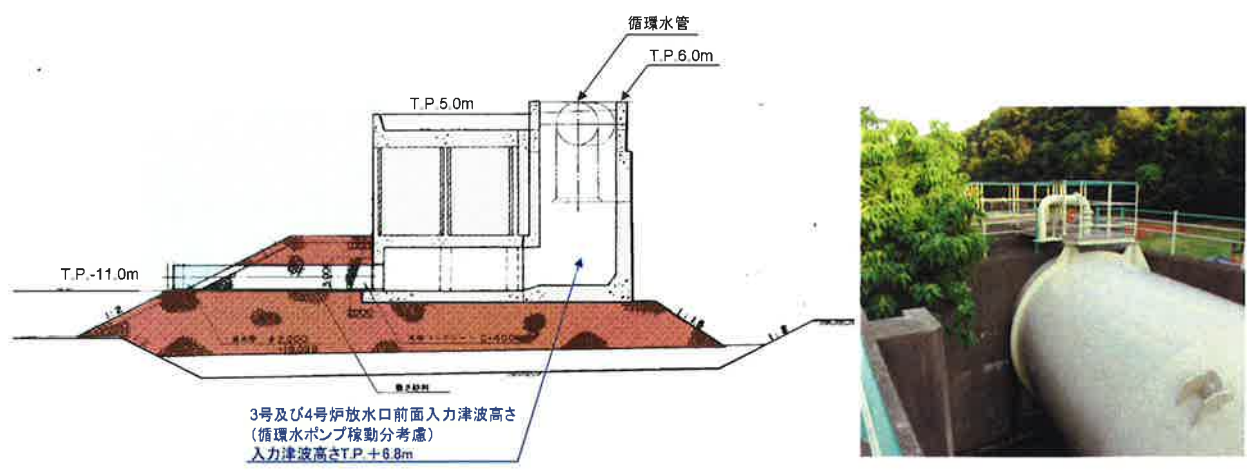
図-2-2-52 3号及び4号炉 放水路断面図
