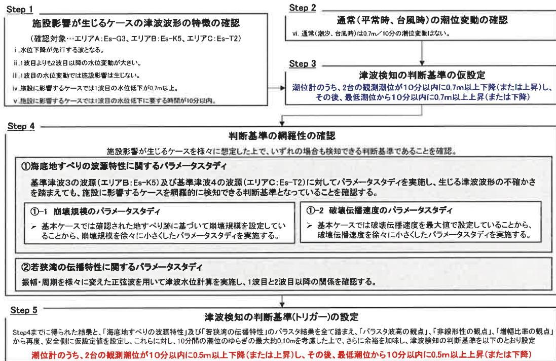
図-1-4-2 閉止判断基準の設定フロー
