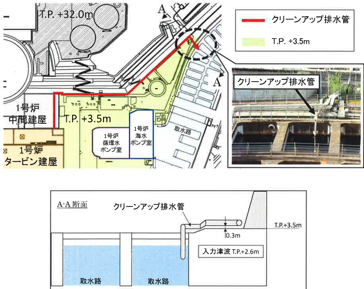
図-2-2-36 1号炉海水ポンプ室付近排水管経路図
