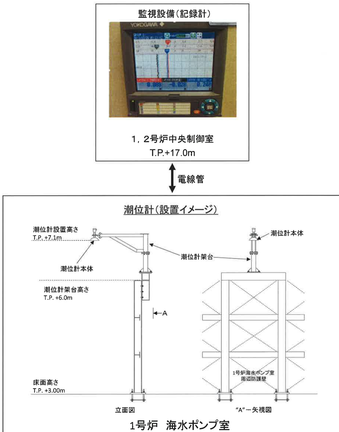
図 3-3-5 (1/2) 潮位計設備構成イメージ
