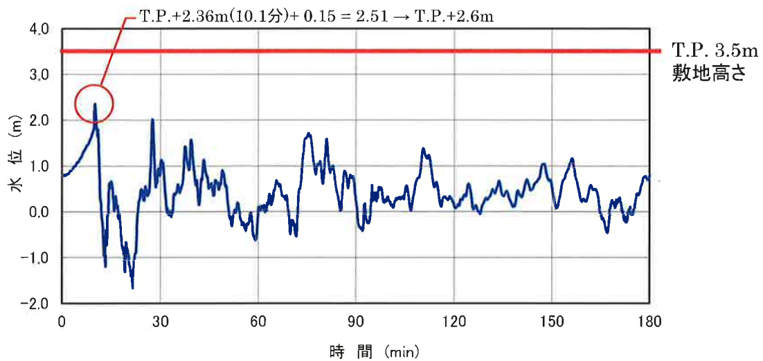
図-2-2-37 1号炉海水ポンプ室 津波波形
