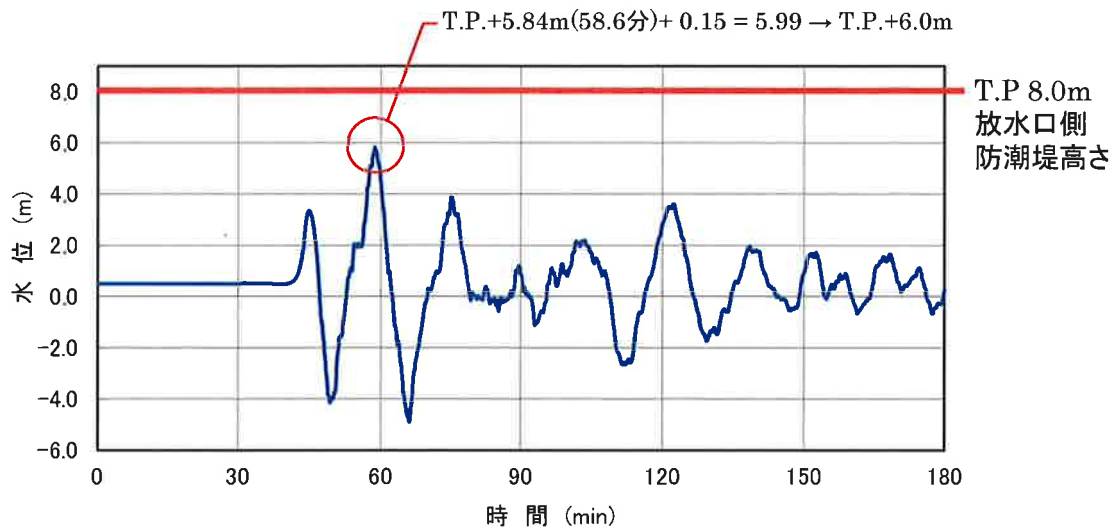
図-2-2-53 3号及び4号炉 放水口前面津波波形
