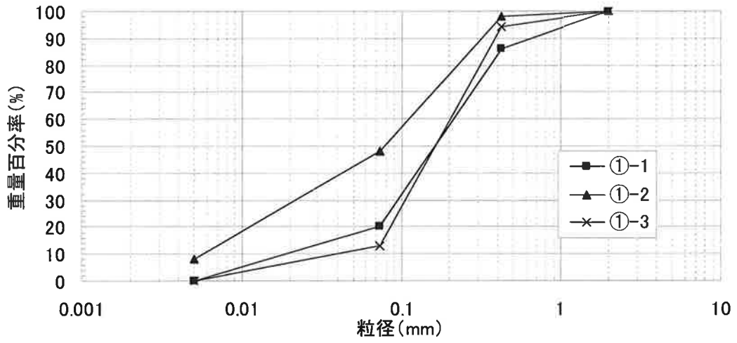
図-2-5-5 粒径加積曲線 (調査地点①-1~3)
