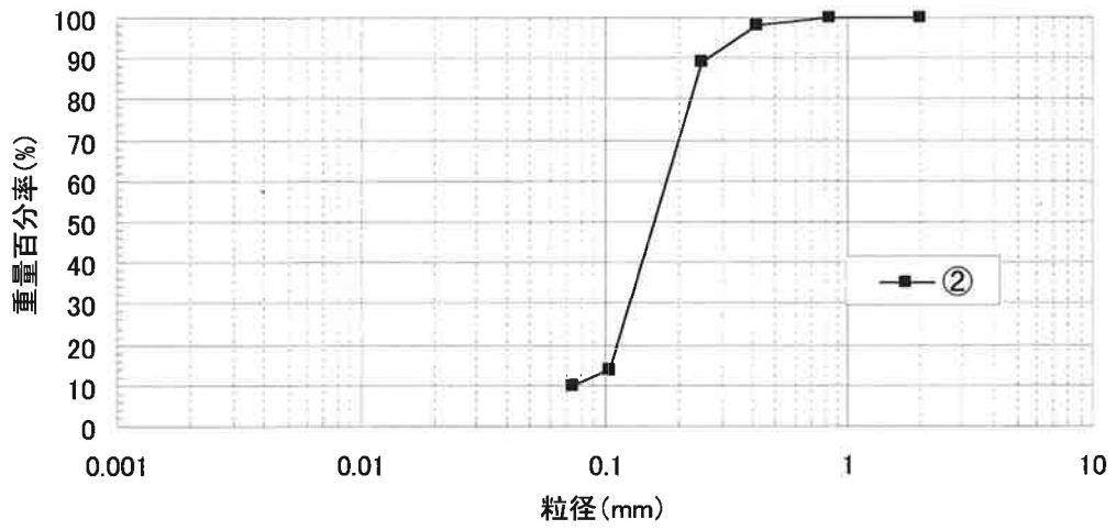
図-2-5-6 粒径加積曲線 (調査地点②)
