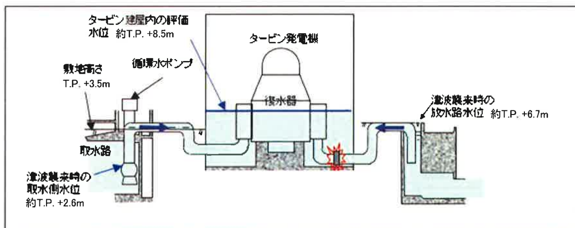
図-2-4-11 タービン建屋内の評価水位と取水側水位及び放水ピット側水位の概略図
