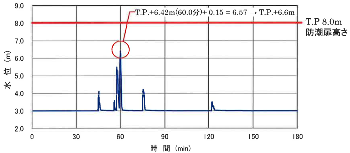
図-2-2-47 防潮扉前 津波波形
