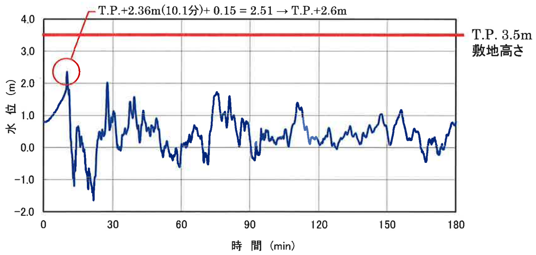
図-2-2-12 1号炉海水ポンプ室 津波波形
