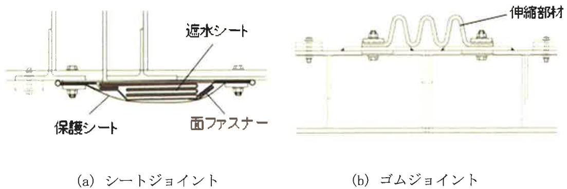
図-3-1-9 止水ジョイント詳細図
