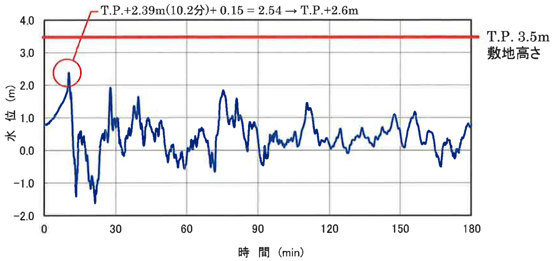
図-2-2-39 2号炉海水ポンプ室 津波波形
