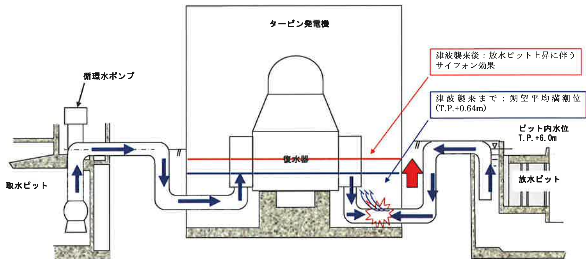
図-2-4-21 津波の流入イメージ
