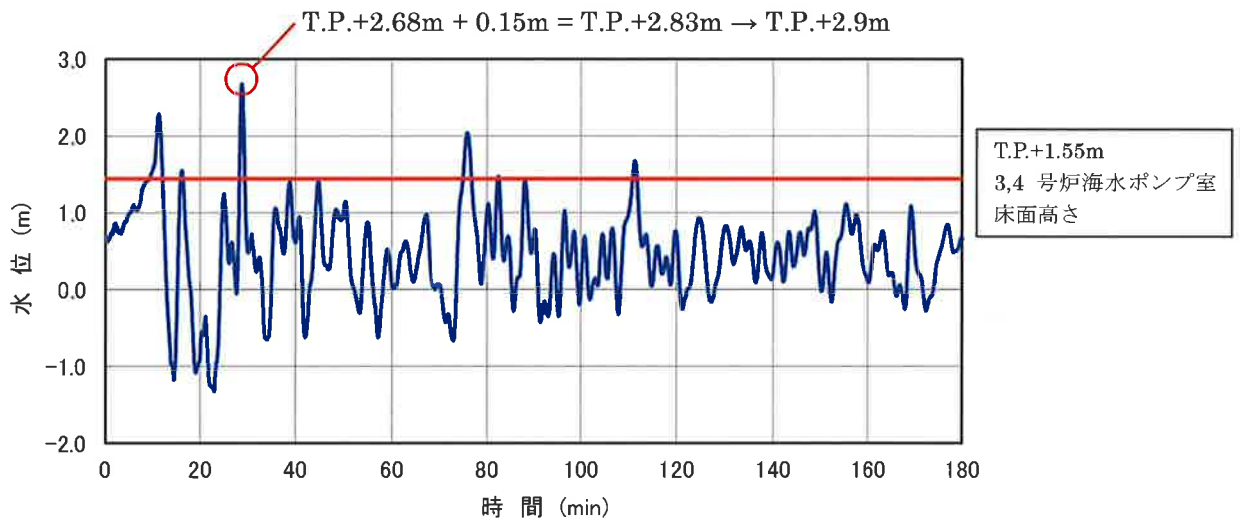
図-2-2-28 3,4号炉海水ポンプ室 津波波形
