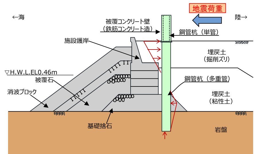
荷重図
