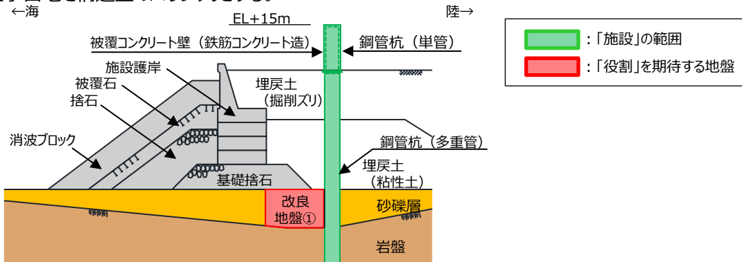
防波壁（多重鋼管杭式擁壁）（改良地盤部）における「施設」と「地盤」の区分
