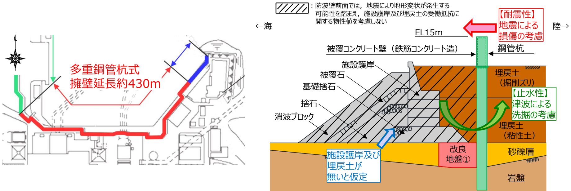
検討概要図
