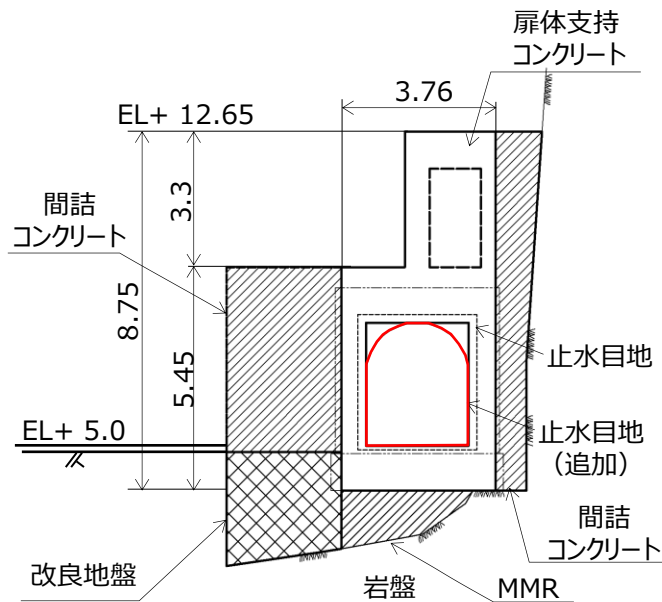
A-A 断面 (取り合い部)
