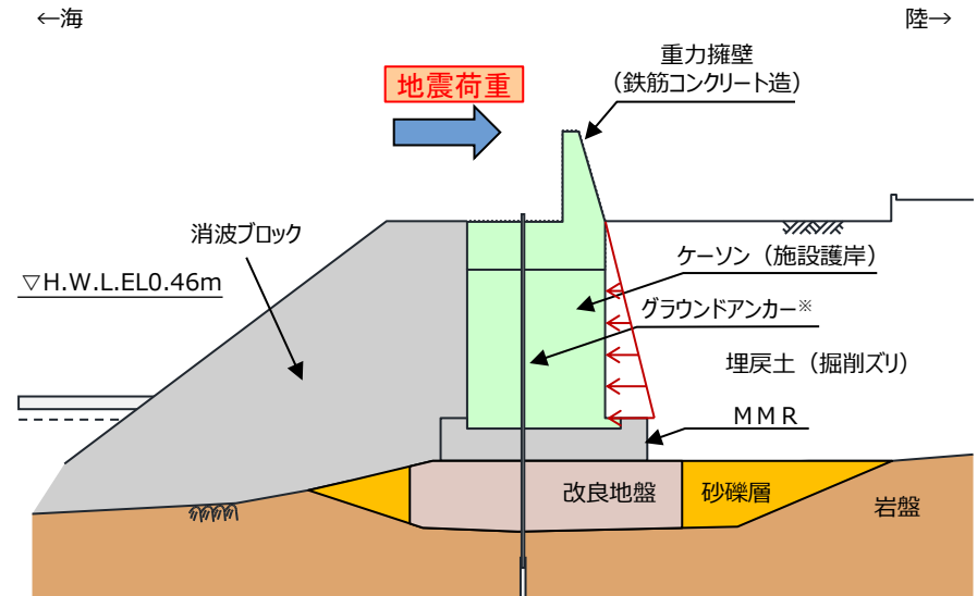
荷重図
