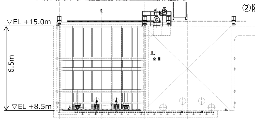
②防波壁通路防波扉（1，2号炉北側） 正面図
