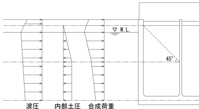
側壁（前壁）に生じる作用イメージ図 （陸側への作用）
