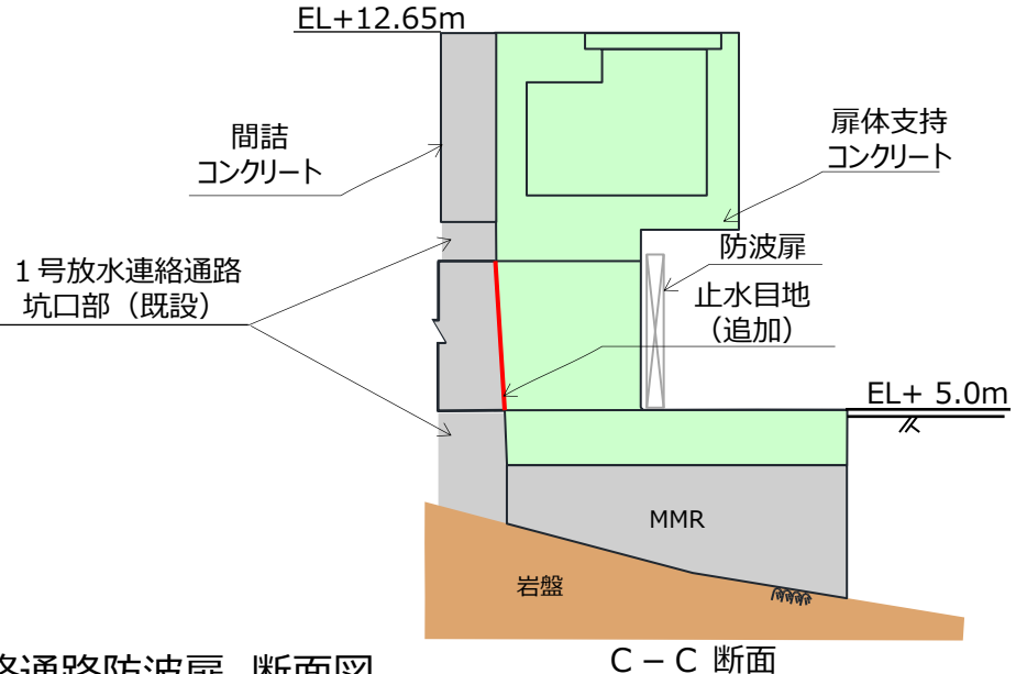
1号放水連絡通路防波扉 断面図
