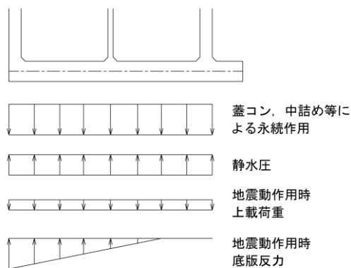
底版に生じる作用イメージ図 （地震動作用時）
