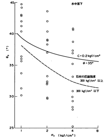
φ 0 と拘束圧の関係
