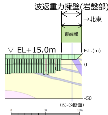
防波壁（波返重力擁壁）岩相縦断図
