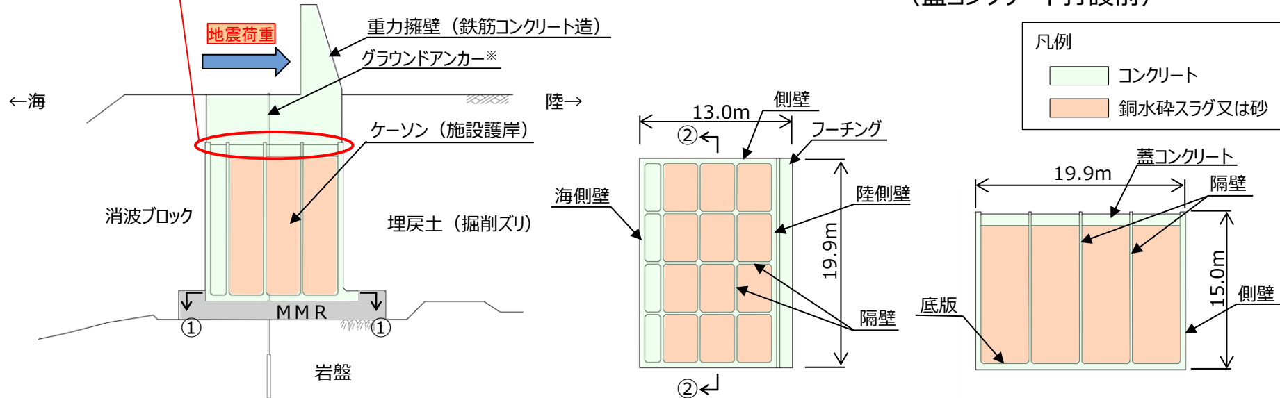
ケーソン構造図 (①-①断面) ケーソン構造図 (②-②断面)
