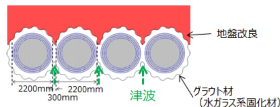
一般部 (① - ①断面)
