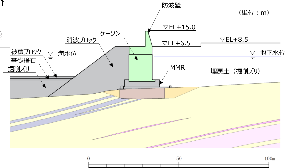
防波壁（波返重力擁壁）改良地盤部（②-②断面） 地質断面図
