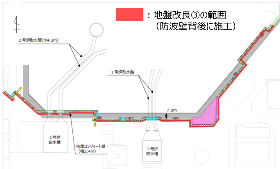
平面図
