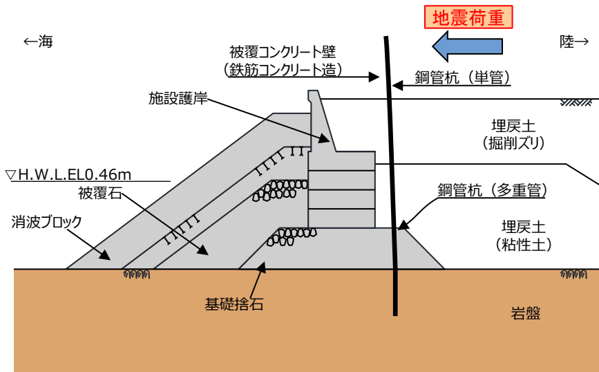
変形モード
