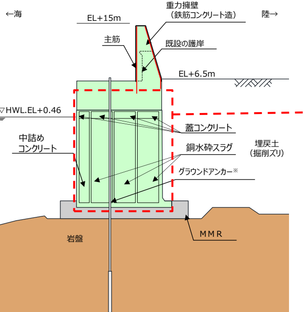
防波壁断面図（波返重力擁壁）
