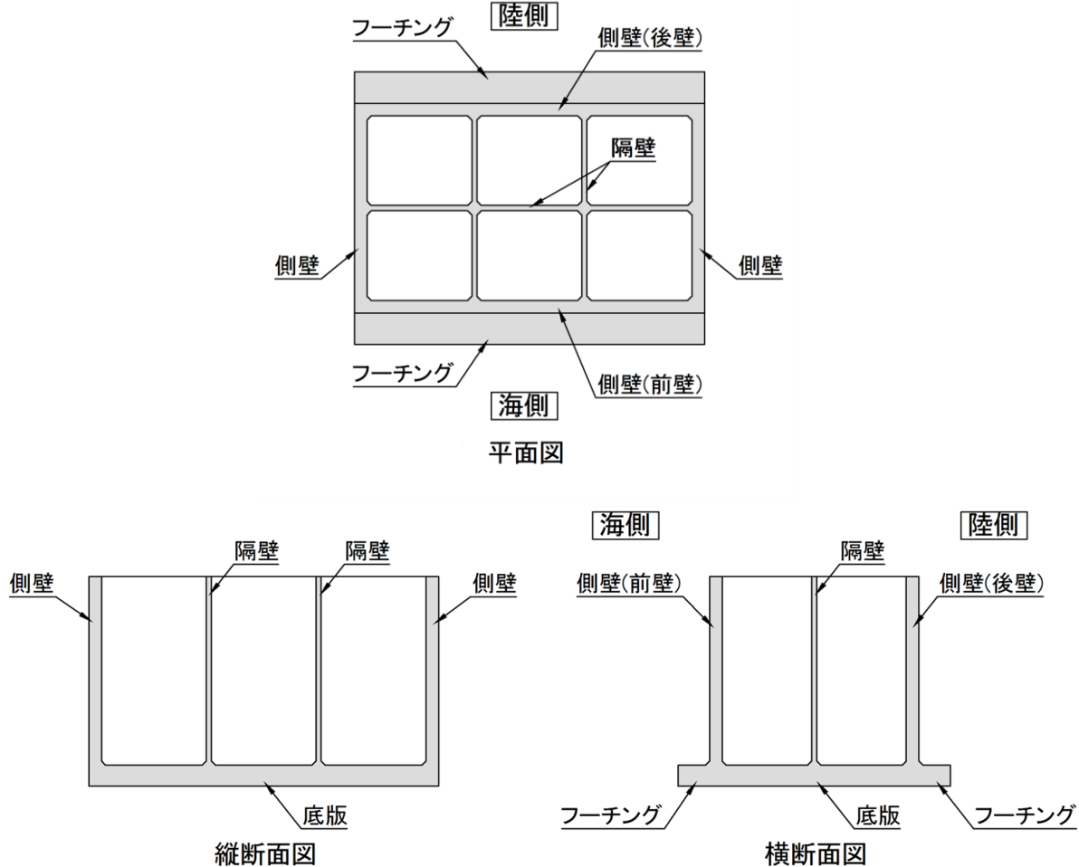
ケーソンの各部の名称 (港湾基準 図-参1.2.1を加筆・修正)
