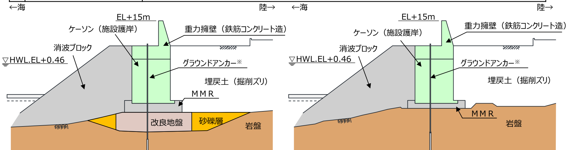
※ グラウンドアンカーの効果を期待しなくても、耐震・耐津波安全性を担保している。 防波壁（波返重力擁壁（岩盤部））断面図
