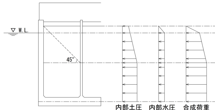
側壁（前壁）に生じる作用イメージ図 （海側への作用）
