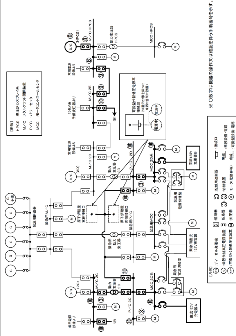
第 1.14.2.4-1 図 高圧炉心スプレィ系ディーゼル発電機による非常用 所内電気設備への給電手順の概要図
