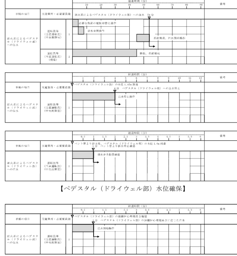
【原子炉圧力容器破損後のペDESTAL（ドライウエル部）への注水】 【ペDESTAL（ドライウエル部）水位確保】 第1.8-9図 消火系によるペDESTAL（ドライウエル部）への注水 タイムチャート
