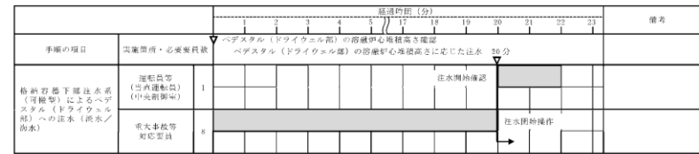
第1.8-7図 格納容器下部注水系(可搬型)によるペDESTAL(ドライウェル部)への注水(淡水/海水) タイムチャート
