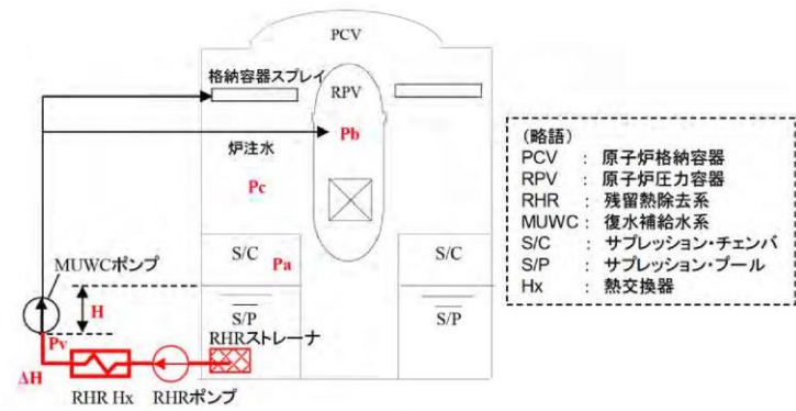
図2 NPSH 評価条件図
