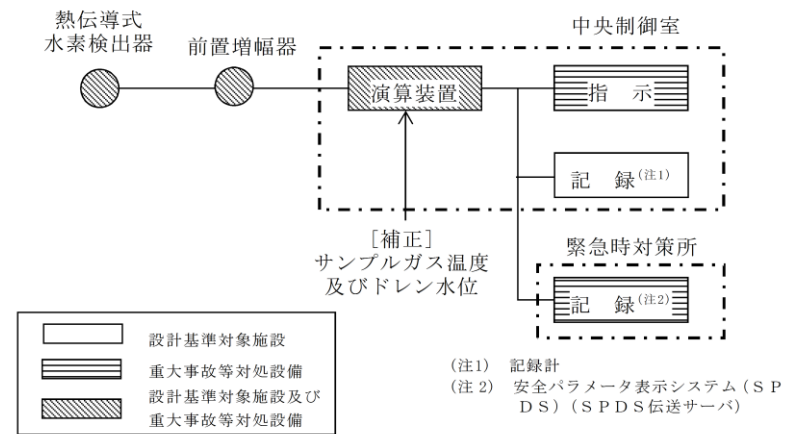
図6 格納容器水素濃度の概略構成図
