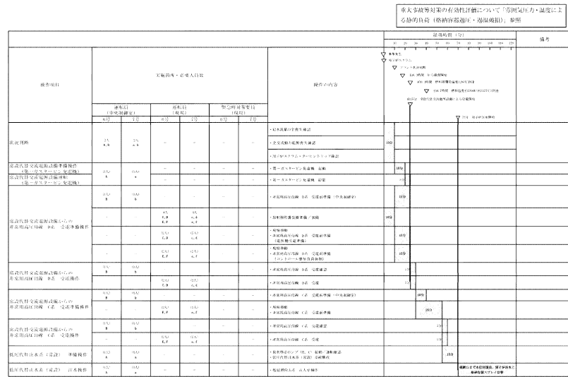
図 2.2.2-4 代替循環冷却系運転の作業と所要時間(0~320分後) 「雰囲気圧力・温度による静的負荷(格納容器過圧・過温破損)の場合」
