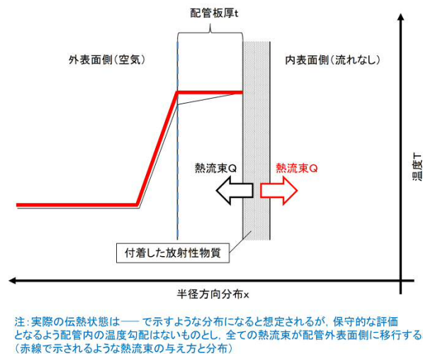
図3 配管内表面の温度評価 (ケース2のイメージ)
