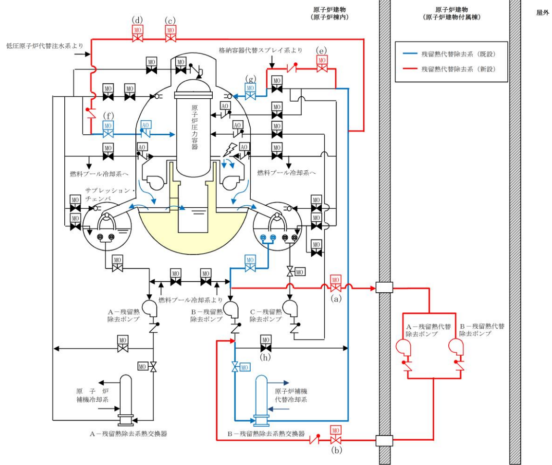
図 2.2.1-1 残留熱代替除去系概要図
