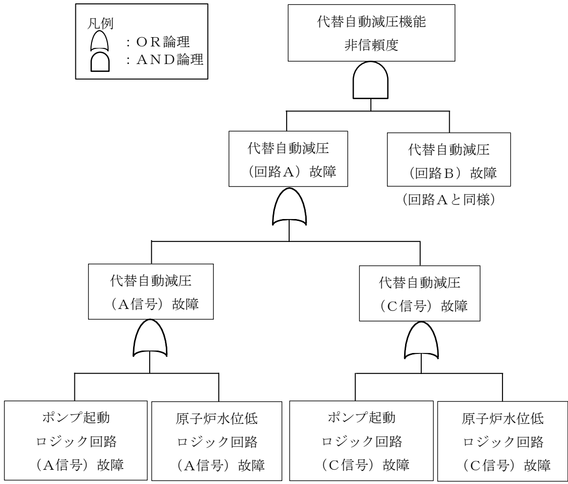
図4 非信頼度の評価に適用したフォールトツリー
