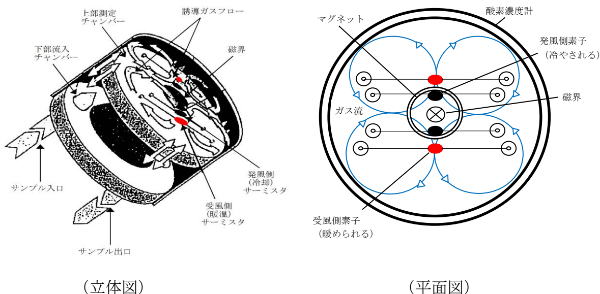
図7 酸素含有ガスの流れ
