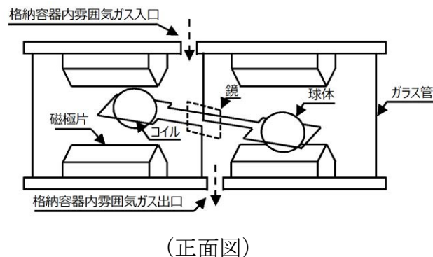
図3 格納容器酸素濃度 (S A) の概要図
