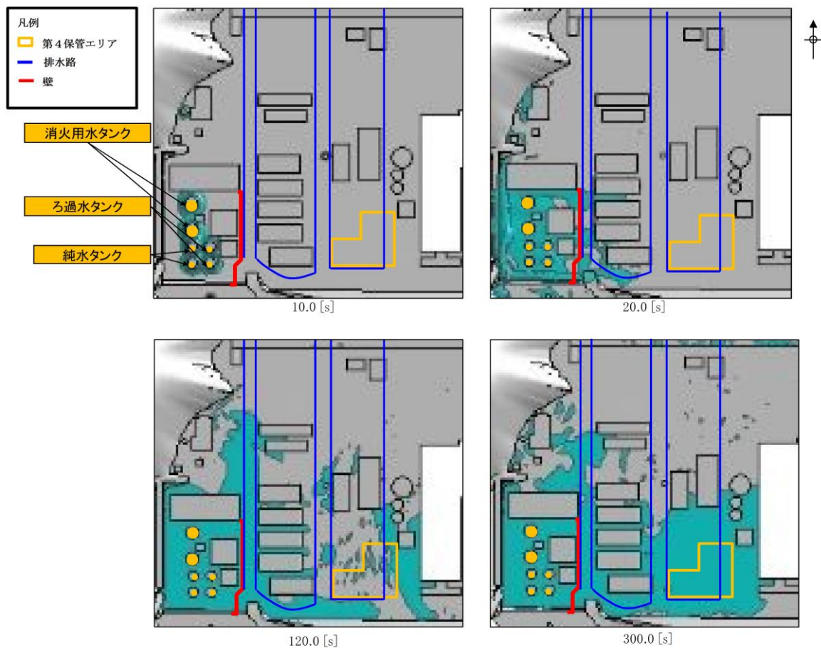
第13図 第4保管エリア近傍の溢水の伝播挙動
