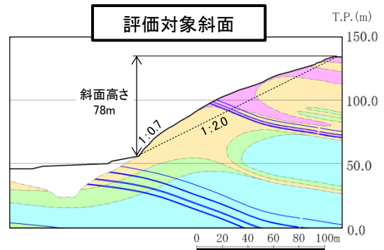
⑬-⑬' 断面
