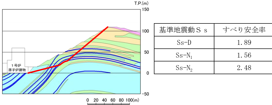
④-④' 断面
