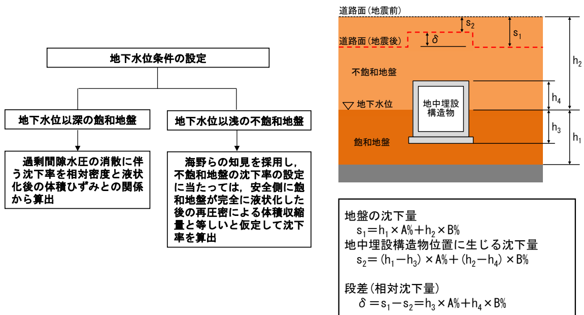
第3-6 図 不飽和地盤及び飽和地盤の沈下量算出フロー
