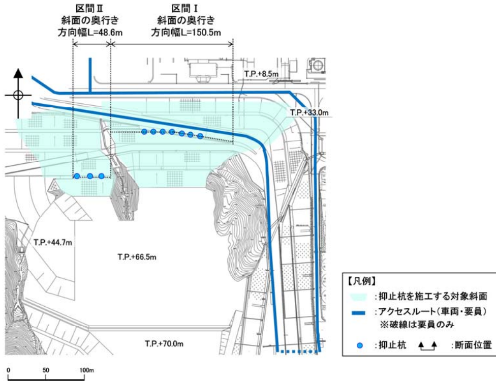
平面図
