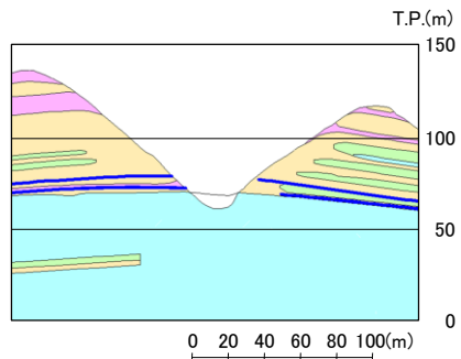
第 4.3-6 図 ⑭-⑭' 断面 解析モデル図
