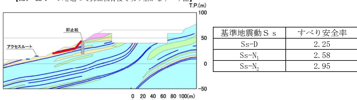
【B21・22 シームを通過して法面に抜けるすべり面】
