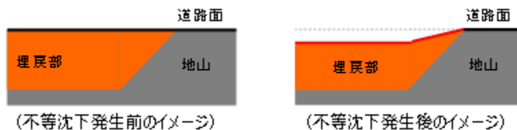
第 4-17 図 地山と埋戻部との境界部の状況
