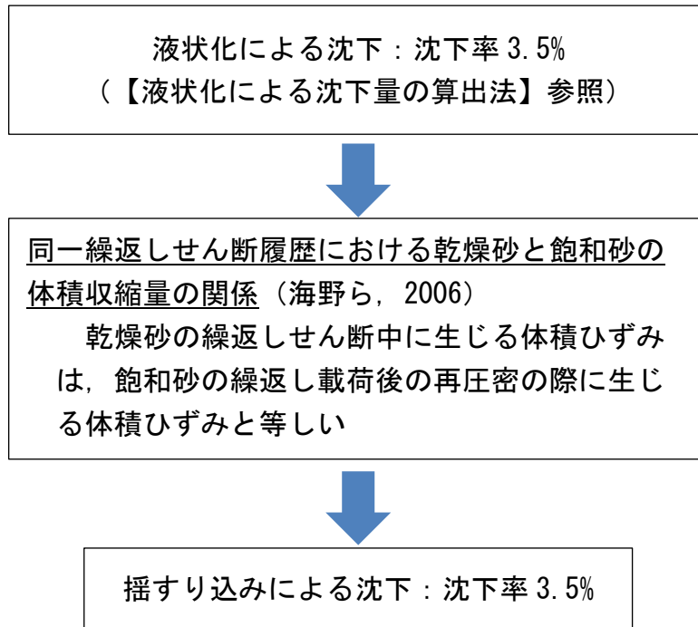
第3-9図 不飽和地盤の揺すり込み沈下率
