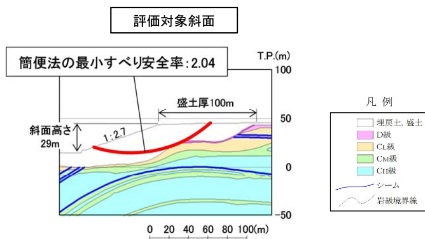
第5図 ⑧-⑧'断面の比較結果
