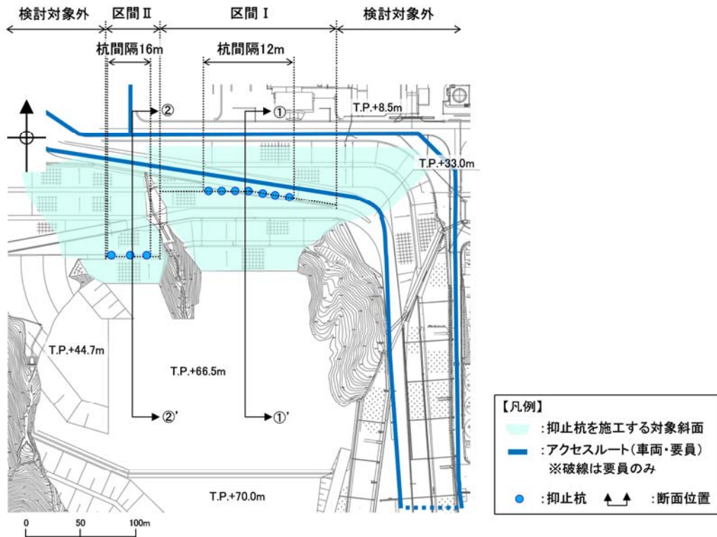
平面図
