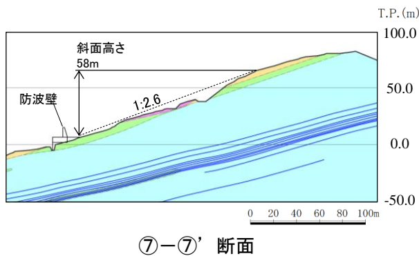
第3.2-3 図 グループA (T.P.+15m程度)の斜面の地質断面図(岩盤斜面)
