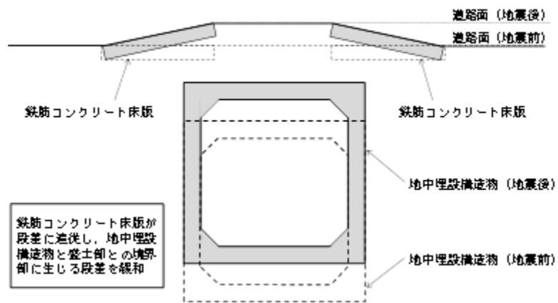
第 4-16 図 段差緩和対策例 (浮き上がり後)
