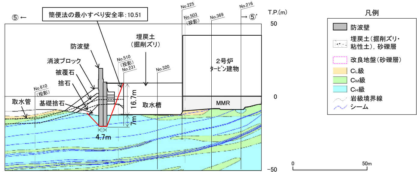
防波壁(多重鋼管杭式擁壁) ⑤-⑤'断面横断面図(岩級・シーム)
