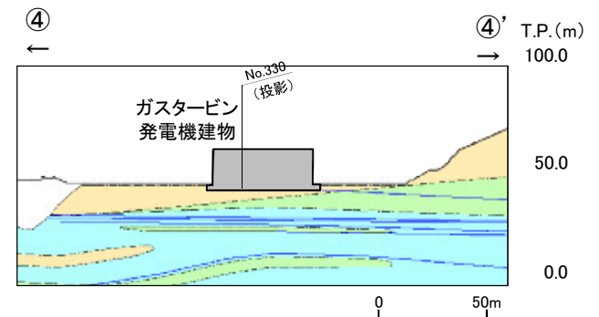
地質断面図(④-④'断面, 岩級・シーム)
