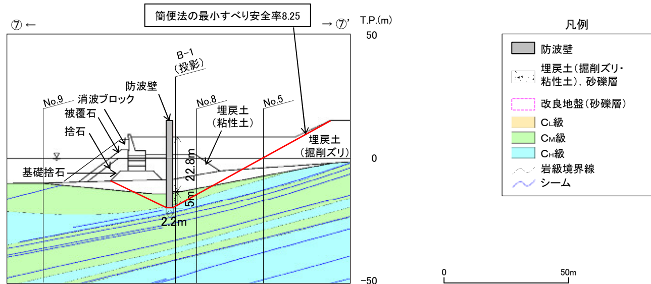
防波壁(多重鋼管杭式擁壁) ⑦-⑦'断面横断面図(岩級・シーム)
