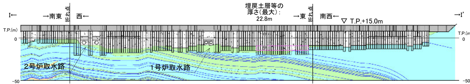
防波壁(多重鋼管杭式擁壁) 縦断面図(岩級・シーム)
