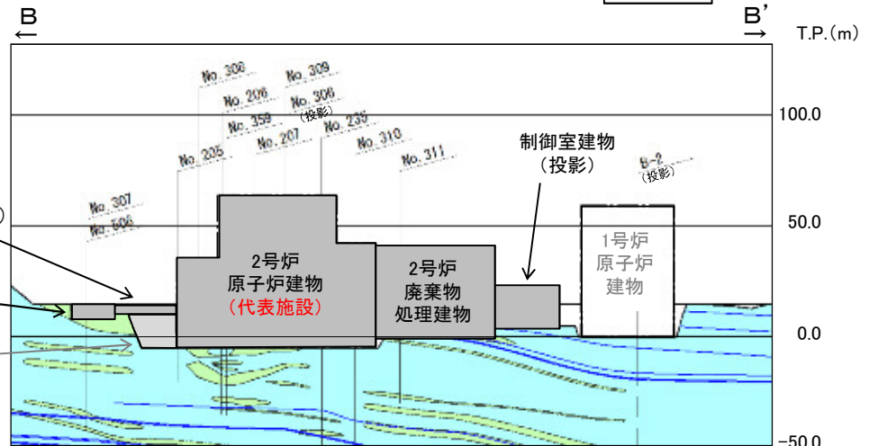
地質断面図(B-B'断面, 岩級・シーム)
