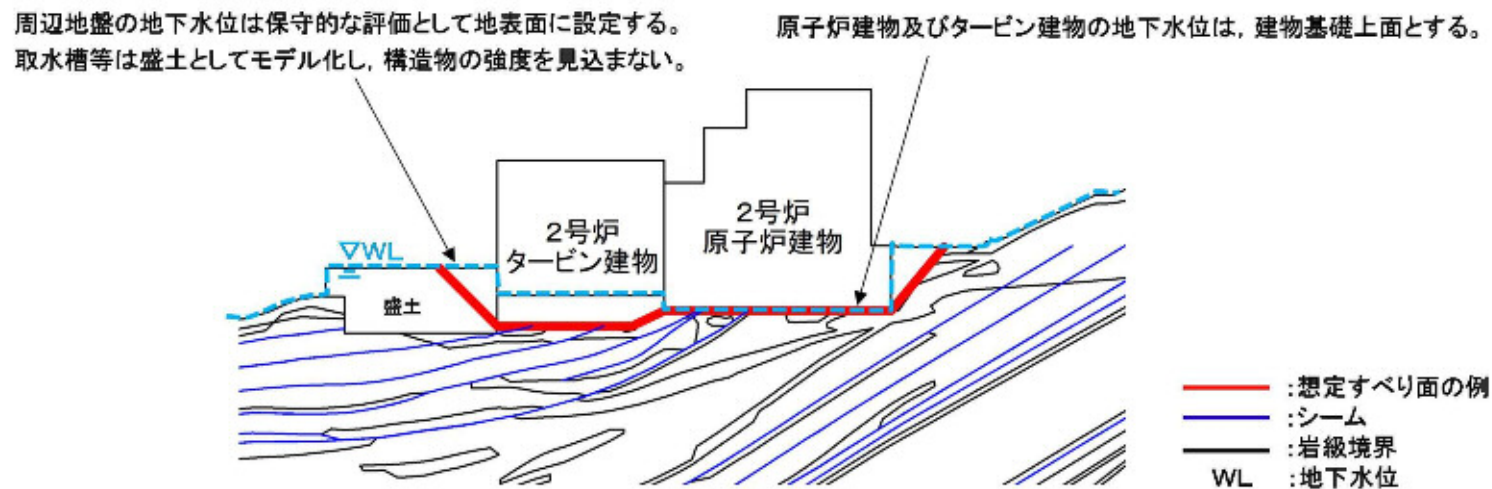
基礎地盤安定性評価における地下水位設定イメージ
