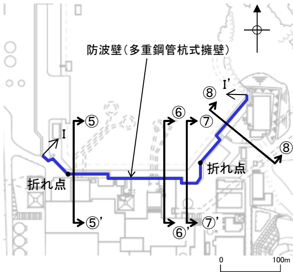
検討断面平面位置図
