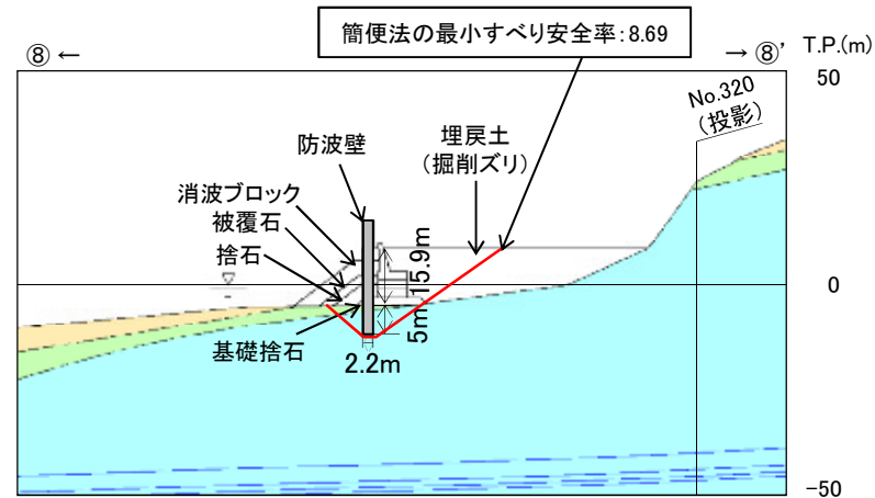
防波壁(多重鋼管杭式擁壁) ⑧-⑧' 断面横断面図(岩級・シーム)
