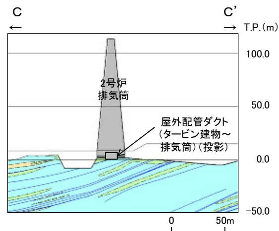
地質断面図(C-C'断面, 岩級・シーム)
