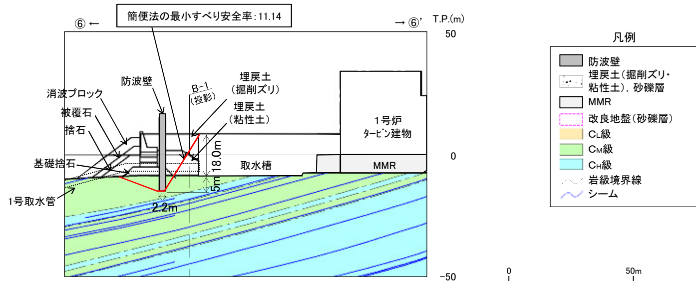
防波壁(多重鋼管杭式擁壁) ⑥-⑥'断面横断面図(岩級・シーム)
