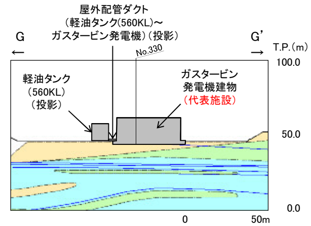
地質断面図(G-G'断面, 岩級・シーム)
