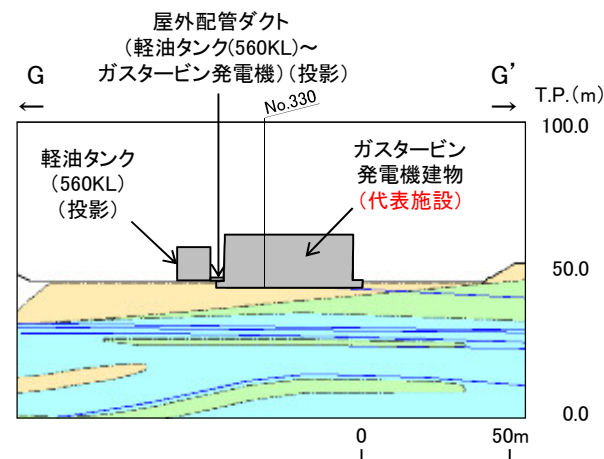
地質断面図(G-G'断面, 岩級・シーム)
