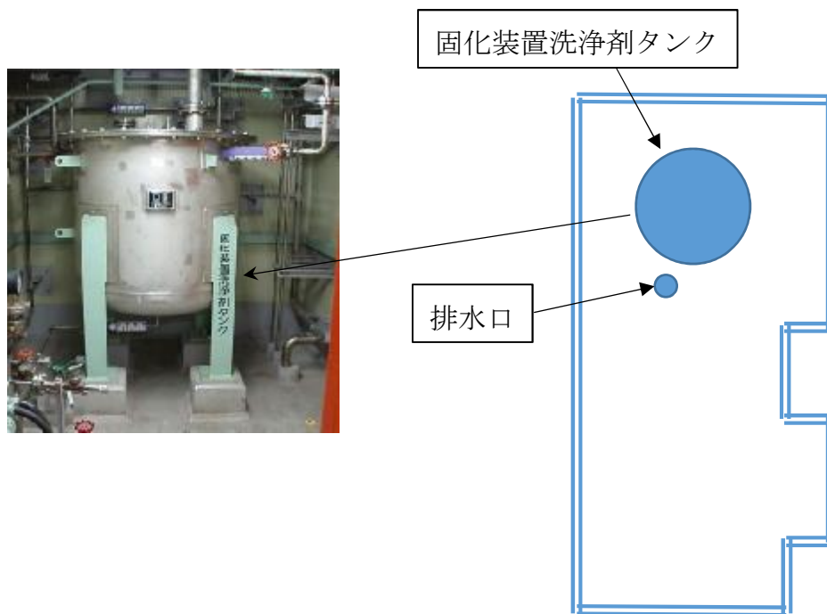
図4 1・2号機 固化装置洗淨剤タンク
