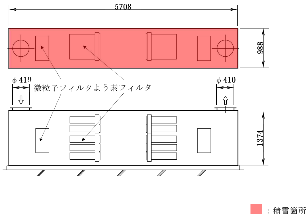
第6-1図 外形図（緊急時対策所非常用空気浄化フィルタユニット）
