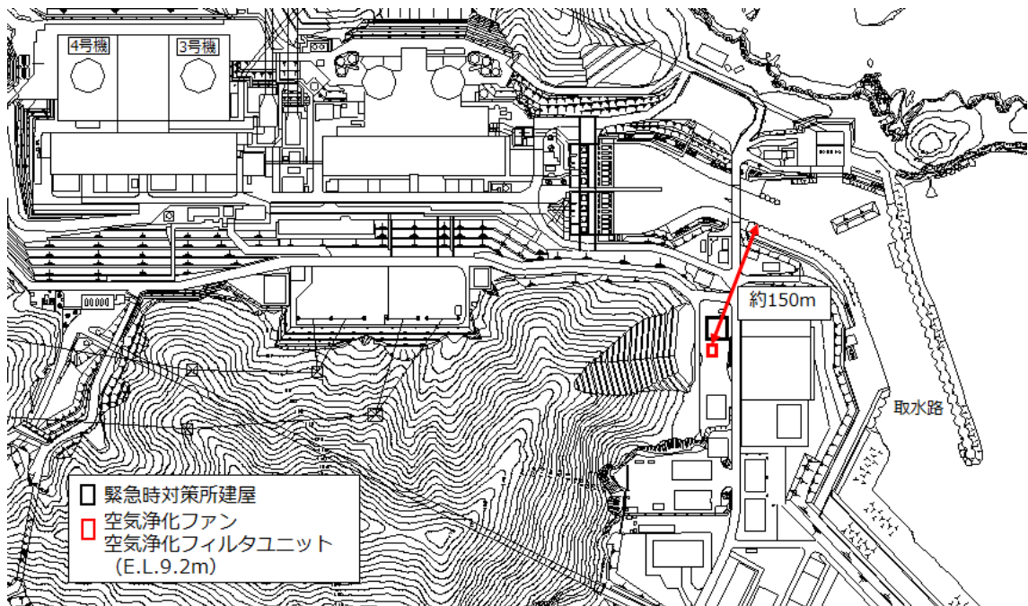
第6図 空気浄化ファン及び空気浄化フィルタユニットの設置場所
