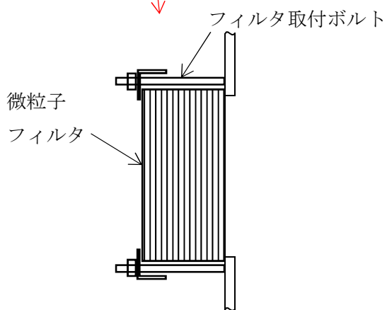
第2-1図 微粒子フィルタ取付概要
