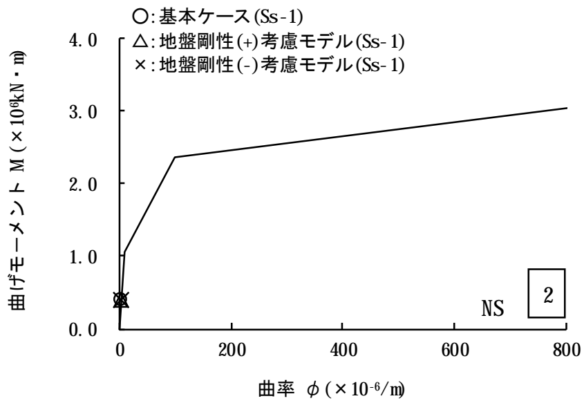
第2-13図 M- \phi 関係と最大応答値 (NS方向)
