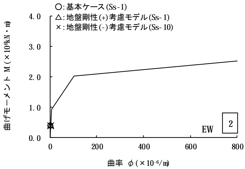
第2-15図 M- \phi 関係と最大応答値 (EW方向)
