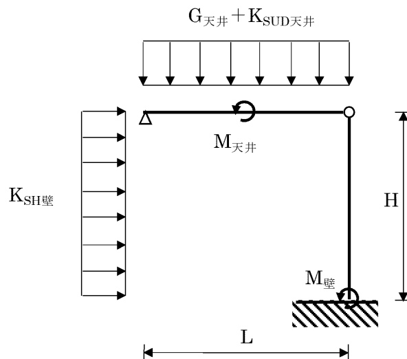
第 3-1 図 応力模式図 (曲げモーメント)
