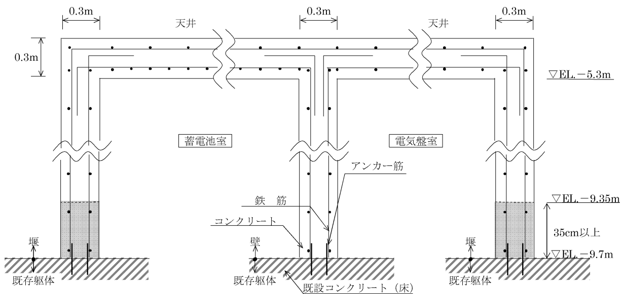
第 2-2 図 概略断面図 (A-A 断面)
