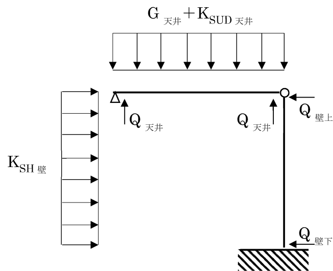
第3-2図 応力模式図 (せん断力)
