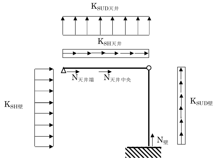
第 3-3 図 応力模式図 (軸力)
