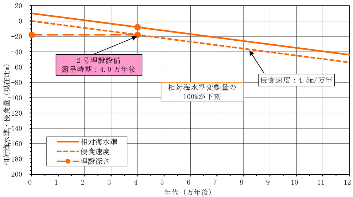
第 13 図 温暖期継続ケース厳しい設定における侵食量と施設露呈時期
