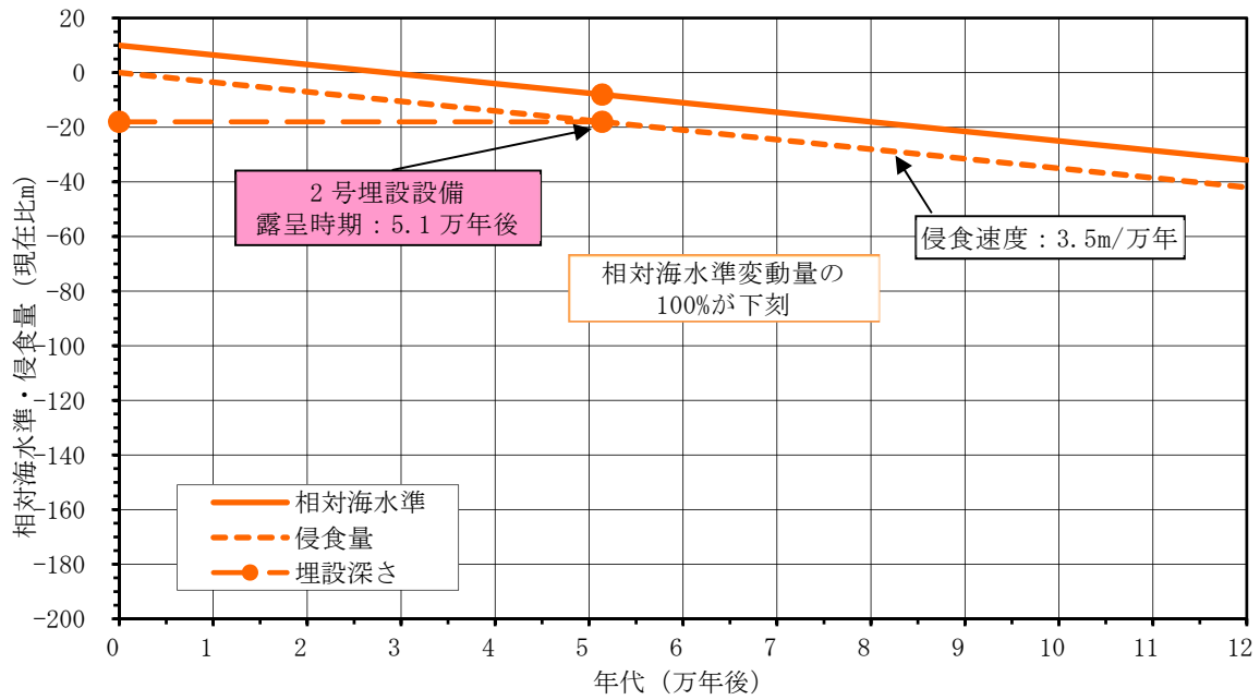
第 12 図 温暖期継続ケース確からしい設定における侵食量と施設露呈時期
