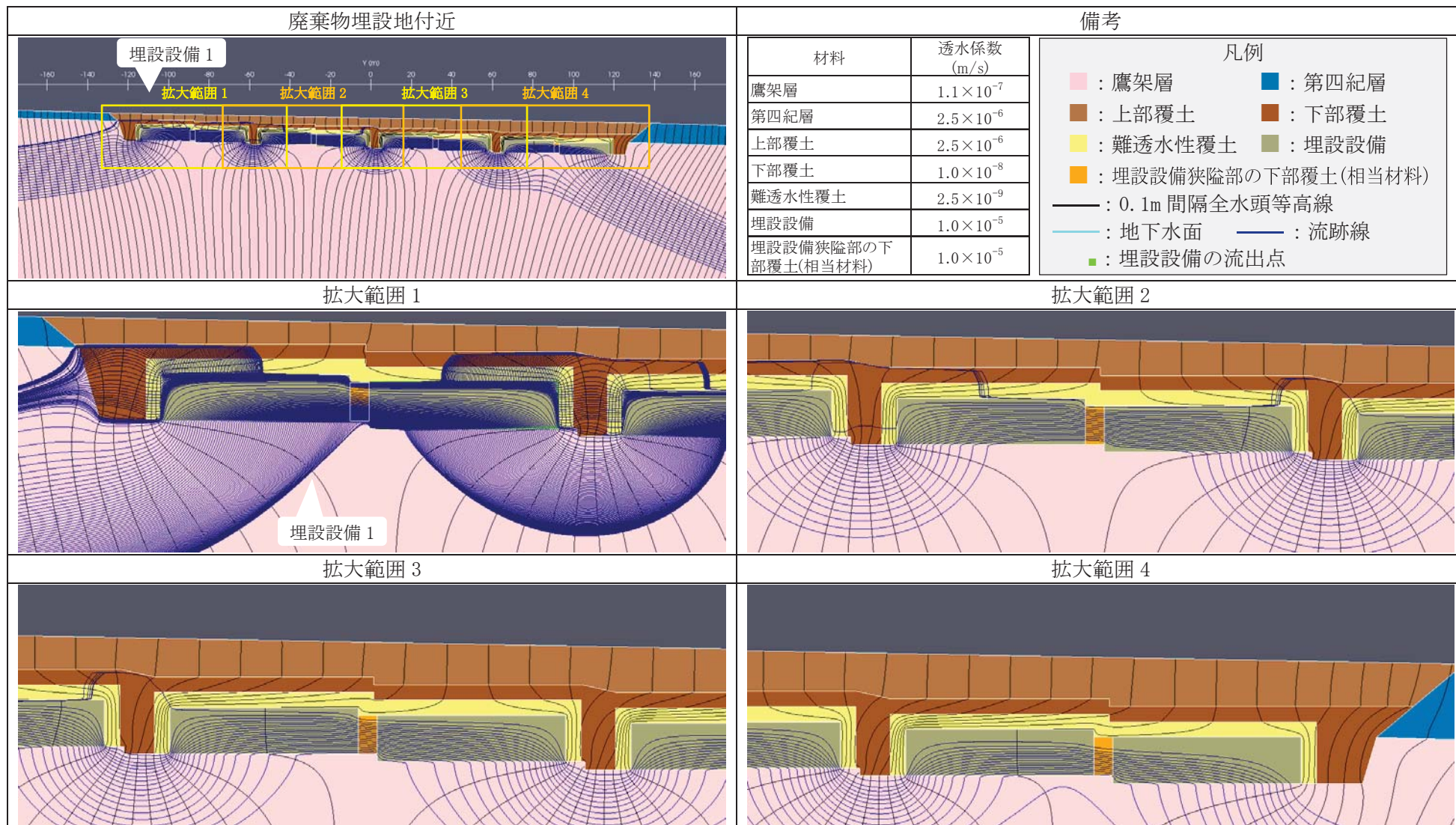
第1図 2次元地下水浸透流解析結果(確からしい設定 1,000年後) (2/9) <埋設設備1の流出点を通る流跡線>
