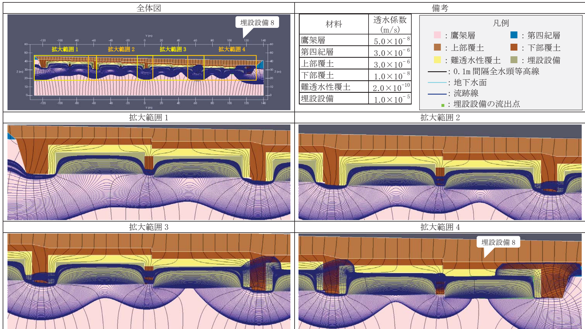
第9図 2次元地下水浸透流解析結果【1号廃棄物埋設地 水平方向】(確からしい設定 1,000年後) (9/9) <埋設設備8の流出点を通る流跡線>
