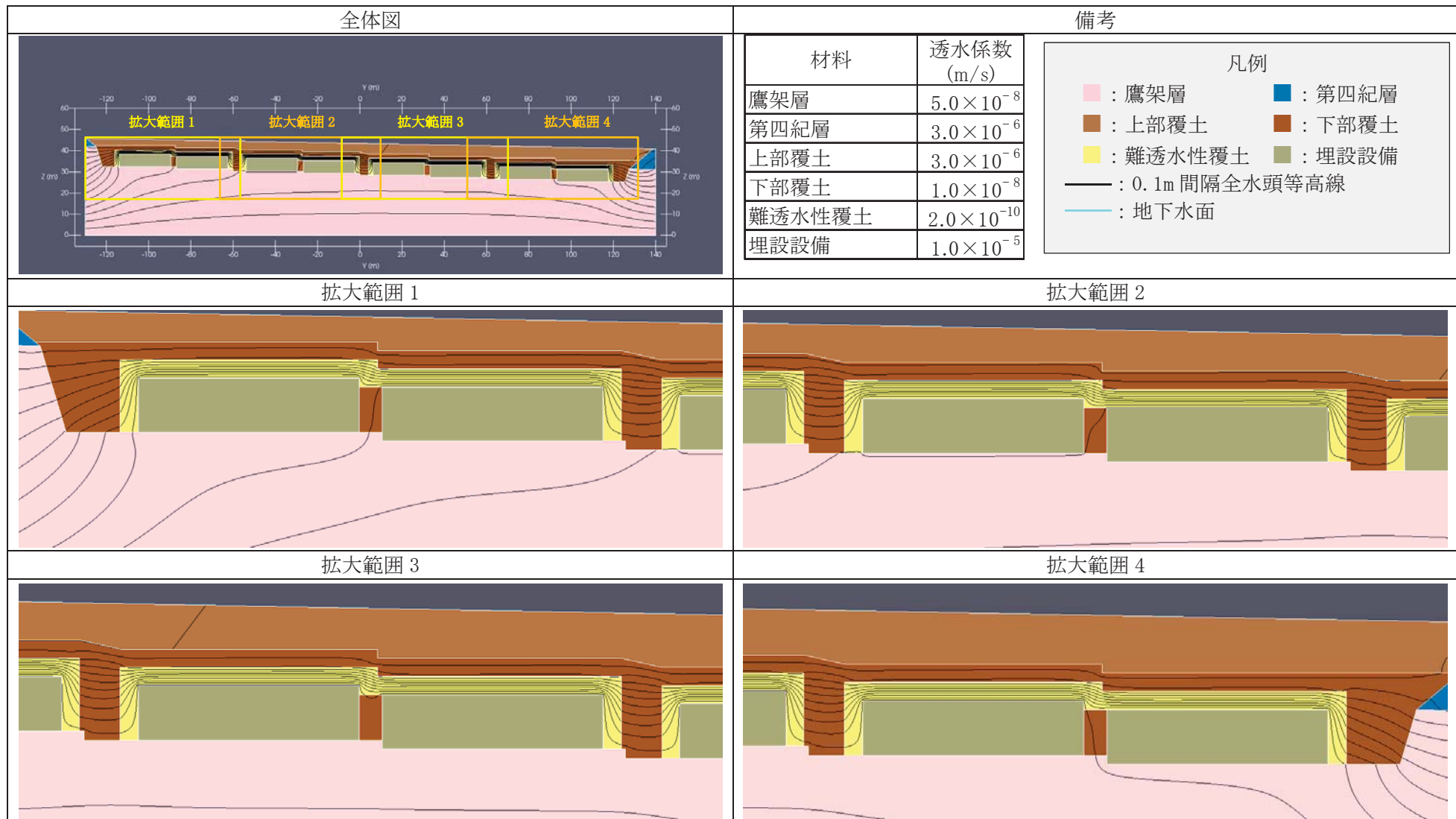
第 10 図 2 次元地下水浸透流解析結果【1 号廃棄物埋設地 鉛直下方】(確からしい設定 1,000 年後) (1/9) <0.1m 間隔全水頭等高線>
