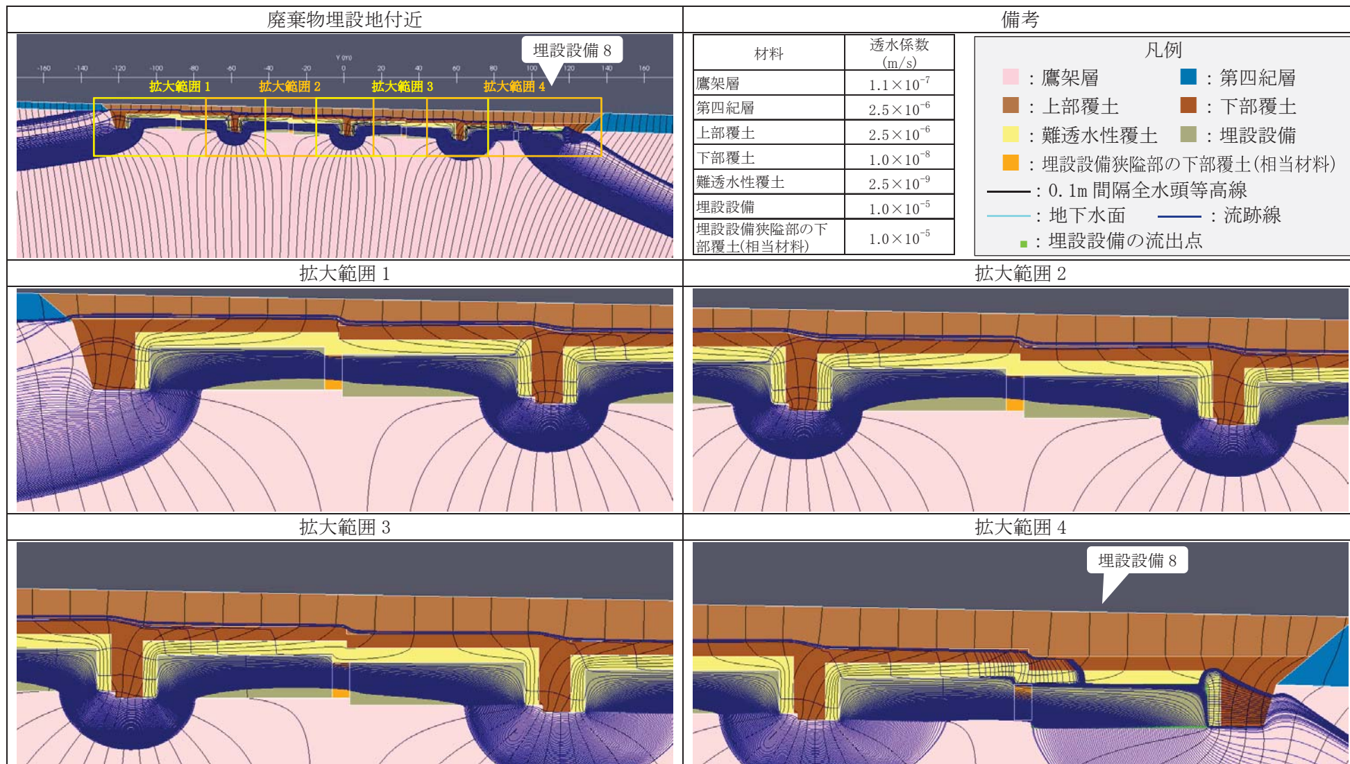
第1図 2次元地下水浸透流解析結果(確からしい設定 1,000年後) (9/9) <埋設設備8の流出点を通る流跡線>
