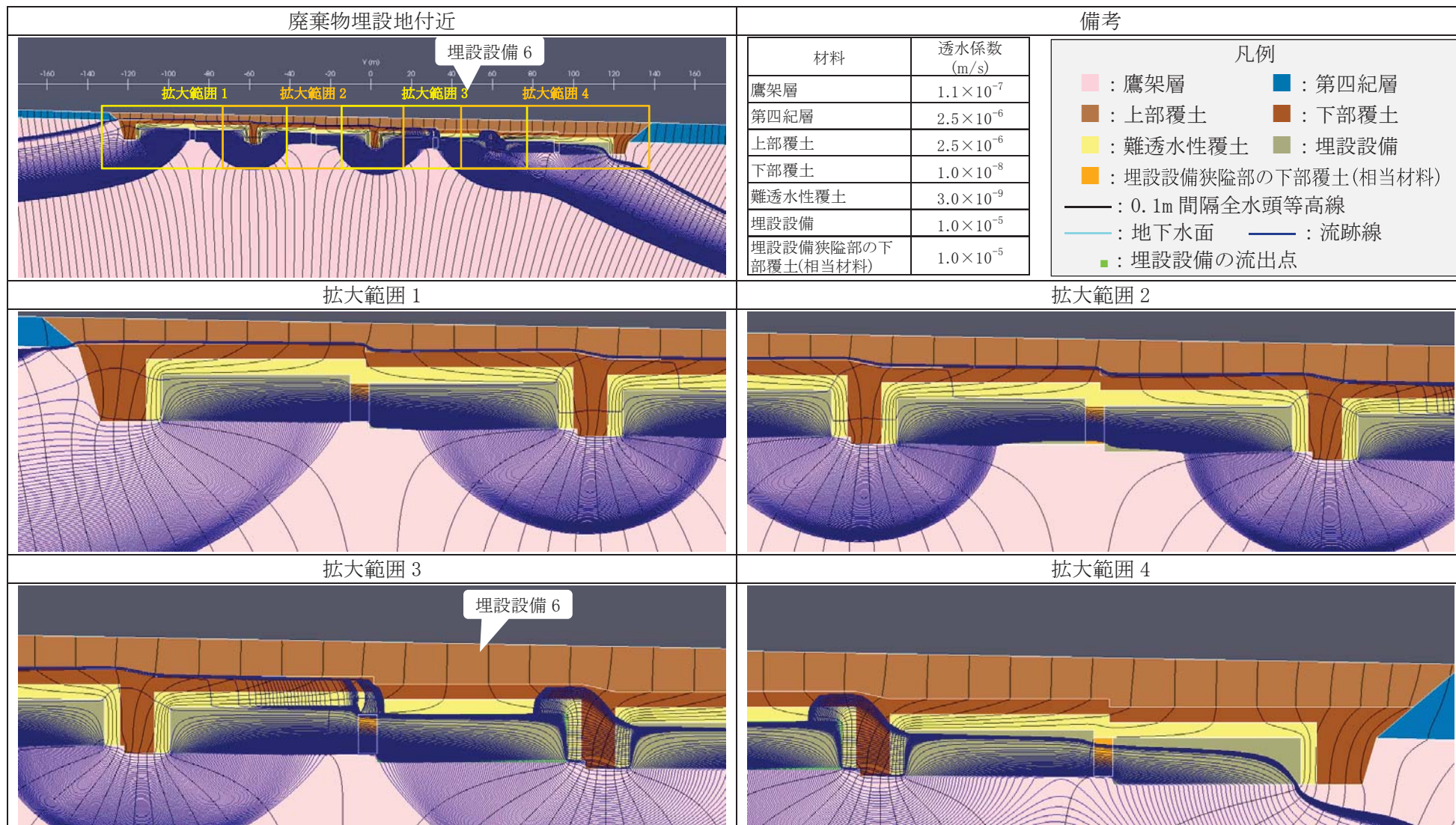
第2図 2次元地下水浸透流解析結果(厳しい設定 1,000年後) (7/9) <埋設設備6の流出点を通る流跡線>
