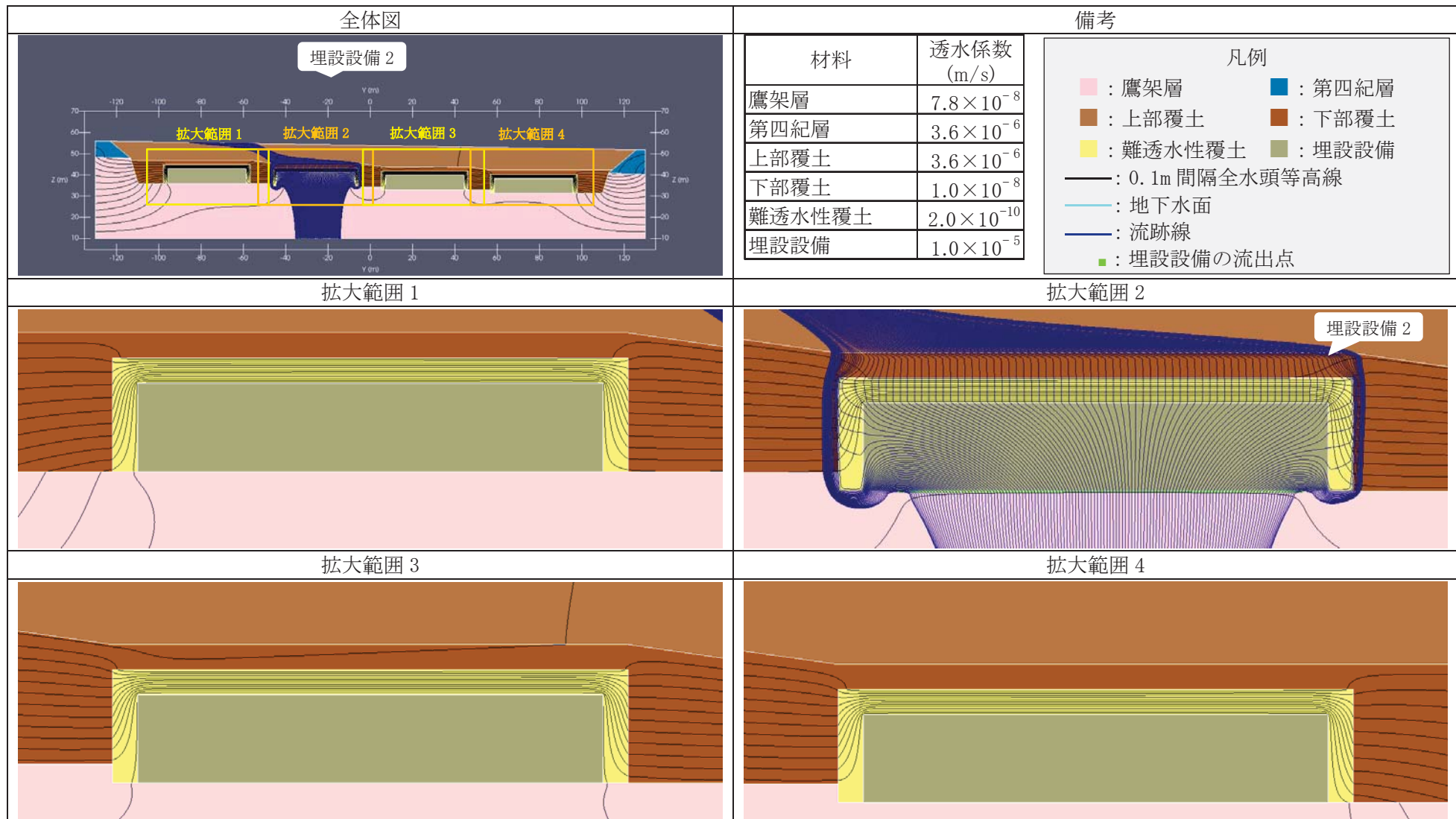
第 12 図 2 次元地下水浸透流解析結果【2 号廃棄物埋設地 鉛直下方】(確からしい設定 1,000 年後) (3/5) <埋設設備 2 の流出点を通る流跡線>
