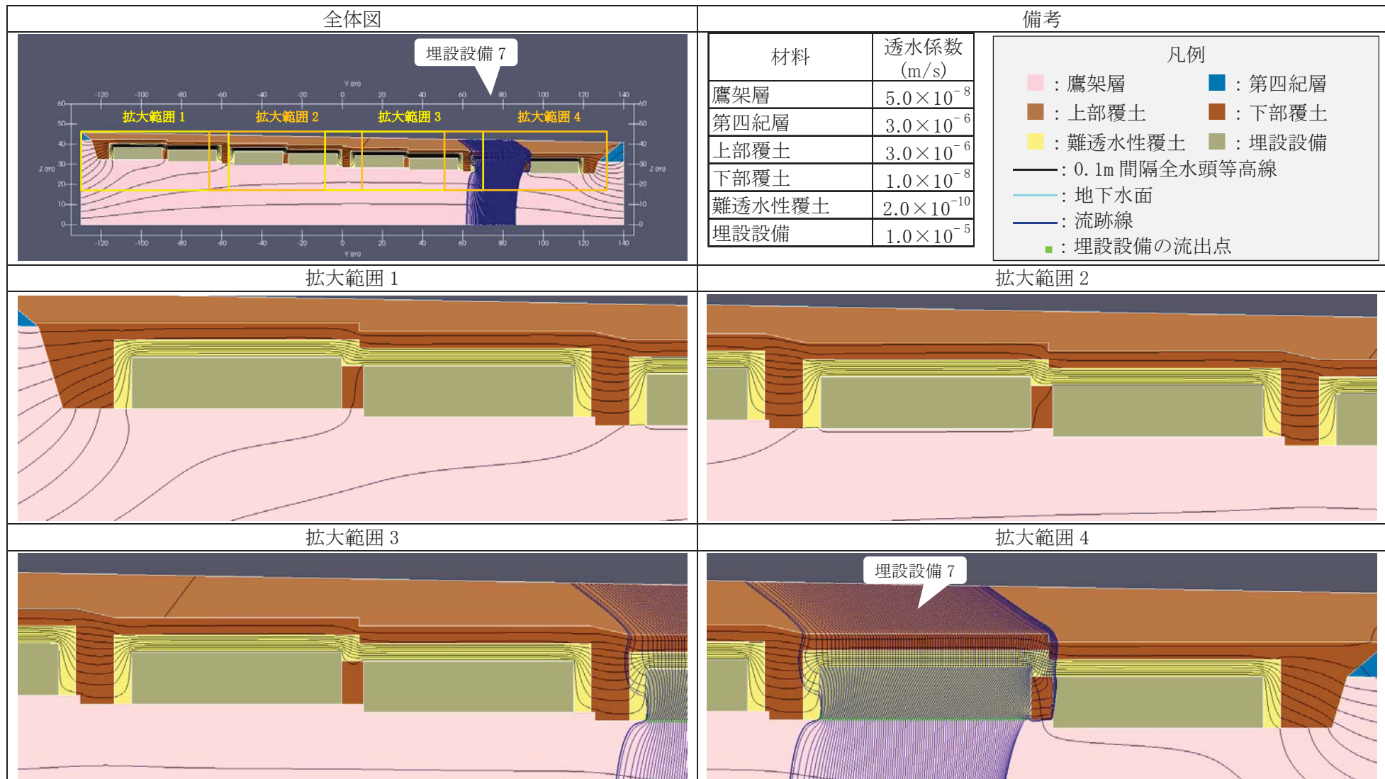
第 10 図 2次元地下水浸透流解析結果【1号廃棄物埋設地 鉛直下方】(確からしい設定 1,000 年後) (8/9) <埋設設備 7 の流出点を通る流跡線>
