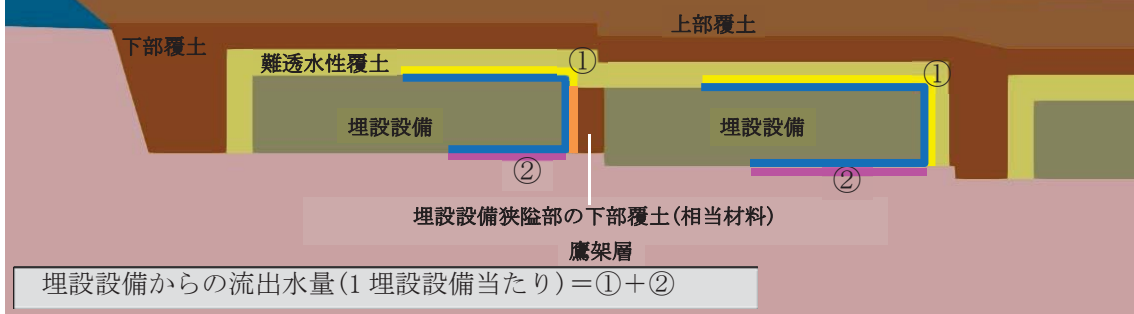
(a) 埋設設備狭隘部の下部覆土(相当材料)が劣化していないケース
