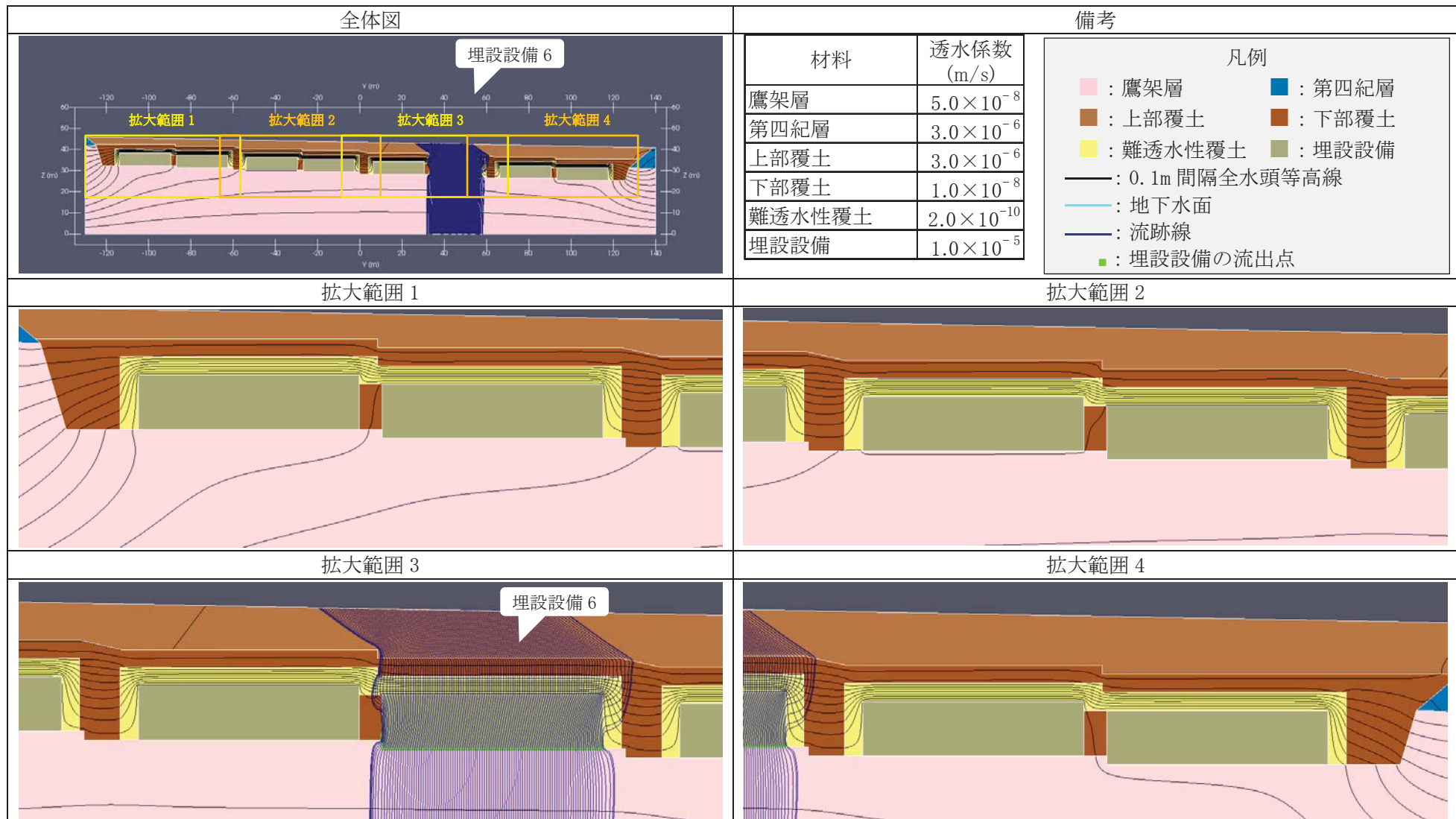
第 10 図 2 次元地下水浸透流解析結果【1 号廃棄物埋設地 鉛直下方】(確からしい設定 1,000 年後) (7/9) <埋設設備 6 の流出点を通る流跡線>
