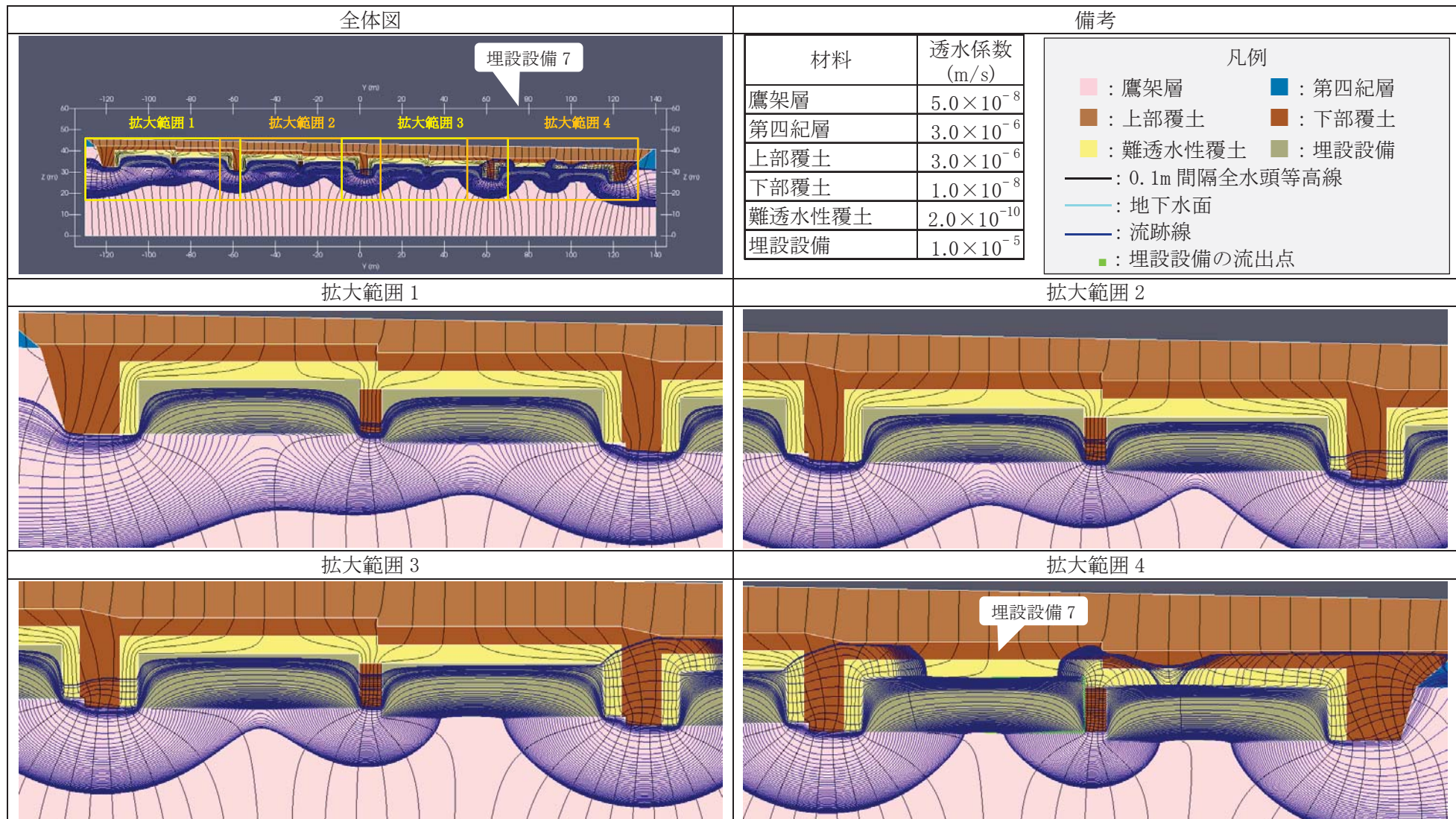
第9図 2次元地下水浸透流解析結果【1号廃棄物埋設地 水平方向】(確からしい設定 1,000年後) (8/9) <埋設設備7の流出点を通る流跡線>
