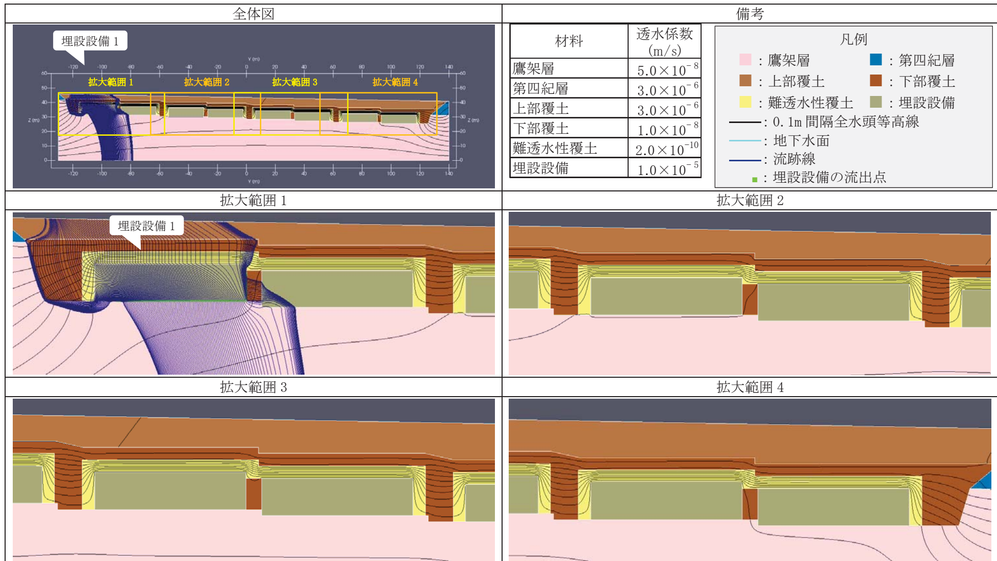
第 10 図 2 次元地下水浸透流解析結果【1 号廃棄物埋設地 鉛直下方】(確からしい設定 1,000 年後) (2/9) <埋設設備 1 の流出点を通る流跡線>
