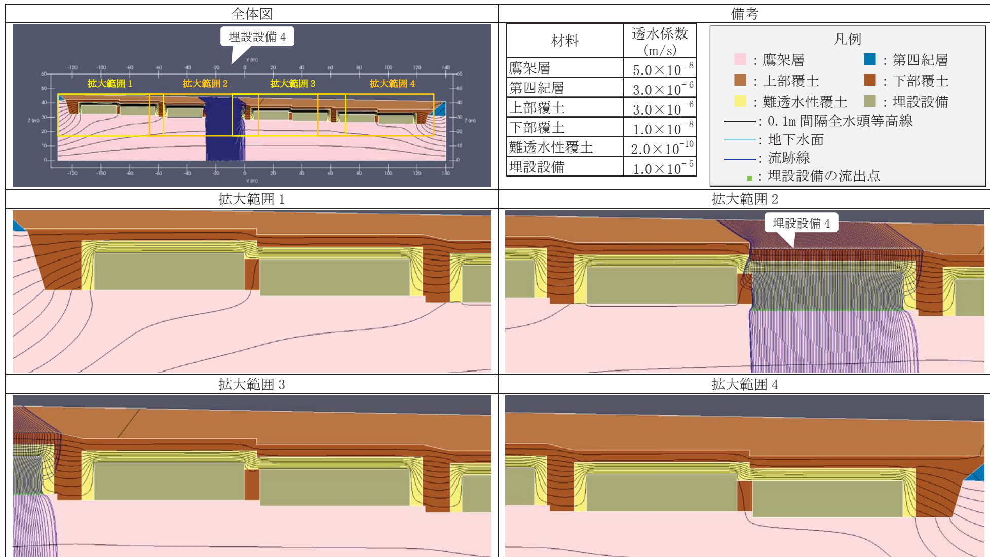
第 10 図 2次元地下水浸透流解析結果【1号廃棄物埋設地 鉛直下方】(確からしい設定 1,000 年後) (5/9) <埋設設備 4 の流出点を通る流跡線>
