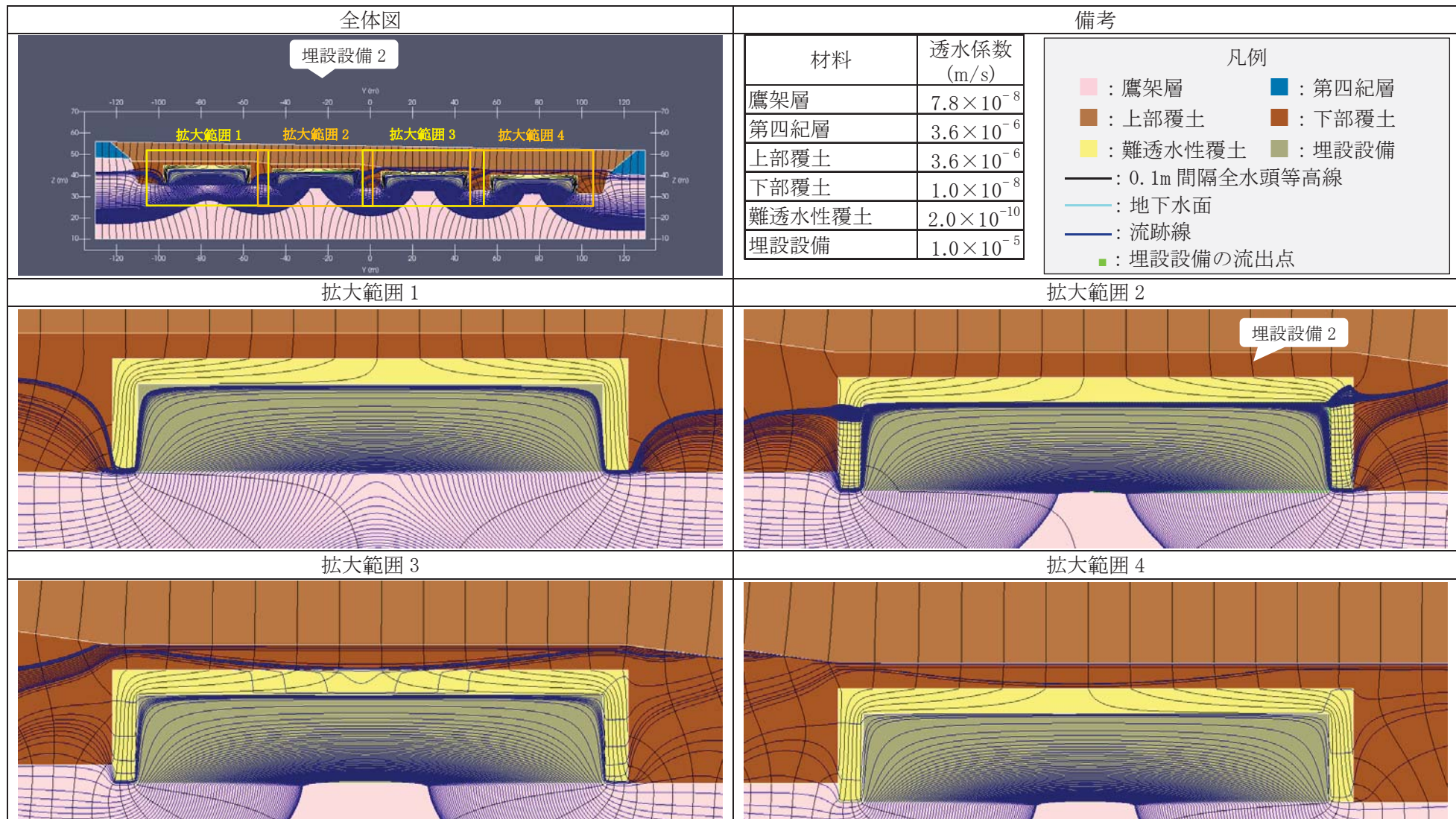
第 11 図 2 次元地下水浸透流解析結果【2号廃棄物埋設地 水平方向】(確からしい設定 1,000 年後) (3/5) <埋設設備 2 の流出点を通る流跡線>
