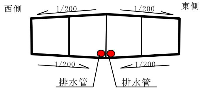
第 2 図 1 号集水構造断面図
