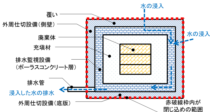
第12図 漏出防止機能の概念図
