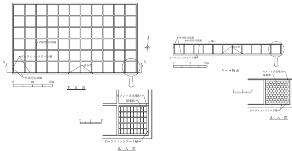
第 1 図 埋設設備平面図及び断面図
