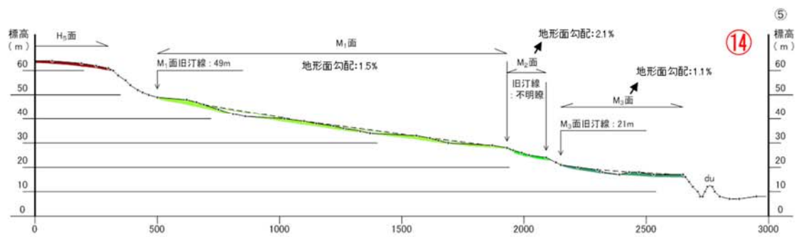
地形断面図(再処理審査会合(H28.12.26)資料1-3 p35再掲の一部抜粋加筆)
