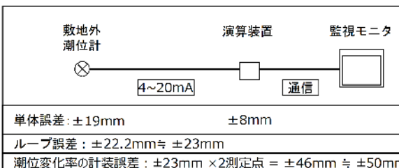
● 潮位計の誤差の考え方
