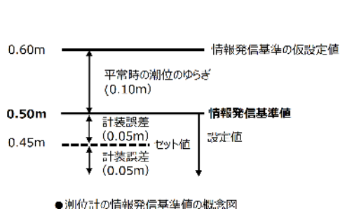
● 潮位計の情報発信基準値の概念図
