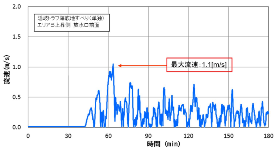
図-5 最大流速
