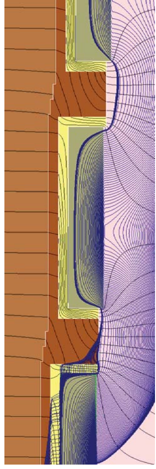
第1図 2次元地下水浸透解析結果【3号廃棄物埋設地】(確からしい設定 1,000年後) (3/5) <埋設設備 2の流出点を通る流跡線>
