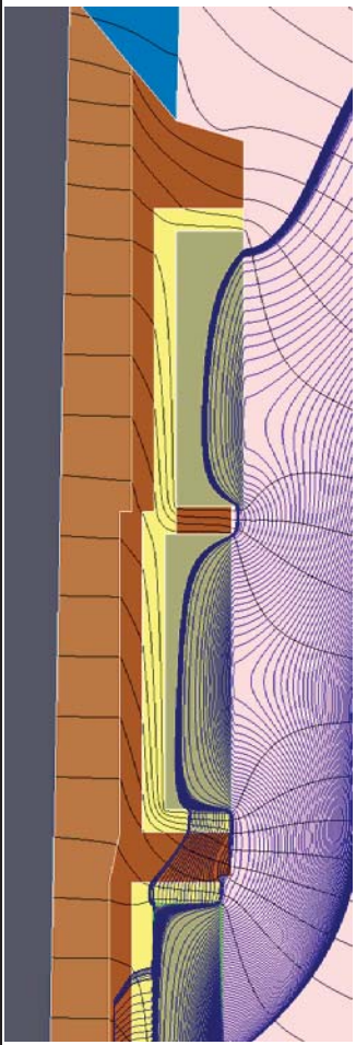
第 4 図 2 次元地下水浸透解析結果【1 号廃棄物埋設地】(厳しい設定 1,000 年後) (7/9) <埋設設備 6 の流出点を通る流跡線>
