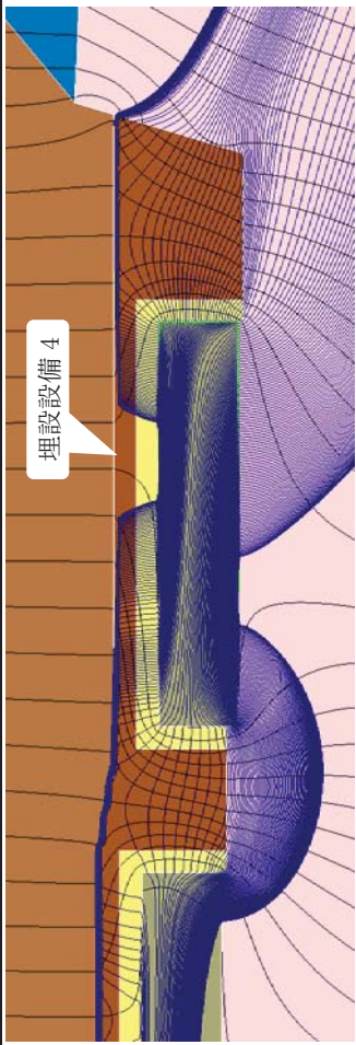
第2図 2次元地下水浸透解析結果【3号廃棄物埋設地】(厳しい設定 1,000年後) (5/5) <埋設設備 4の流出点を通る流跡線>
