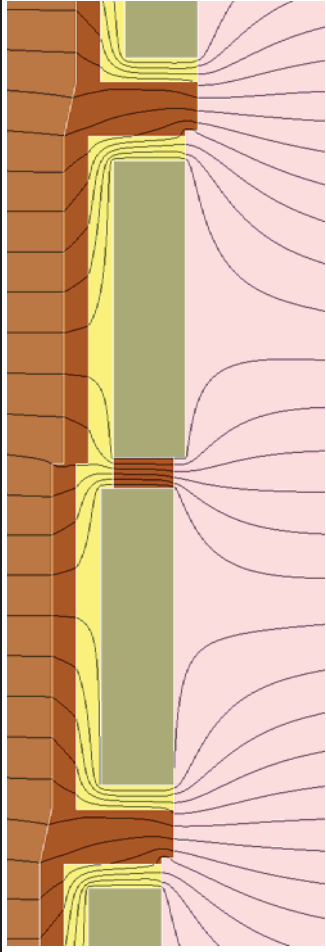
第9図 2次元地下水浸透流解析結果【1号廃棄物埋設地 水平方向】(確からしい設定 1,000年後) (1/9) <0.1m 間隔全水頭等高線>
