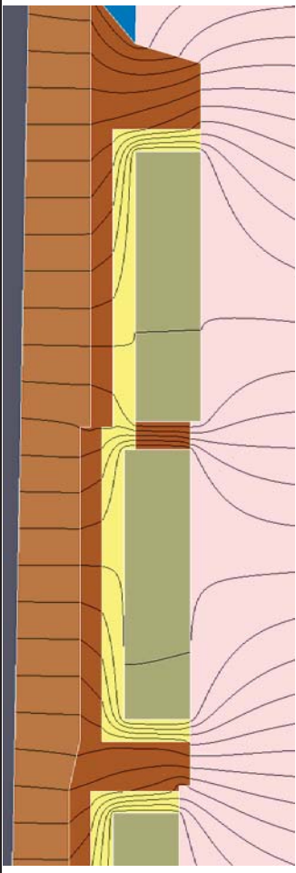
第9図 2次元地下水浸透流解析結果【1号廃棄物埋設地 水平方向】(確からしい設定 1,000年後) (1/9) <0.1m 間隔全水頭等高線>
