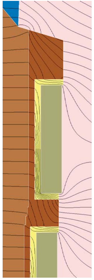
第 1 図 2 次元地下水浸透解析結果【3号廃棄物埋設地】(確からしい設定 1,000 年後) (1/5) <0.1m 間隔全水頭等高線>
