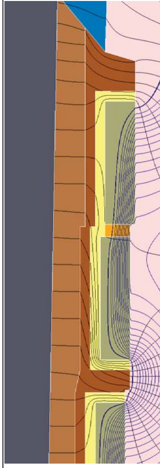
第 2 図 2 次元地下水浸透解析結果(厳しい設定 1,000 年後) (2/9) <埋設設備 1 の流出点を通る流跡線>
