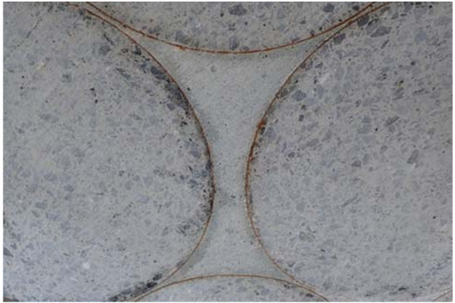
第 31 図 充填状況（輪切り断面）（その 1）
