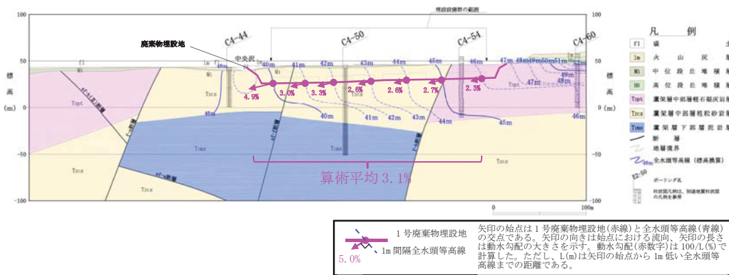
第10図 全水頭分布図(鉛直断面)(2/3)【1号廃棄物埋設地付近】
