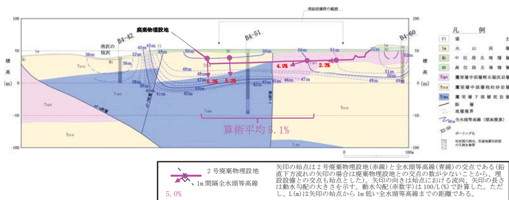
第10図 全水頭分布図(鉛直断面)(3/3)【2号廃棄物埋設地付近】
