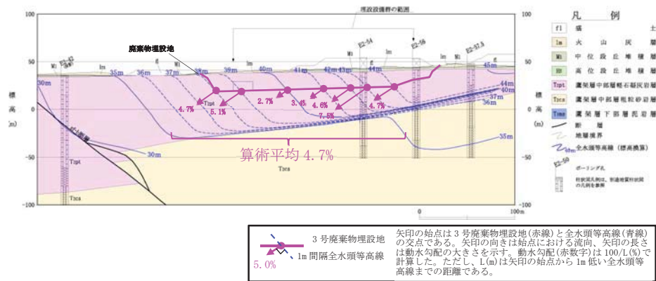
第10図 全水頭分布図(鉛直断面)(1/3)【3号廃棄物埋設地付近】
