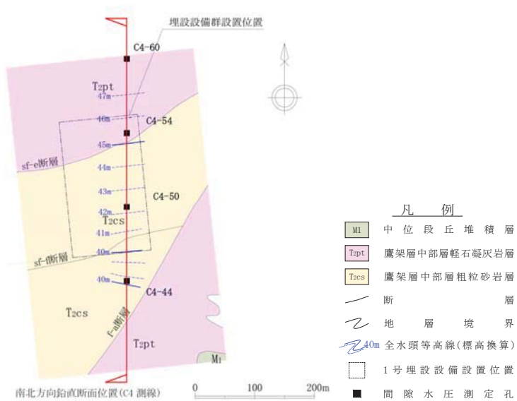
標高+30m 水平断面
