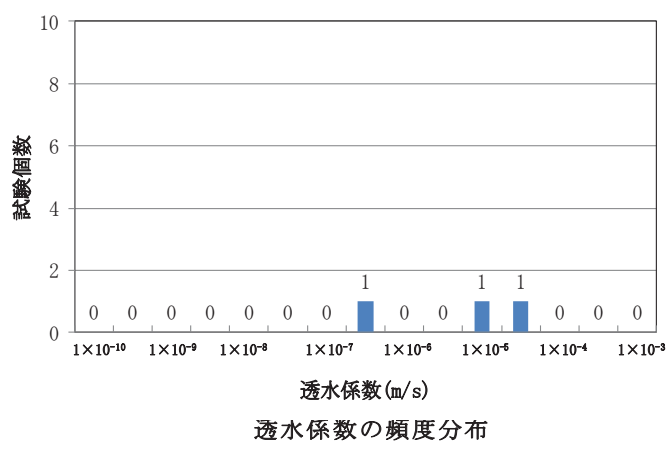
第 17 図 透水試験位置及び透水係数・試験標高頻度グラフ (2/11)
