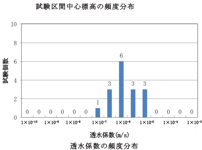
第 15 図 透水試験位置及び透水係数・試験標高頻度グラフ (2/12) 【第四紀層(火山灰層、段丘堆積層)】
