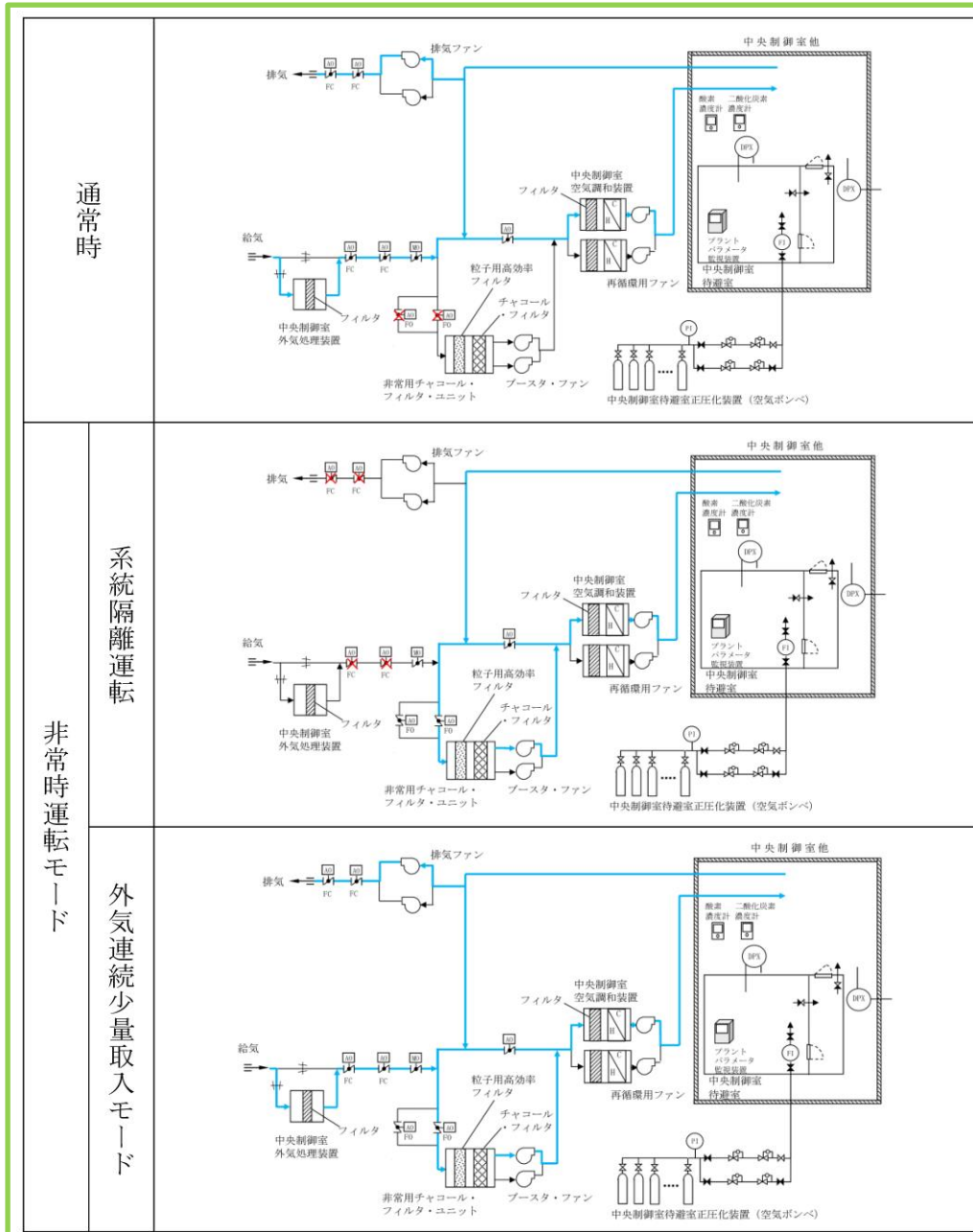
図 2.4-17 運転モード毎の中央制御室換気系 系統概要図（1／2）
