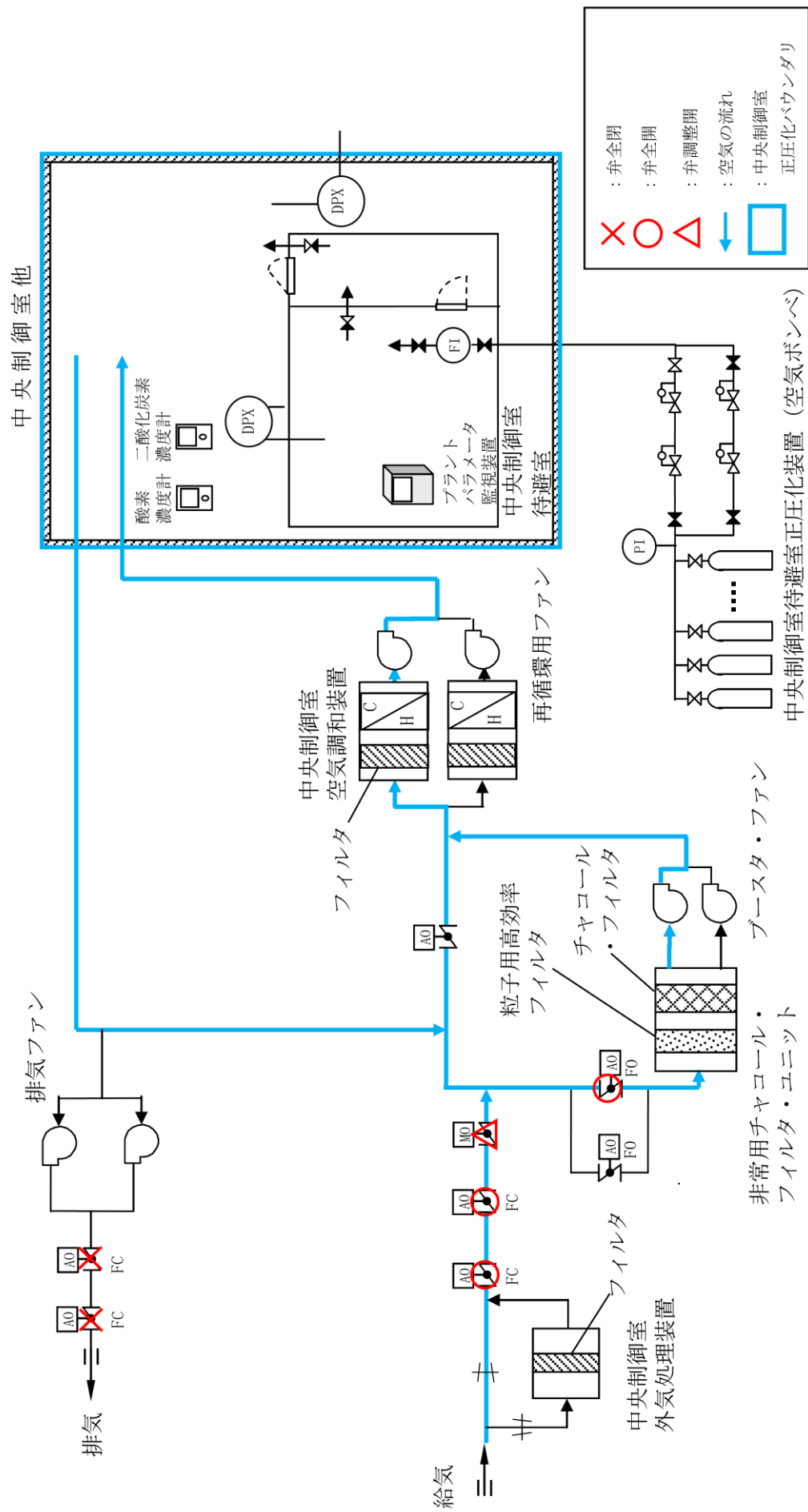
図 59-4-4 中央制御室換気系及び中央制御室待避室正圧化装置 (空気ポンベ) 概略系統図 (非常時運転モード (加圧運転 (プルーム通過前及びプルーム通過後)))
