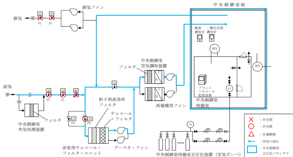
図 2.4-4 中央制御室換気系及び中央制御室待避室正圧化装置系統概要図（炉心の著しい損傷の発生時、プルーム通過前及びプルーム通過後）
