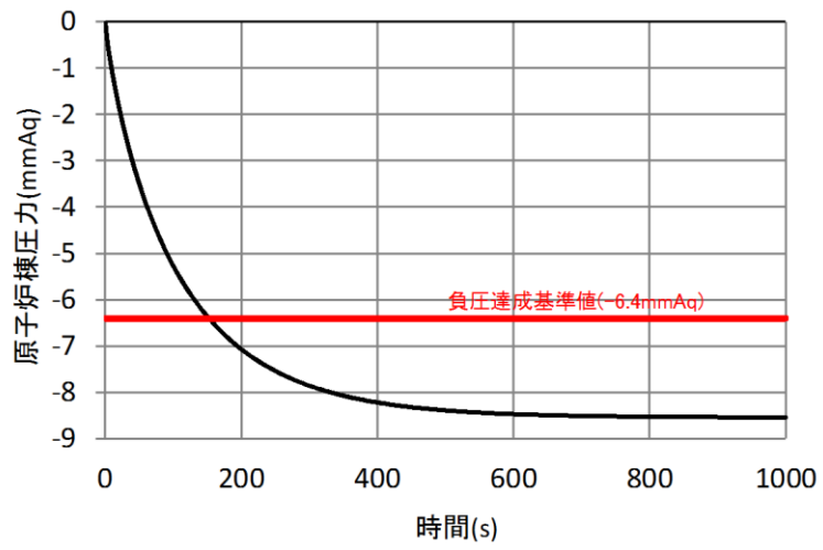
図 2 原子炉棟圧力の時間変化
