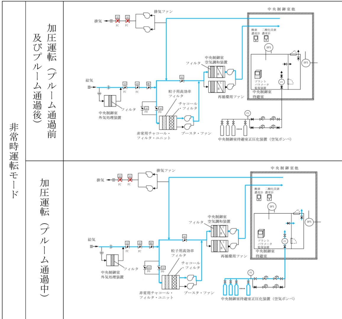
図 2.4-17 運転モード毎の中央制御室換気系 系統概要図 (2/2)
